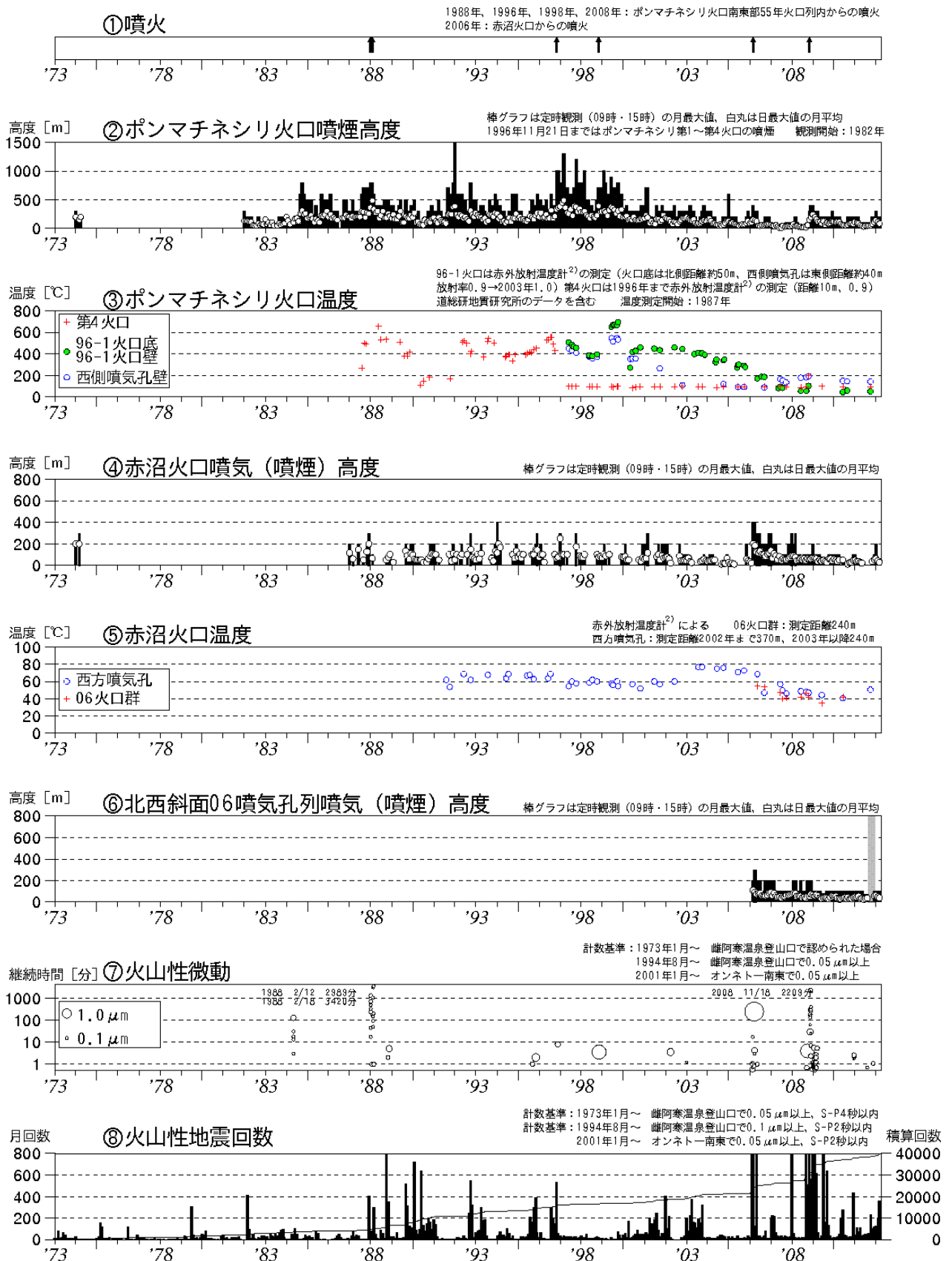
図 1 ※ 雌阿寒岳 火山活動経過図（1973年 1 月～2012年 3 月）
