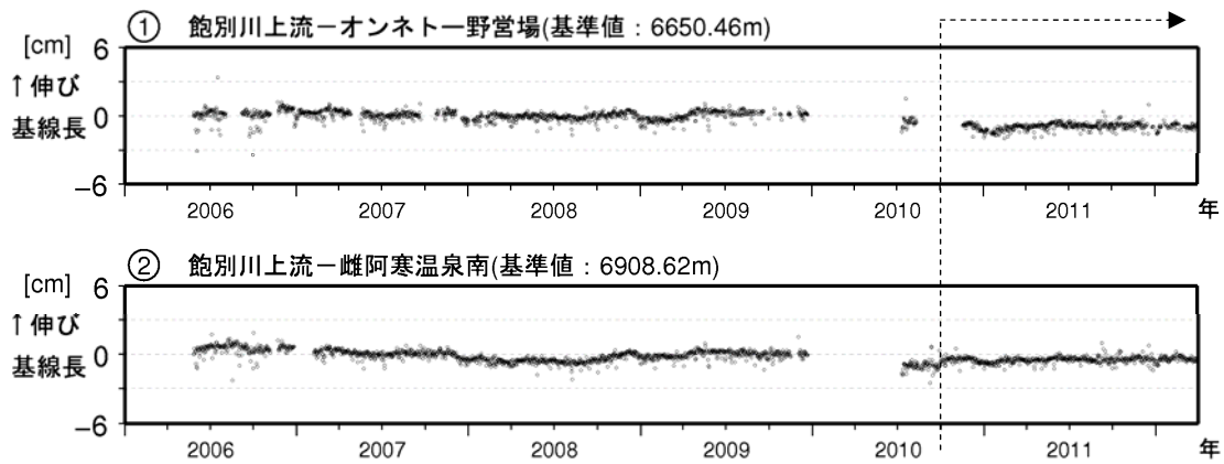
図 5 雌阿寒岳 GPS連続観測による基線長変化（2006年 1 月～2012年 3 月） ・グラフの空白部分は欠測 GPS基線①～②は図 6 の①～②に対応 ・2010年10月以降のデータについては、電離層の影響を補正する等、解析方法を改良しています
