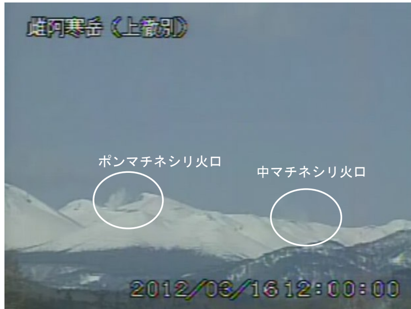
図2 雌阿寒岳 山体南側の状況（3月16日、 かみてしべつ 上徹別遠望カメラによる） 白丸内はポンマチネシリ火口の噴煙及び中マチネシリ火口の噴気
