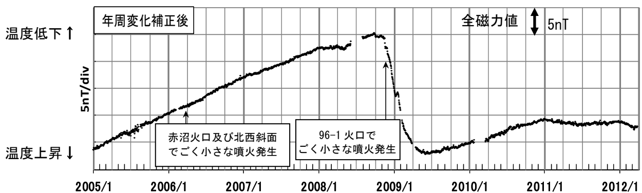
図3 雌阿寒岳 全磁力連続観測 1) による連続観測点MEA（上図中◎）の全磁力値変化 （2005年1月1日～2012年3月26日）※グラフの空白部分は欠測
