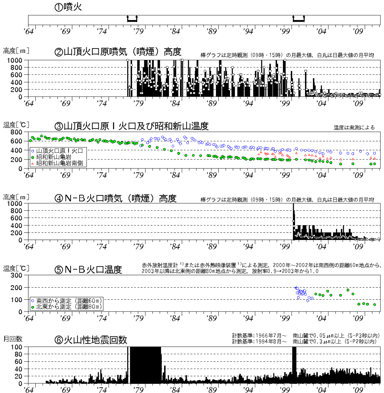
図 1※ 有珠山 火山活動経過図（1964年 1 月～2012年 2 月）
