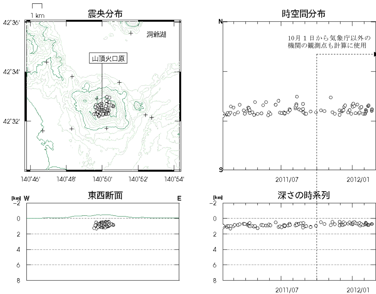
図3※ 有珠山 火山性地震の震源分布 (2011年2月～2012年2月)
