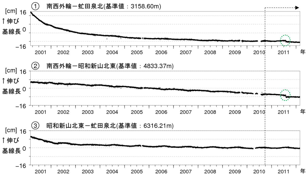
図 4 有珠山 GPS連続観測による基線長変化 (2001年3月~2012年2月)
