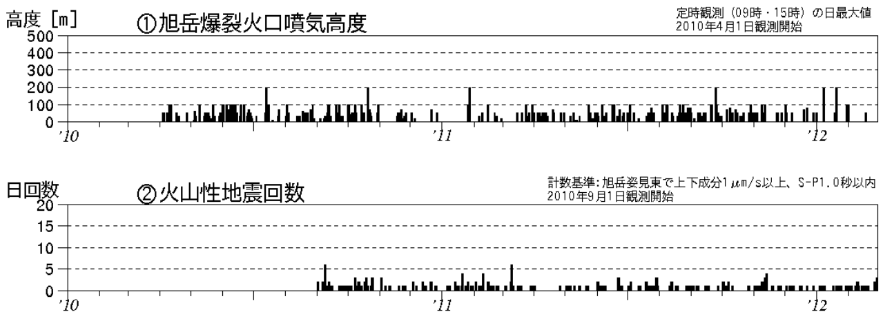
図1 大雪山 火山活動経過図（2010年4月～2012年2月）
