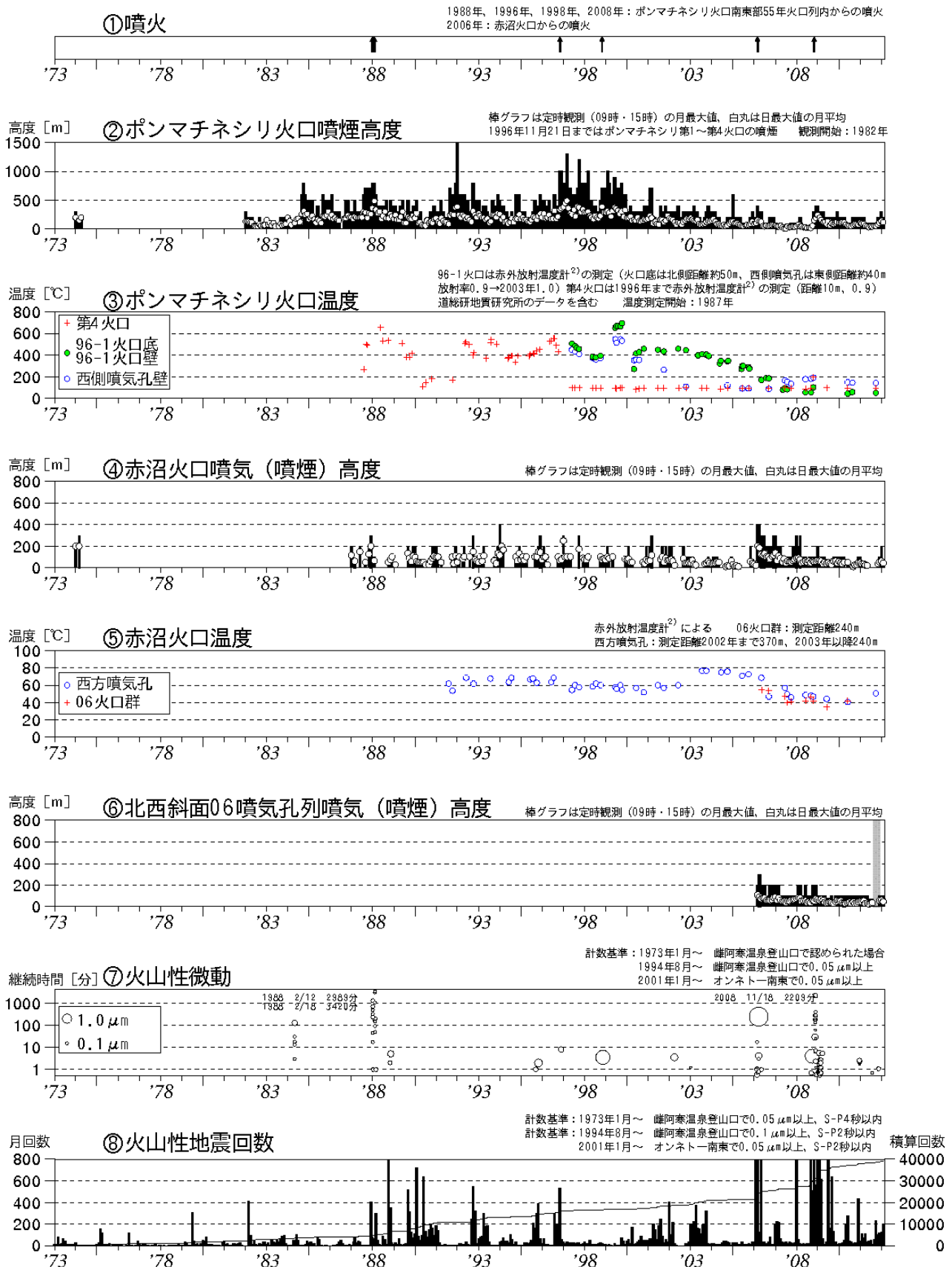
図 1 ※ 雌阿寒岳 火山活動経過図（1973年 1 月～2012年 2 月）
