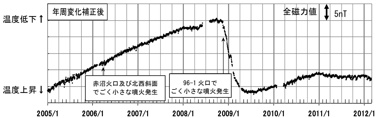
図 3 雌阿寒岳 全磁力連続観測 1) による連続観測点MEA（上図中◎）の全磁力値変化 （2005年1月1日～2012年2月26日）※グラフの空白部分は欠測
