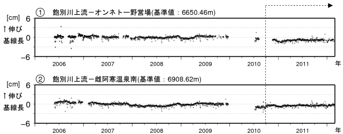
図 5 雌阿寒岳 GPS連続観測による基線長変化（2006年 1 月～2012年 2 月） ・グラフの空白部分は欠測 GPS基線①～②は図 6 の①～②に対応 ・2010年10月以降のデータについては、電離層の影響を補正する等、解析方法を改良しています
