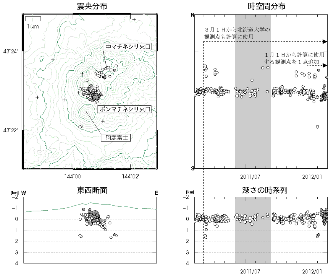
図 4 ※ 雌阿寒岳 火山性地震の震源分布 (2011年 2 月～2012年 2 月) 灰色の期間は一部観測点欠測のため震源の決定数減少や精度低下が見られます ○印：2011年 2 月～2012年 1 月の震源 ●印：2012年 2 月の震源 +印：地震観測点
