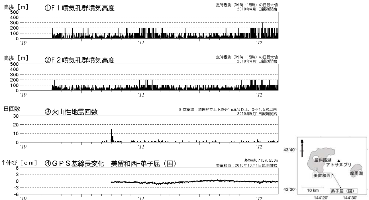
図1※ アトサヌプリ 火山活動経過図（2010年4月～2012年2月）、GPS連続観測点配置図
