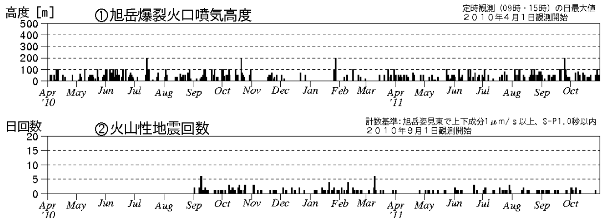
図 1 大雪山 火山活動経過図（2010 年 4 月～2011 年 10 月）
