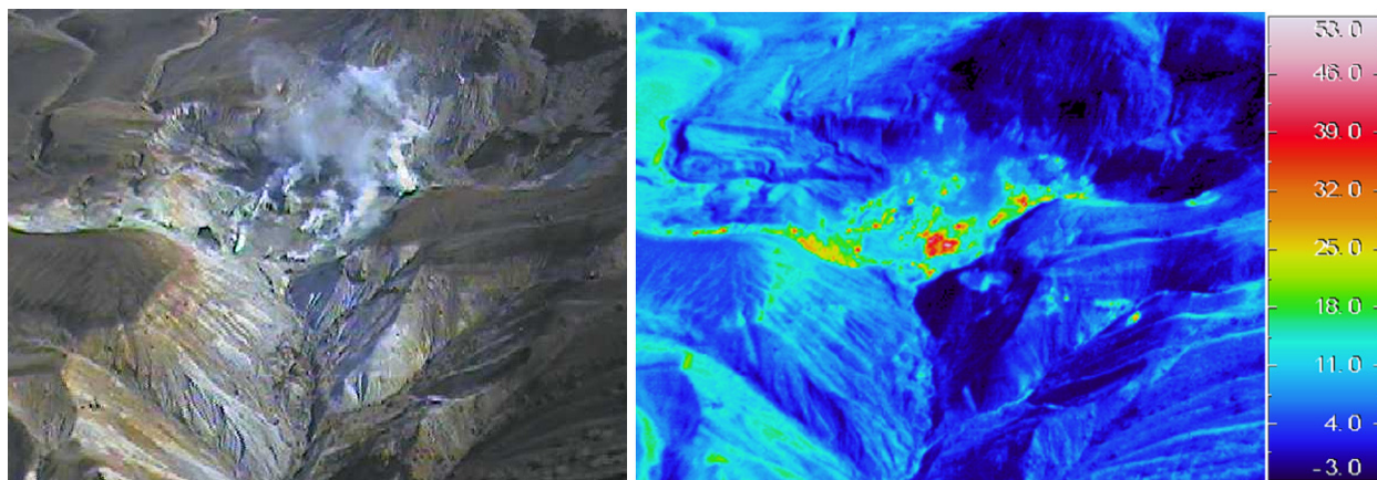
図 7 雌阿寒岳 中マチネシリ火口の地表面温度分布（図 4-③から撮影）
