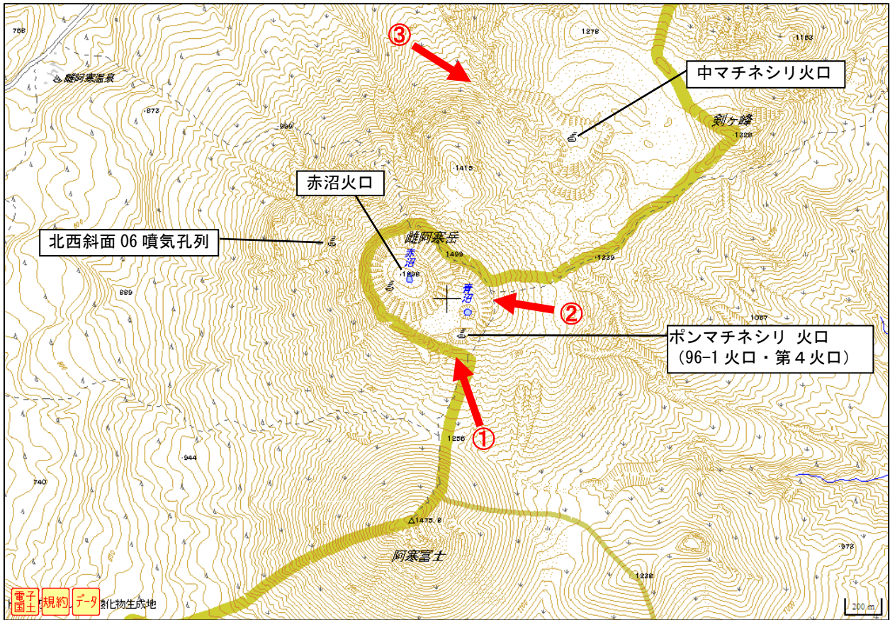
図 4 雌阿寒岳 火口位置図と赤外熱映像及び写真の撮影方向
