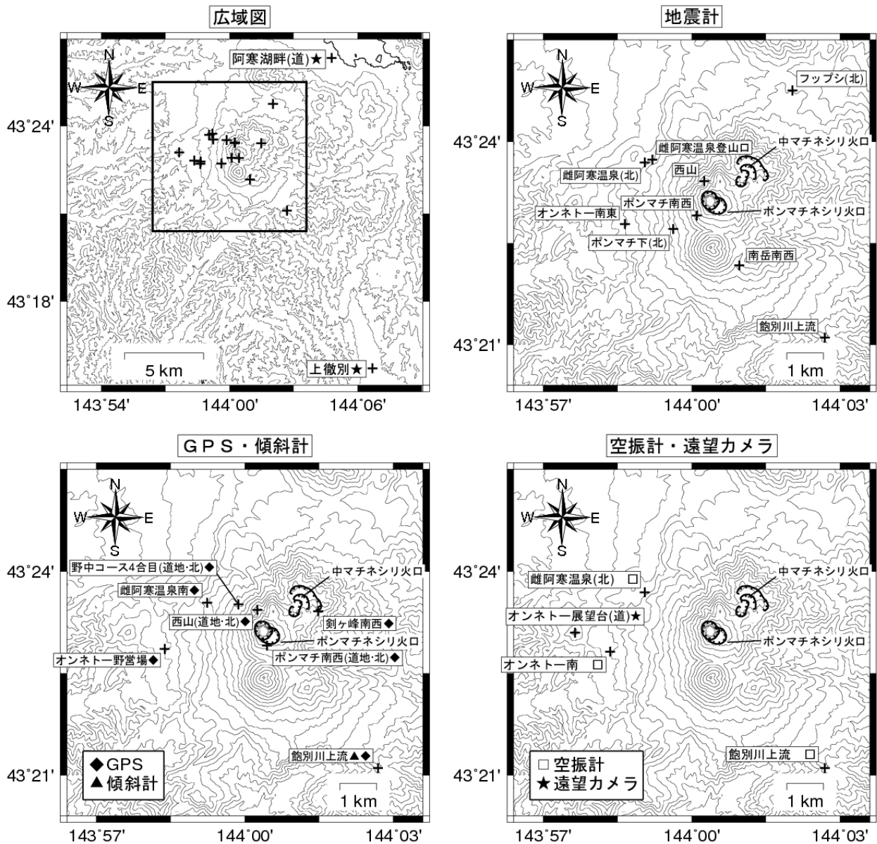
図11 雌阿寒岳 観測点配置図 +は観測点の位置を示す 他機関の観測点には以下の記号を付している (北) : 北海道大学 (道地) : 道総研地質研究所 (道) : 北海道
