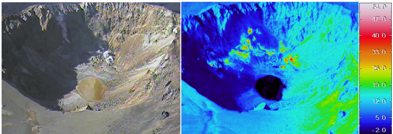
図 6 雌阿寒岳 赤沼火口の地表面温度分布（図 4-②から撮影）
