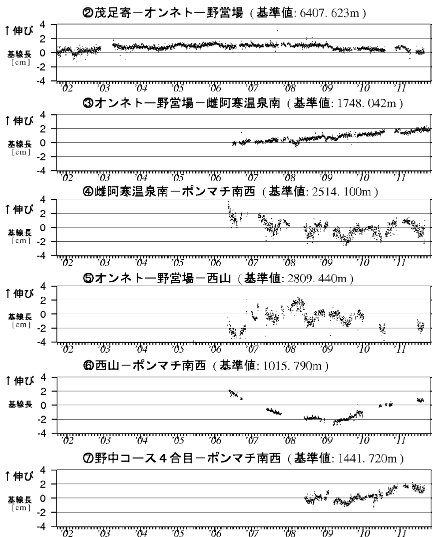
図 9※ 雌阿寒岳 GPS 連続観測による基線長変化 (2001 年 10 月～2011 年 10 月) グラフの空白部分は欠測 GPS 基線②～⑦は図 10 の②～⑦に対応
