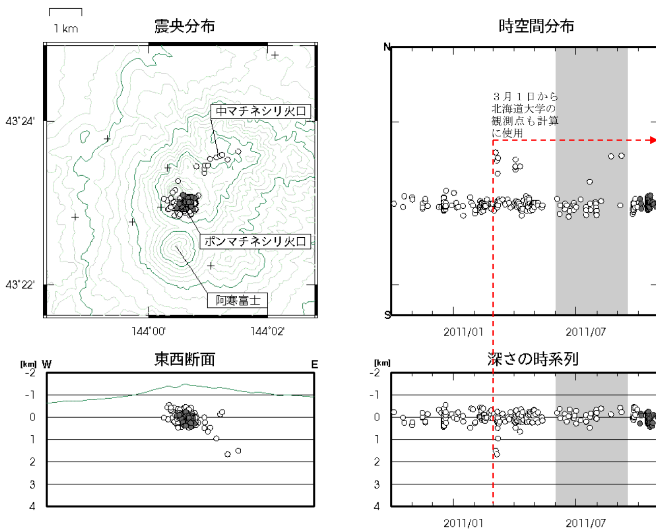
図 8 ※ 雌阿寒岳 火山性地震の震源分布 (2010 年 10～2011 年 10 月) 表示期間中、灰色の期間は一部観測点欠測のため震源の決定数減少や精度低下が見られます。 ○印：2010 年 10 月～2011 年 9 月の震源 ●印：2011 年 10 月の震源 +印：地震観測点
