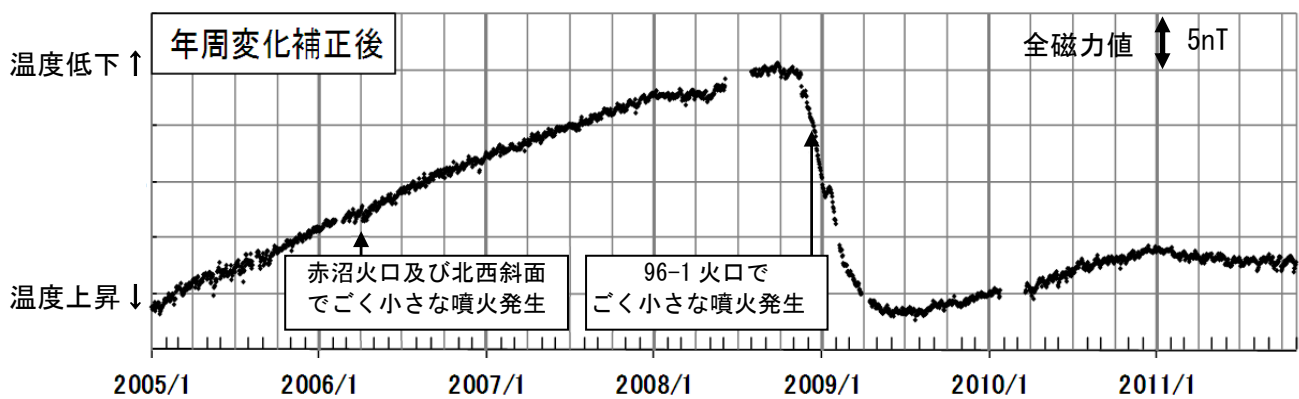
図3 雌阿寒岳 全磁力連続観測 1) による連続観測点 MEA（上図中◎）の全磁力値変化 （2005年1月1日～2011年10月30日）※グラフの空白部分は欠測
