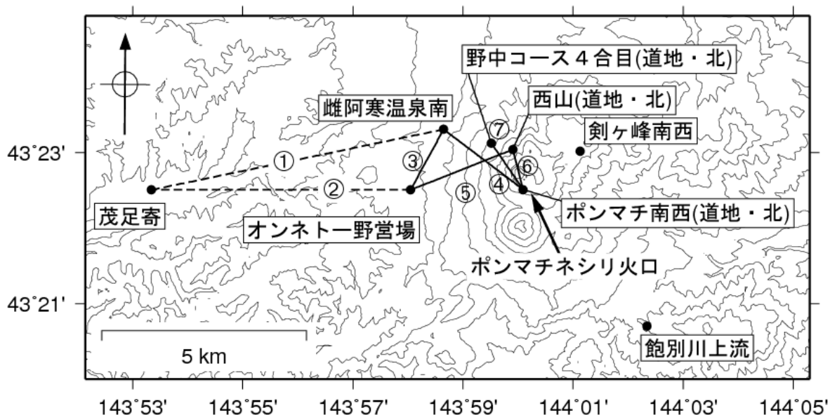
図 10※ 雌阿寒岳 GPS 連続観測点配置図
