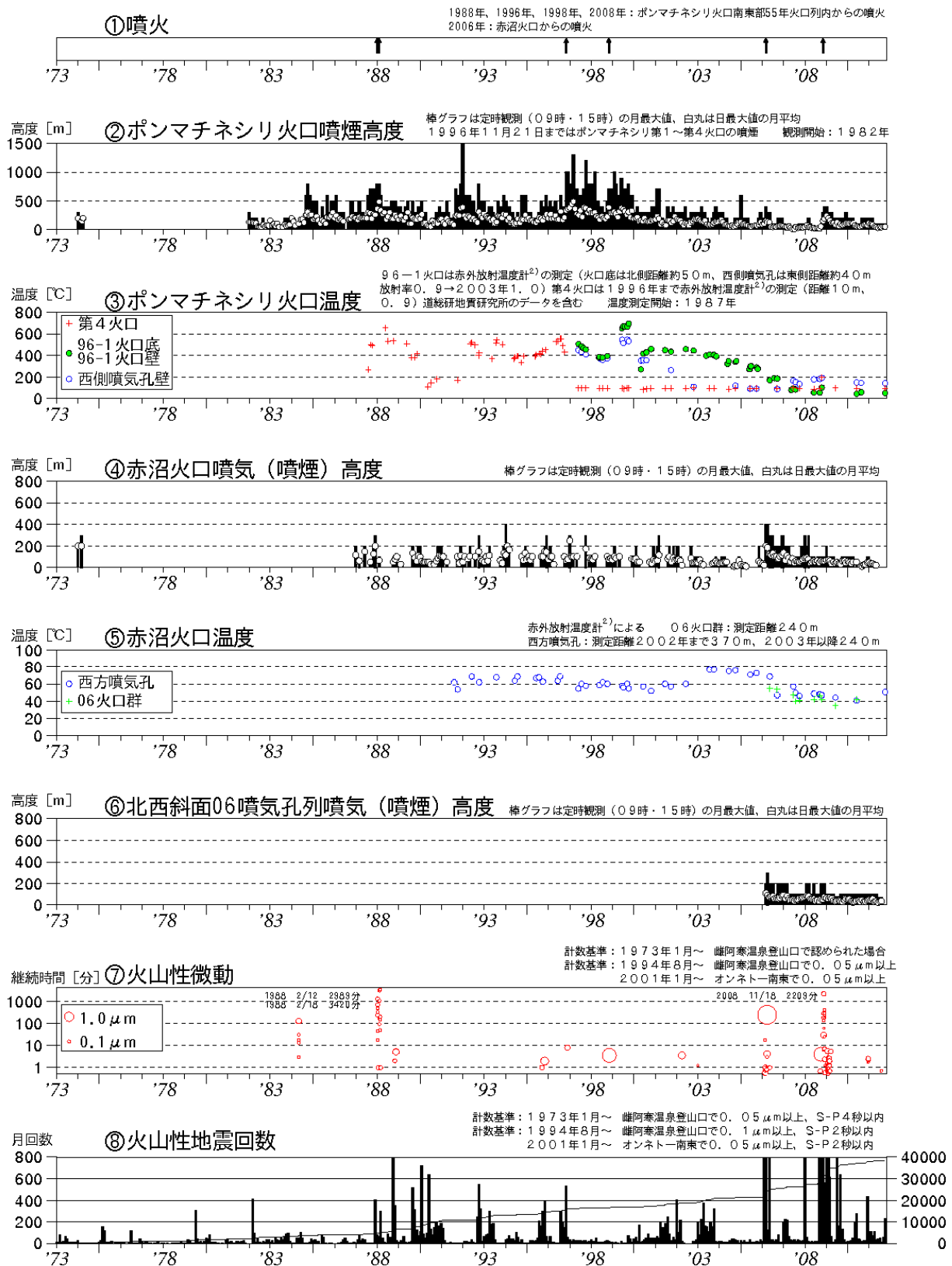
図 1※ 雌阿寒岳 火山活動経過図（1973 年 1 月～2011 年 10 月）
