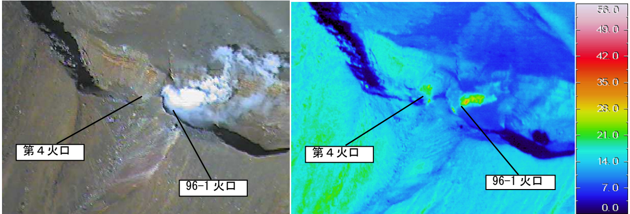
図 5 雌阿寒岳 ポンマチネシリ火口（96-1 火口・第 4 火口）の地表面温度分布（図 4-①から撮影）
