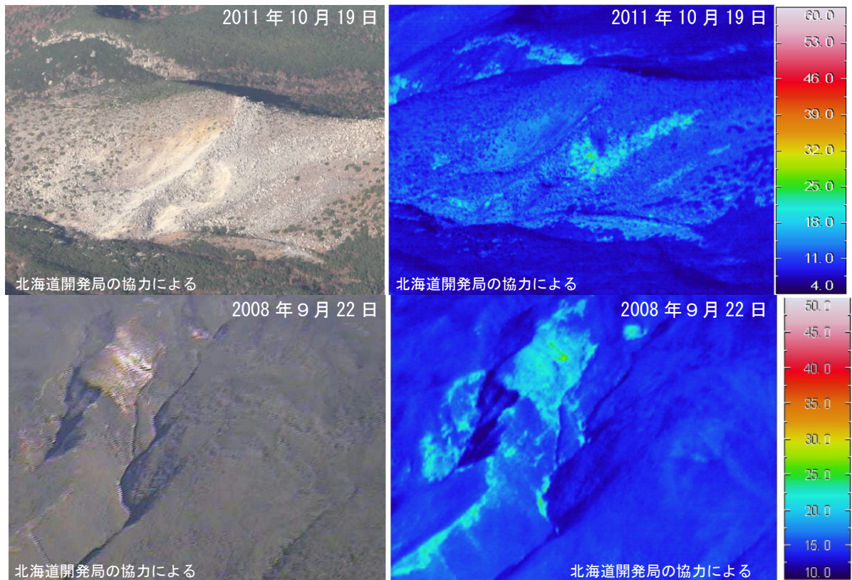
図 3 知床硫黄山 北西側中腹の爆裂火口の地表面温度分布 （上段は今回：図 1-③から撮影、下段は前回：図 1-④から撮影）
