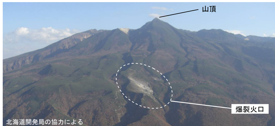
図 2 知床硫黄山 全景（図 1-①から撮影）
