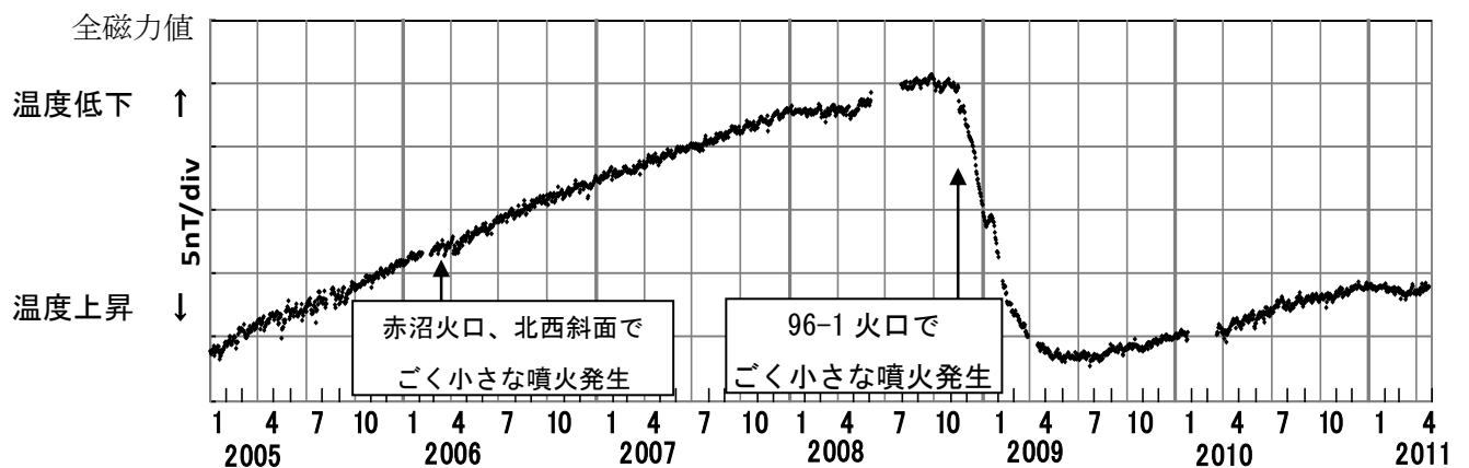
図4 雌阿寒岳 全磁力連続観測結果（2005年1月1日～2011年4月25日） MEAと地磁気観測所女満別出張所の全磁力単純差（日平均値、年周変化補正） 図3のMEA（◎）にて測定 図の空白は欠測
