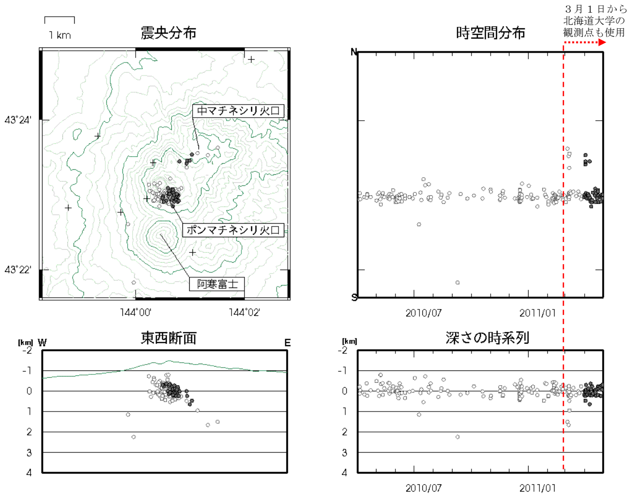
図 5 ※ 雌阿寒岳 火山性地震の震源分布 (2010 年 4 月～2011 年 4 月)
