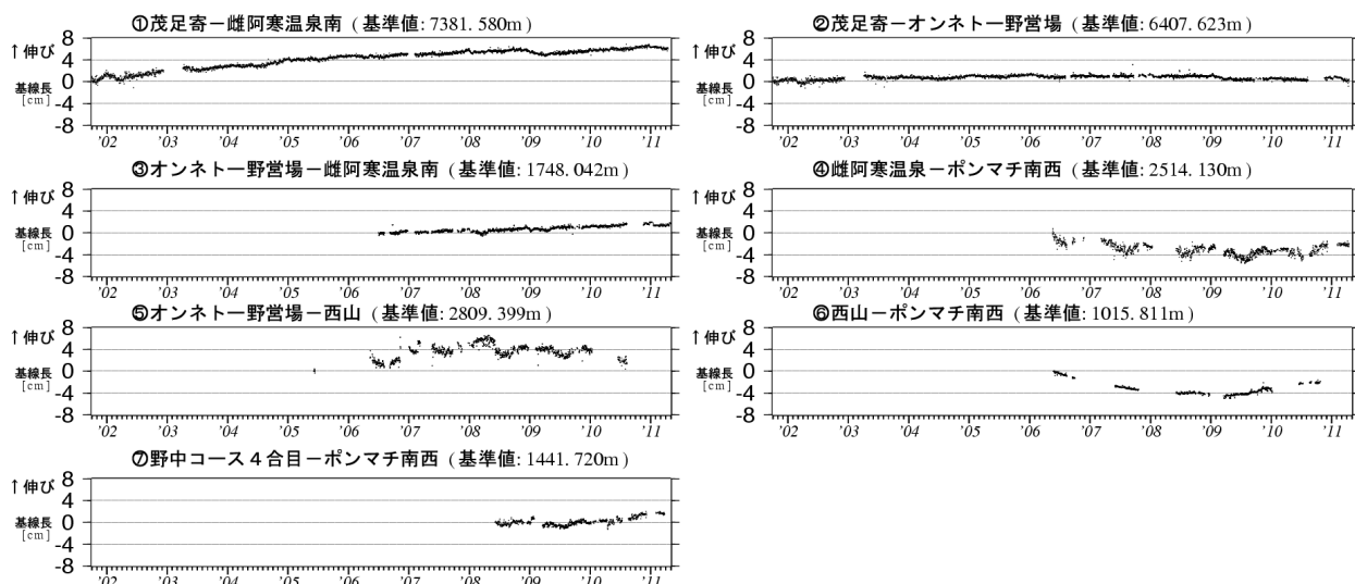
図 6※ 雌阿寒岳 GPS 連続観測による基線長変化（2001 年 10 月～2011 年 4 月） グラフの空白部分は欠測。 GPS 基線①～⑦は図 7 の①～⑦に対応しています。
