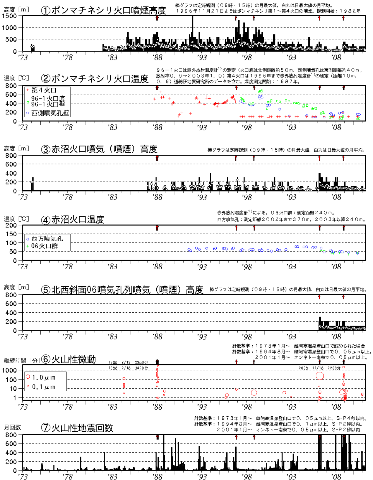
図1※ 雌阿寒岳 長期の火山活動経過図（1973年1月～2011年4月） ↑印は噴火 （1988年、1996年、1998年、2008年：ポンマチネシリ火口南東側からの噴火、2006年：赤沼火口からの噴火）
