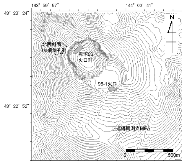
図3 雌阿寒岳 全磁力連続観測点位置図（図中 MEA◎）
