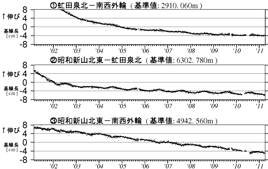
図 4 有珠山 GPS 連続観測による基線長変化（2001 年 3 月～2011 年 3 月） グラフの空白部分は欠測
