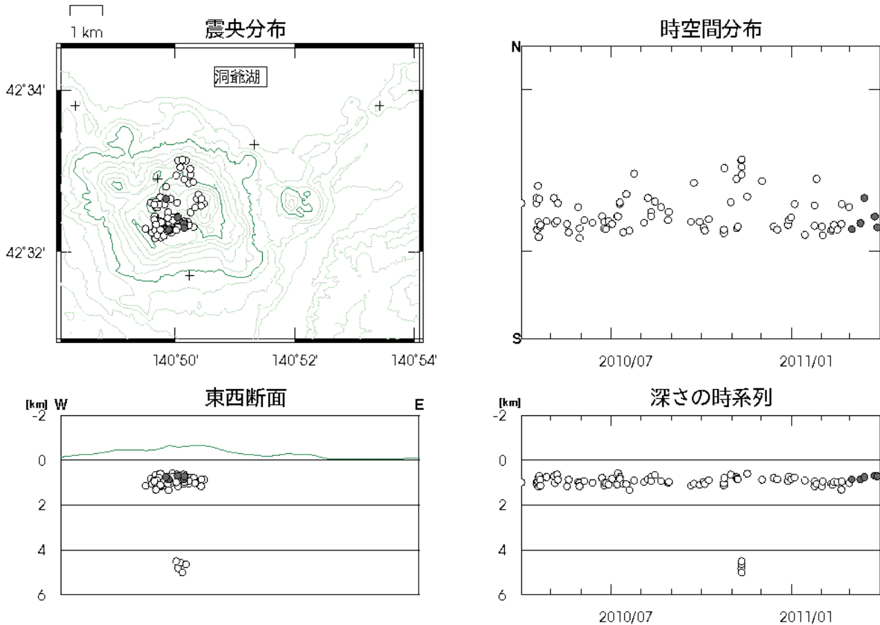
図 3 有珠山 震源分布図（2010 年 4 月～2011 年 3 月、+は地震観測点）
