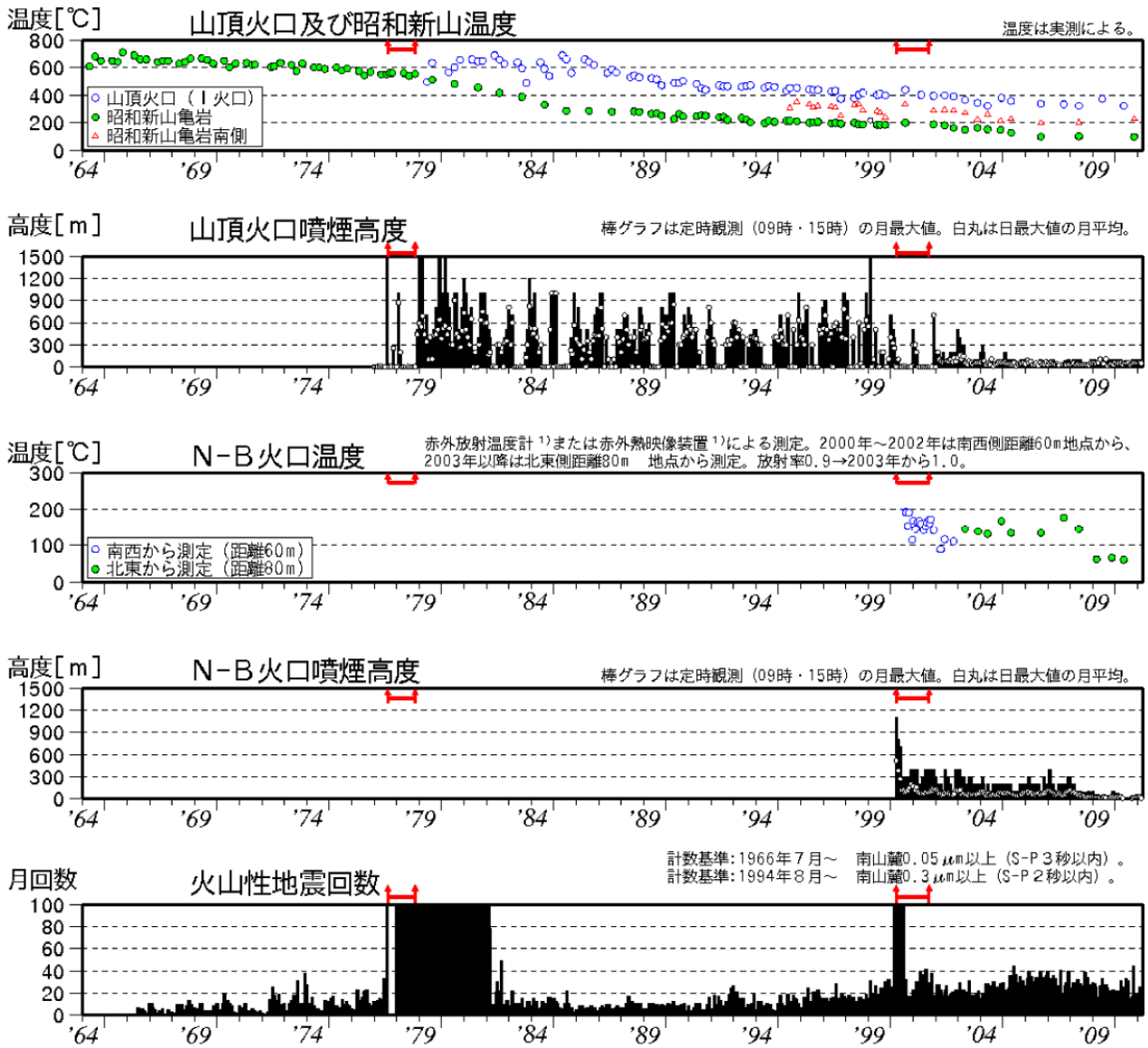
図 1 有珠山 長期の火山活動経過図（1964 年 1 月～2011 年 3 月）
