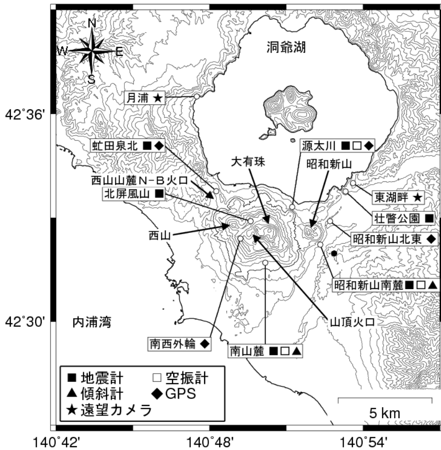
図 7 有珠山 観測点配置図
