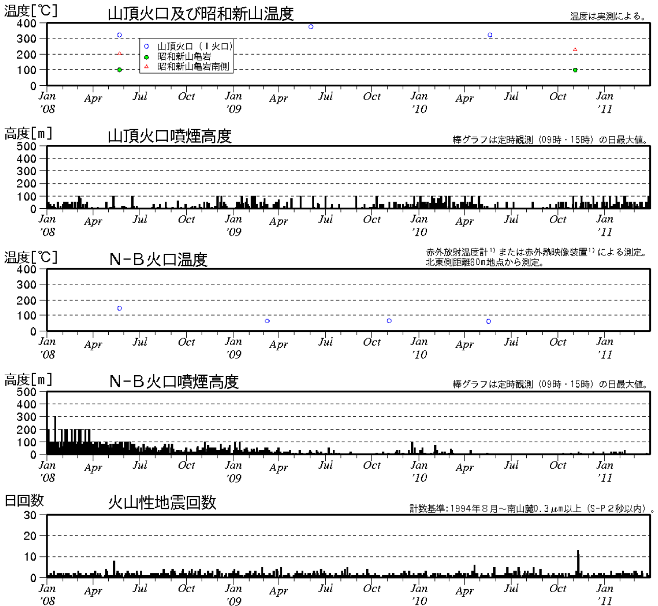
図 2 有珠山 最近の火山活動経過図（2008 年 1 月～2011 年 3 月）
