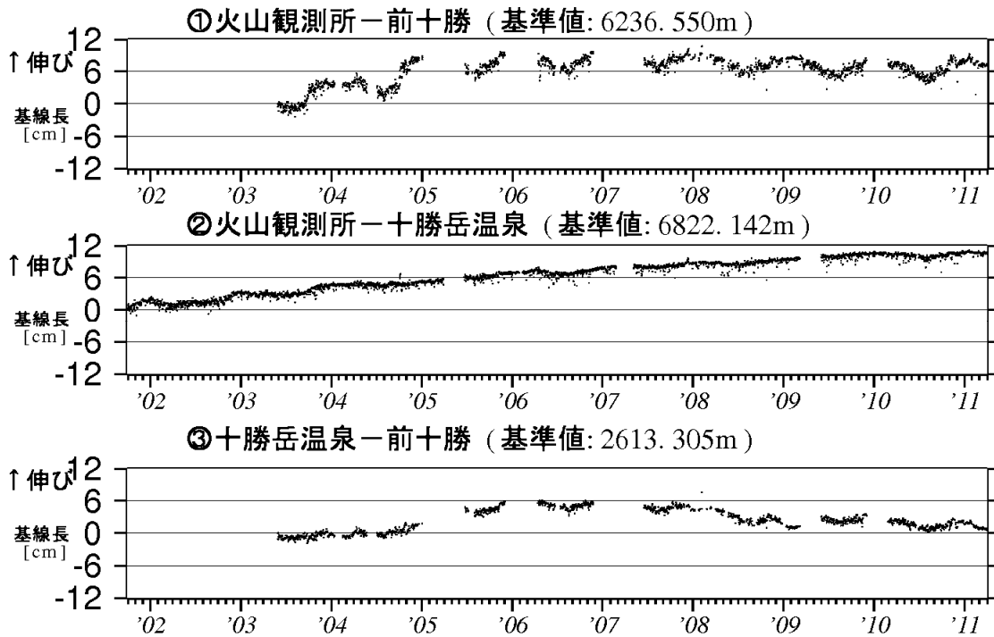
図4※ 十勝岳 GPS 連続観測による基線長変化 (2001 年 10 月～2011 年 3 月)
