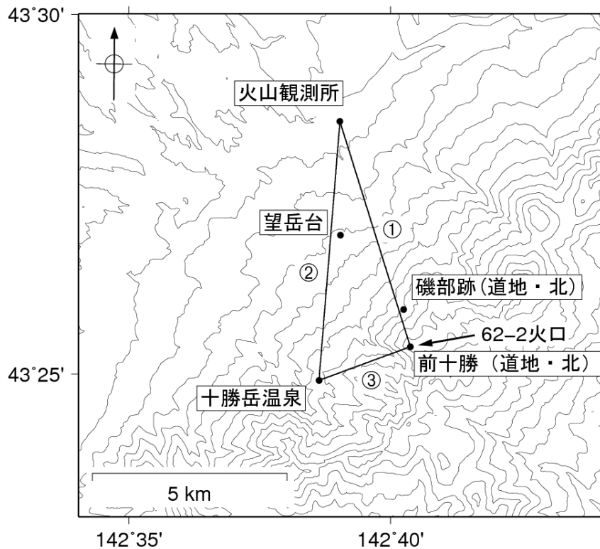
図5※ 十勝岳 GPS 観測点配置図
