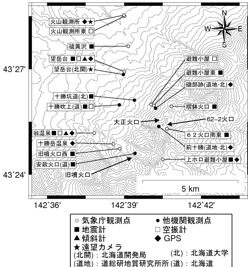
図7 十勝岳 観測点配置図
