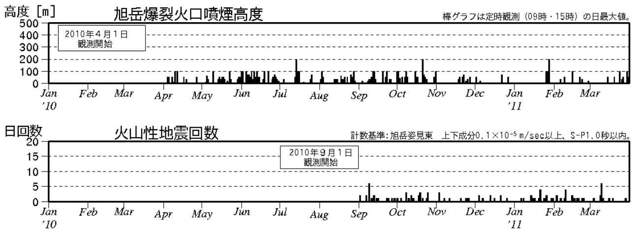
図 1 大雪山 最近の火山活動経過図（2010 年 4 月～2011 年 3 月）
