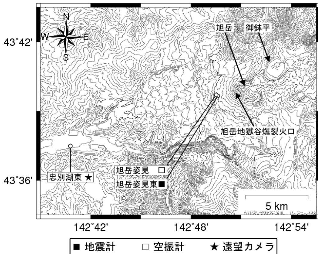
図3 大雪山 観測点配置図
