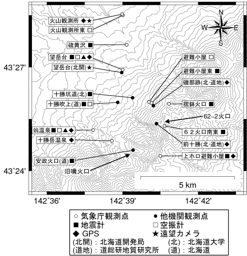
図 11 十勝岳 観測点配置図
