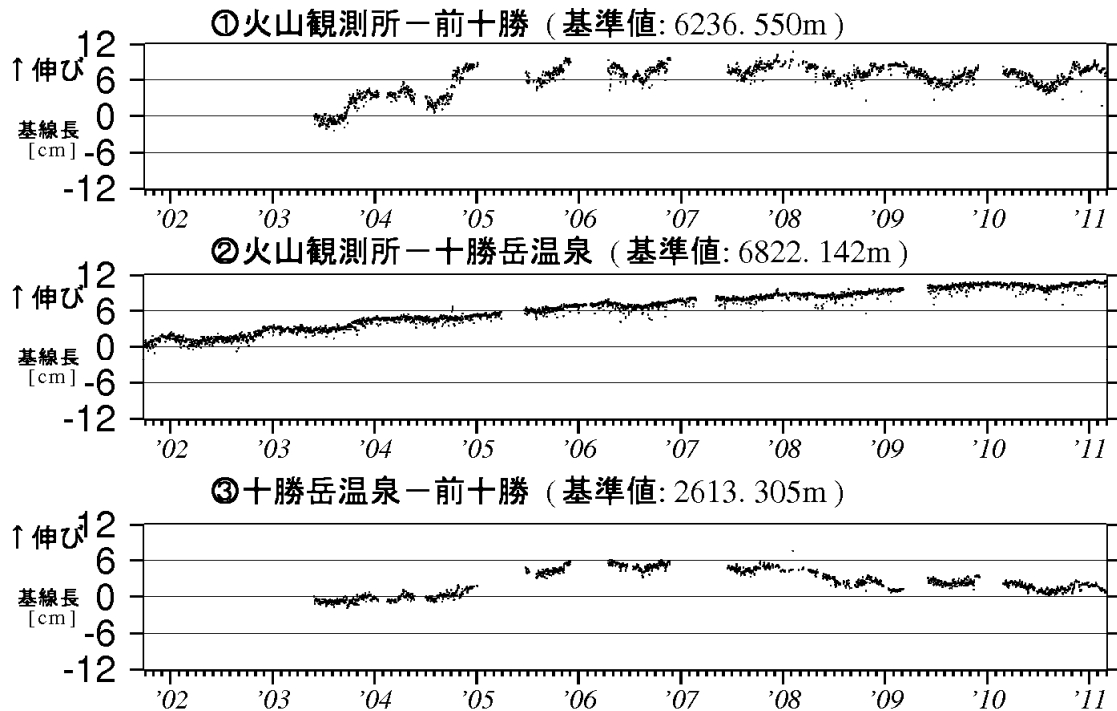
図 8※ 十勝岳 GPS 連続観測による基線長変化（2001 年 10 月～2011 年 2 月）
