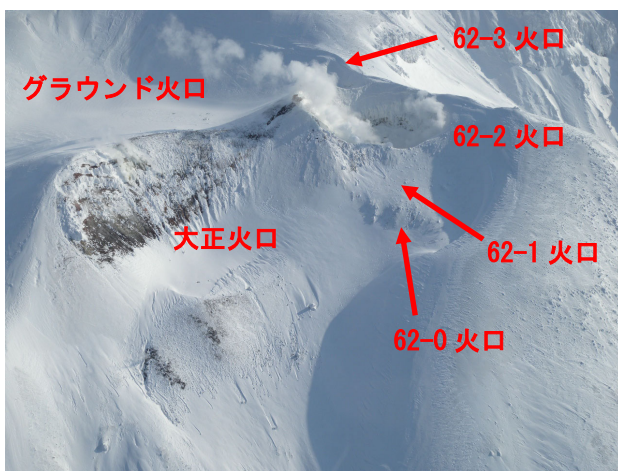
図 4 十勝岳 北西側上空（図 3 の①）から見た 62 火口群及び大正火口の状況
