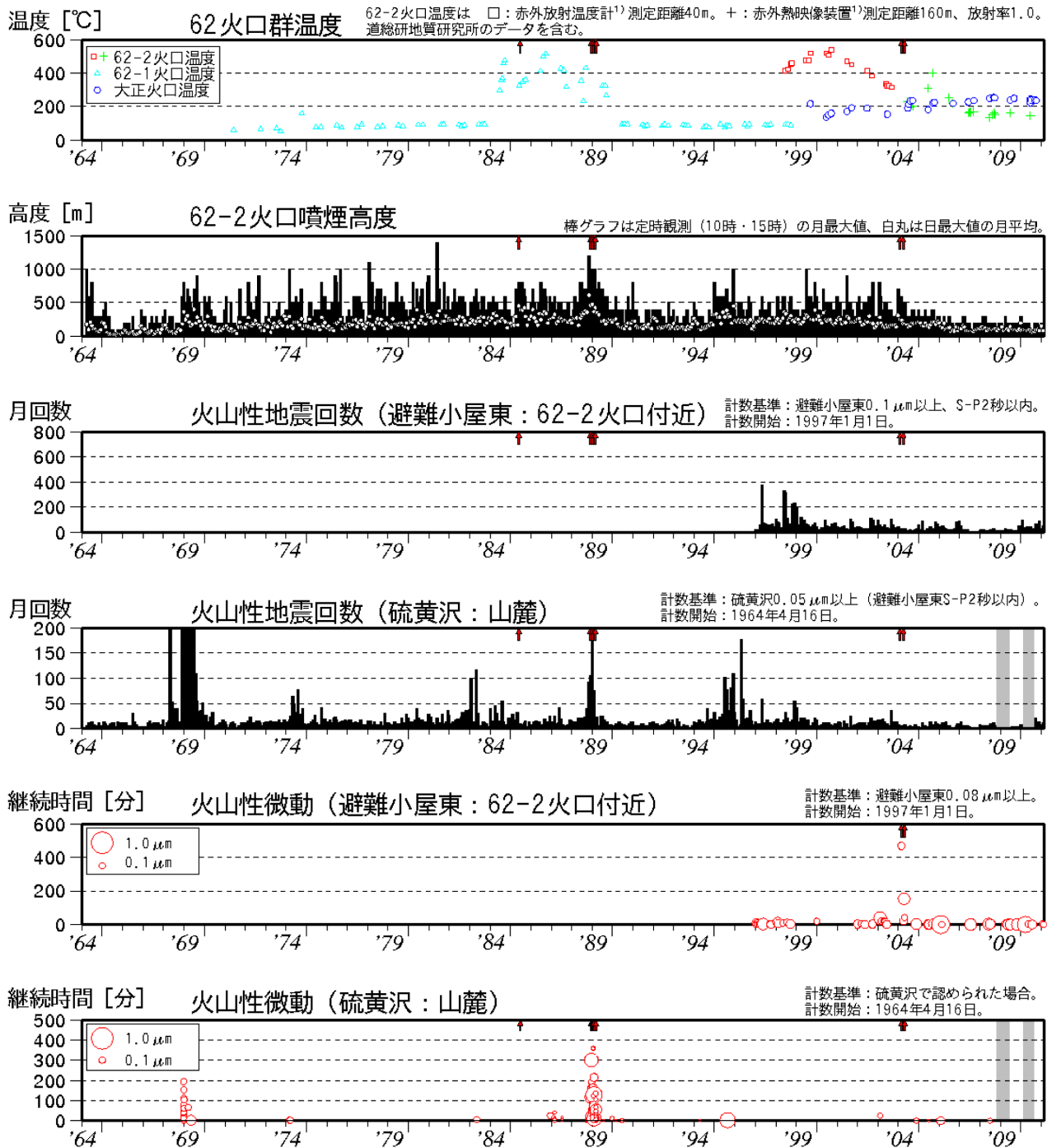
図 1 ※ 十勝岳 長期の火山活動経過図（1964 年 1 月～2011 年 2 月）
