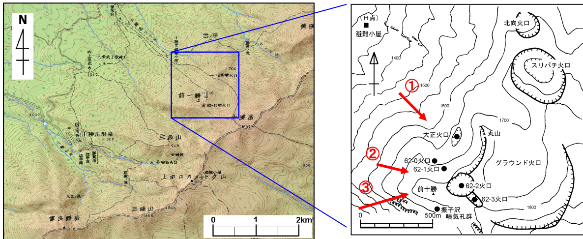
図 3 十勝岳 火口周辺図（矢印は写真及び赤外熱映像撮影方向）
