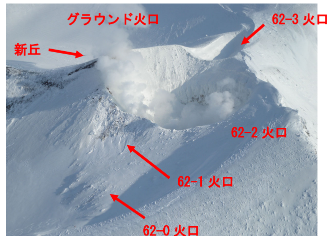
図 5 十勝岳 西側上空（図 3 の②）から見た 62-2 火口の状況
