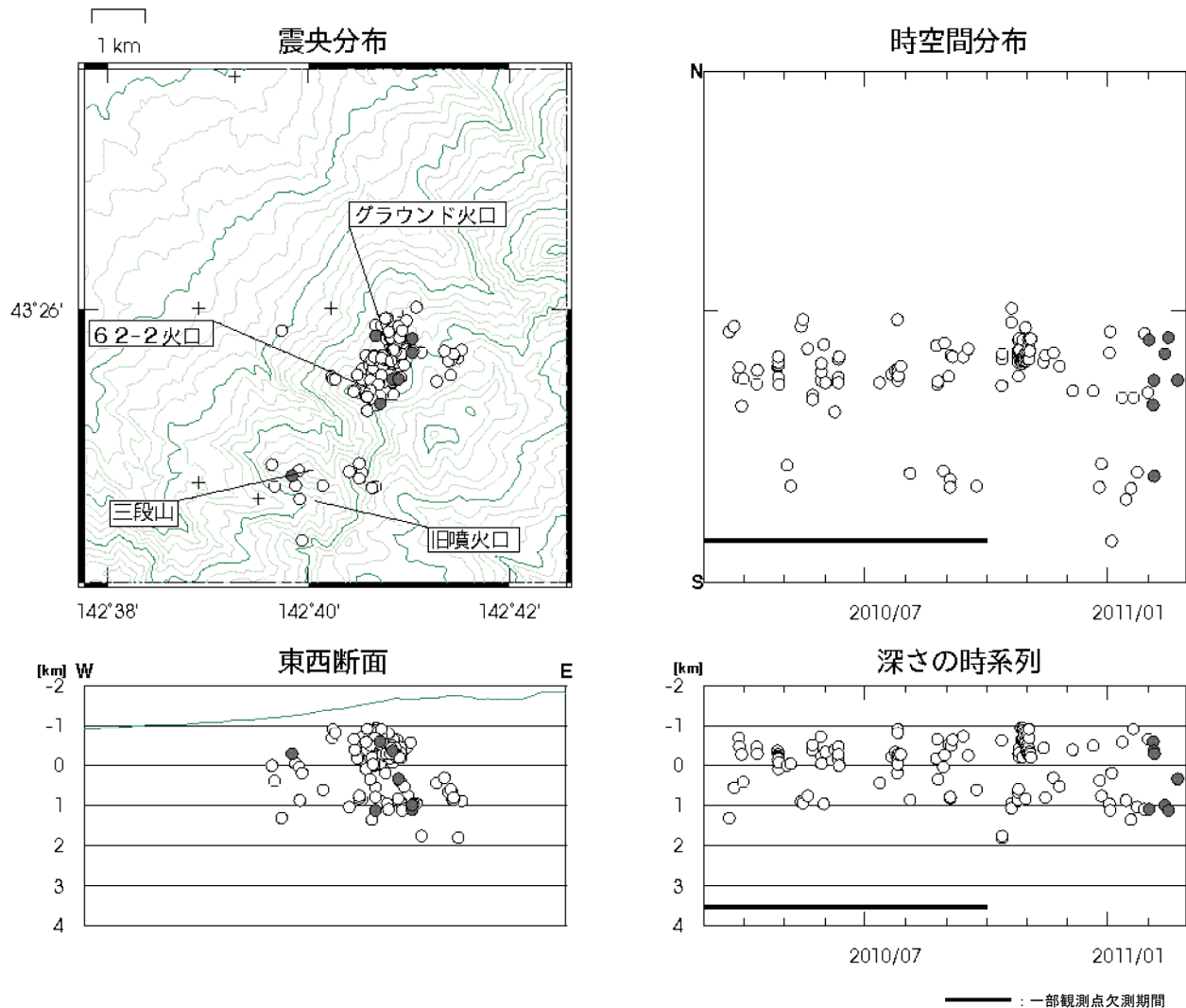
図 7※ 十勝岳 震源分布図（2010 年 3 月～2011 年 2 月、+は地震観測点）
