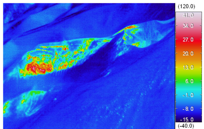
図 6 十勝岳 赤外熱映像装置 1) による 62 火口群及び大正火口の地表面温度分布
