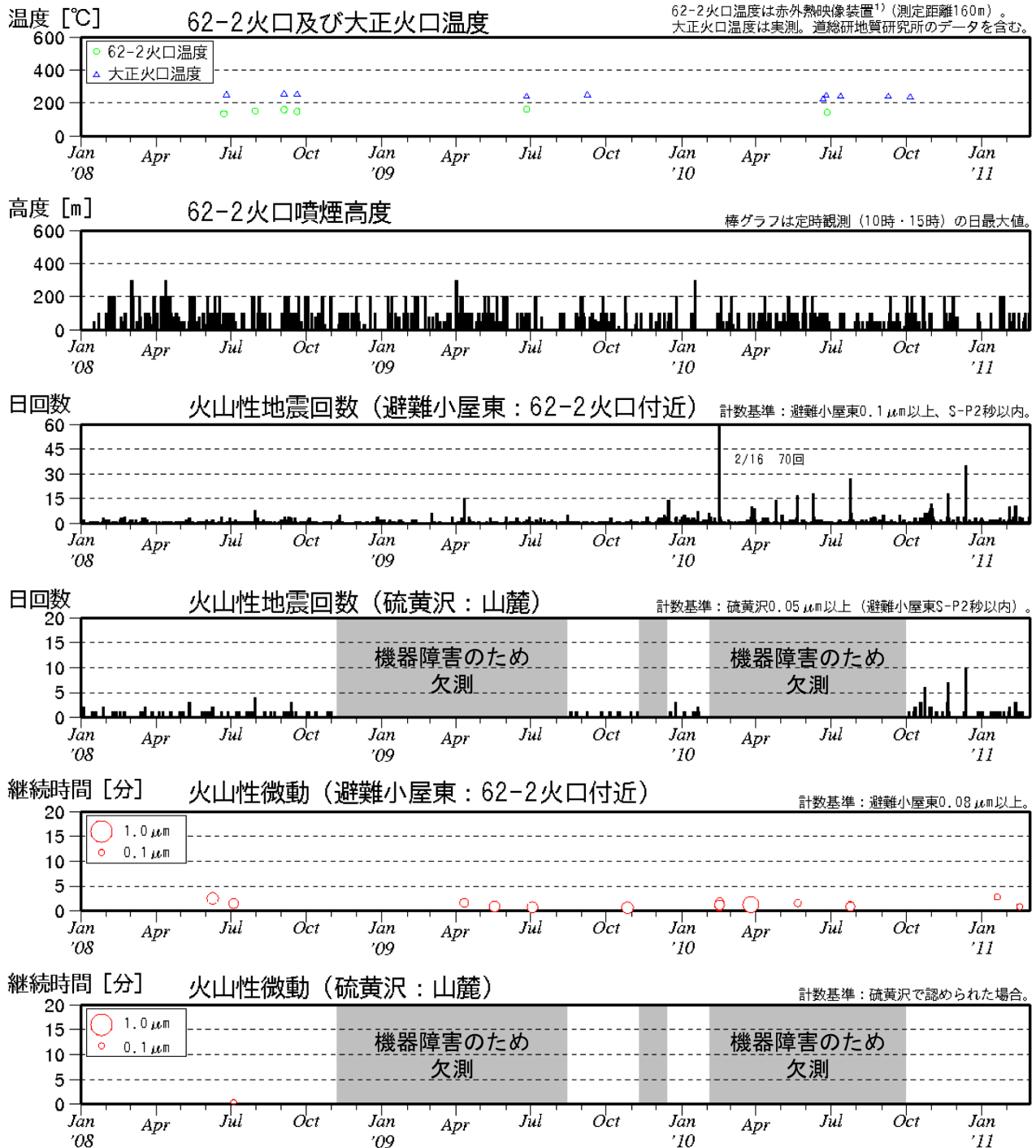
図 2 ※ 十勝岳 最近の火山活動経過図（2008 年 1 月～2011 年 2 月）
