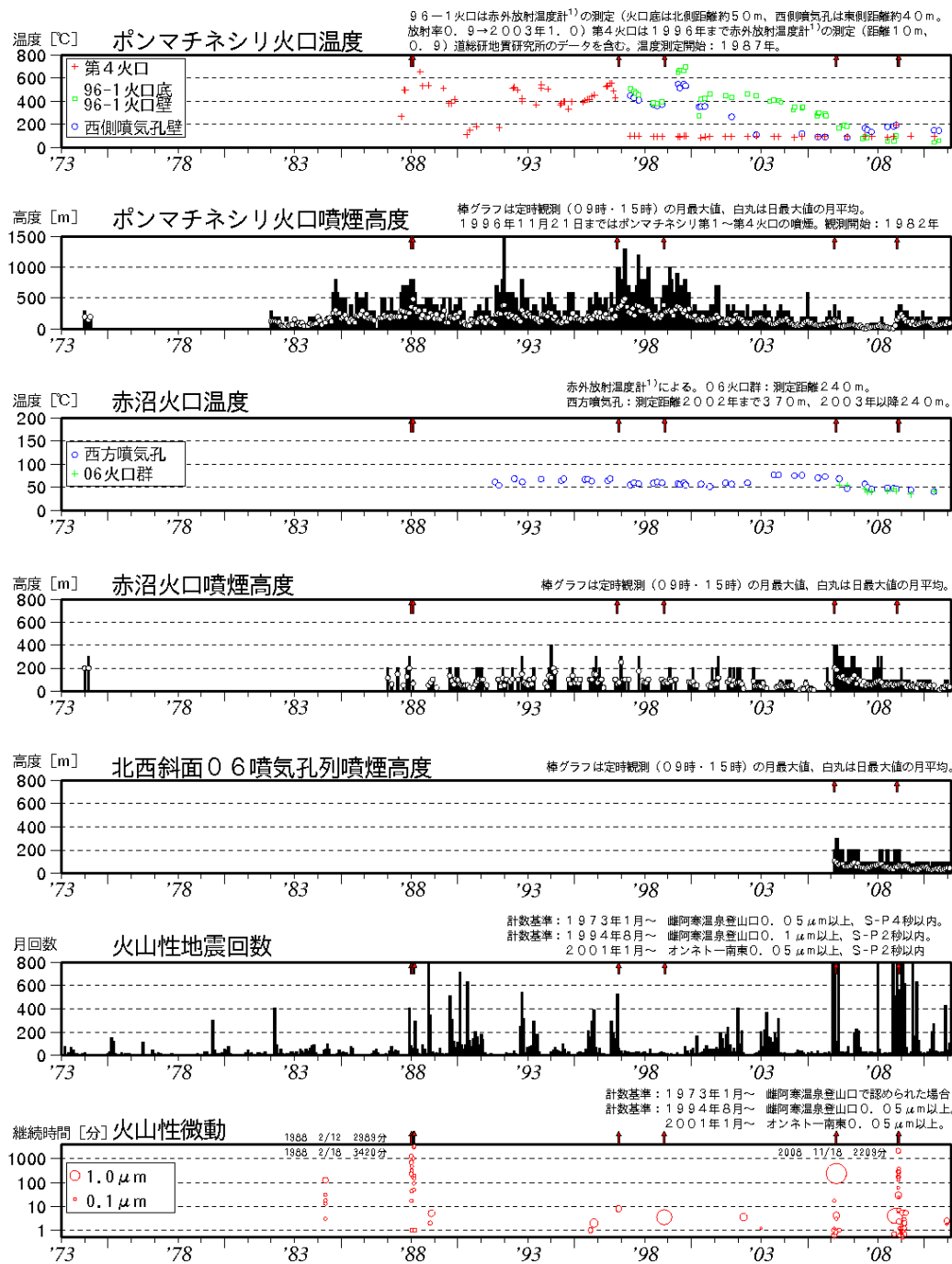
図 1 ※ 雌阿寒岳 長期の火山活動経過図（1973 年 1 月～2011 年 2 月） ↑印は噴火 （1988 年、1996 年、1998 年、2008 年：ポンマチネシリ火口南東側からの噴火、2006 年：赤沼火口からの噴火）
