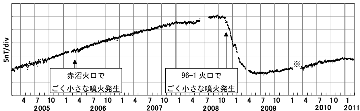
図3 雌阿寒岳 全磁力連続観測結果（2005 年 1 月 1 日～2011 年 2 月 23 日） MEA と地磁気観測所女満別出張所の全磁力単純差（日平均値、年周変化補正） 図4のMEA（◎）にて測定 ※ソーラーパネルへの着雪によりバッテリー電圧が低下し、欠測。
