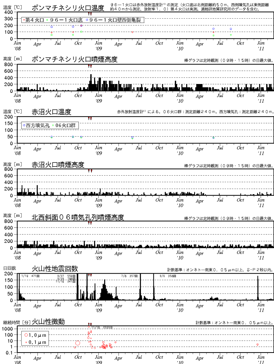
図 2 ※ 雌阿寒岳 最近の火山活動経過図（2008 年 1 月～2011 年 2 月） ↑印は噴火
