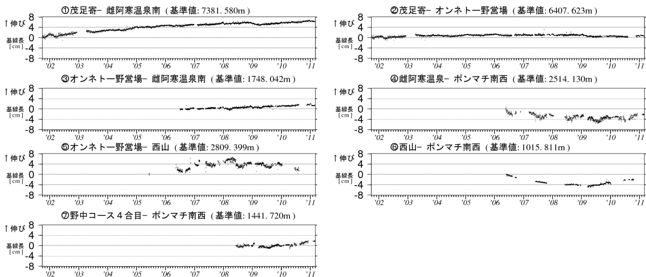
図 6※ 雌阿寒岳 GPS 連続観測による基線長変化（2001 年 10 月～2011 年 2 月） グラフの空白部分は欠測 図 6 の①～⑦は、図 7 の GPS 基線①～⑦に対応しています。
