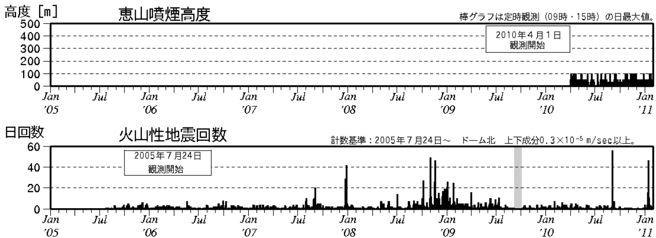
図 1 恵山 最近の火山活動経過図（2005 年 7 月～2011 年 1 月）
