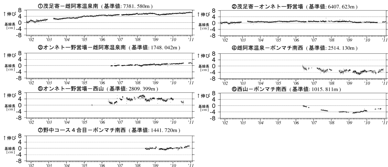
図 6※ 雌阿寒岳 GPS 連続観測による基線長変化（2001 年 10 月～2011 年 1 月） グラフの空白部分は欠測 図 6 の①～⑦は、図 7 の GPS 基線①～⑦に対応しています。
