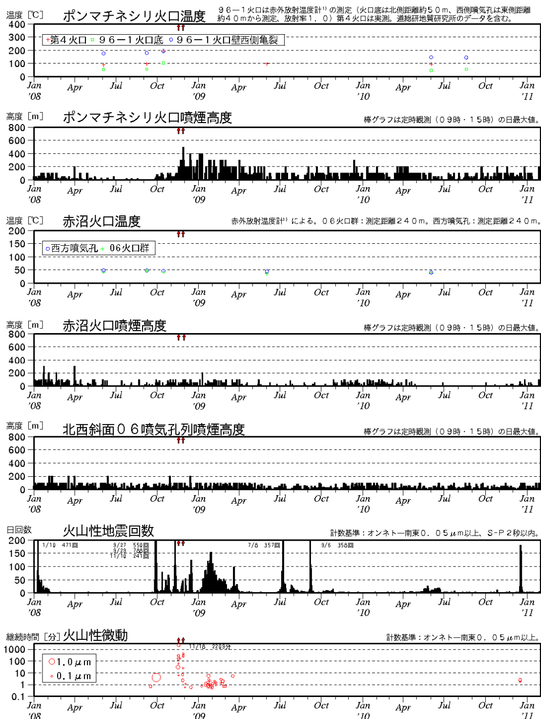
図 2 ※ 雌阿寒岳 最近の火山活動経過図（2008 年 1 月～2011 年 1 月） ↑印は噴火
