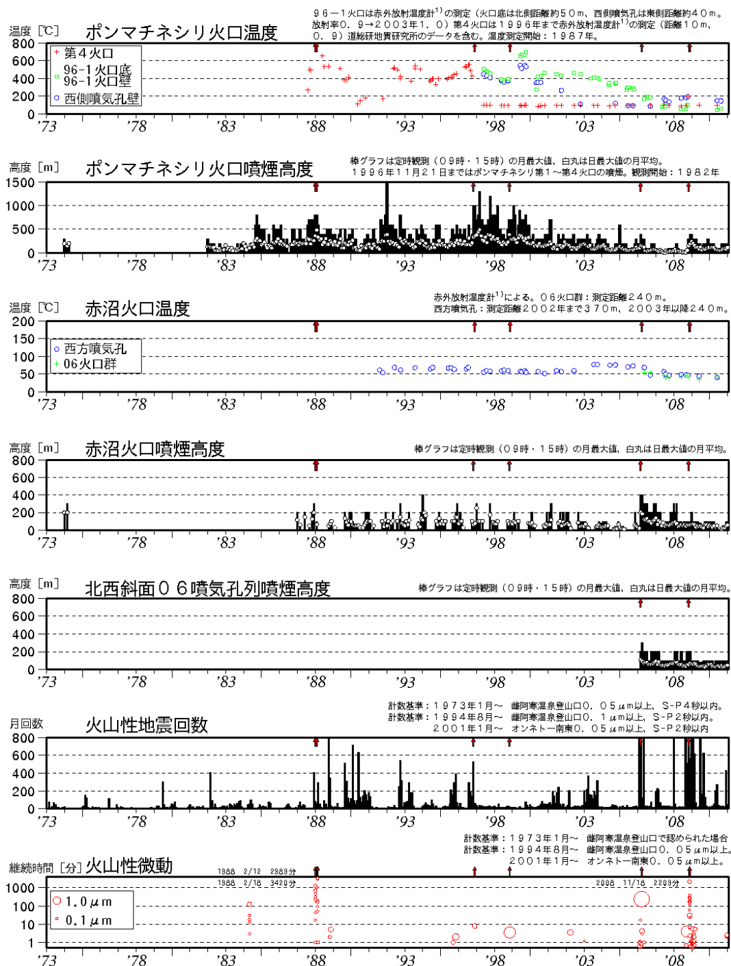
図 1 ※ 雌阿寒岳 長期の火山活動経過図（1973 年 1 月～2011 年 1 月） ↑印は噴火 （1988 年、1996 年、1998 年、2008 年：ポンマチネシリ火口南東側からの噴火、2006 年：赤沼火口からの噴火）
