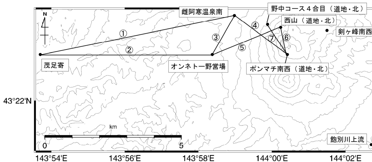
図 7※ 雌阿寒岳 GPS 連続観測点配置図
