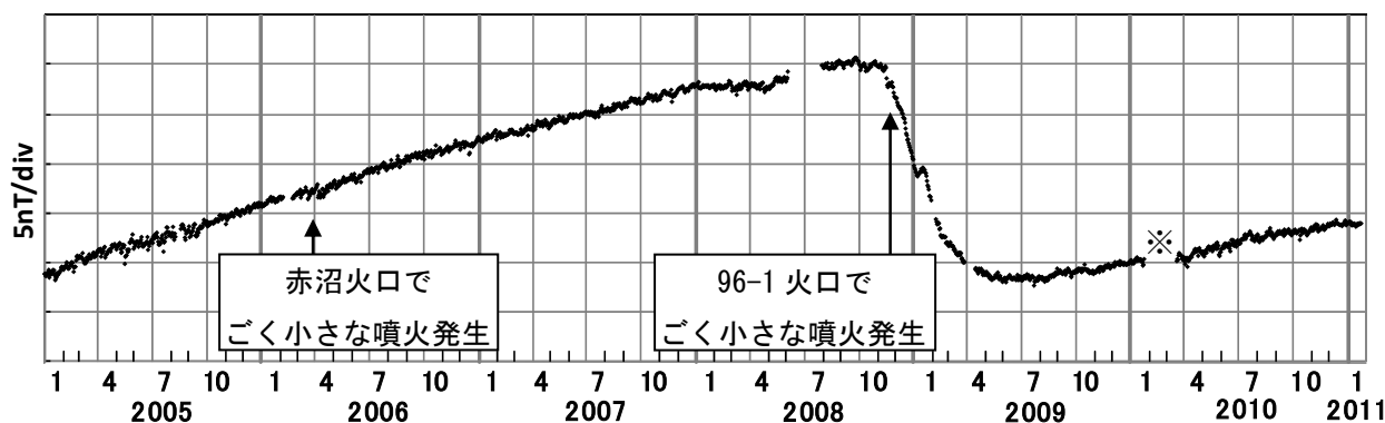
図 3 雌阿寒岳 全磁力連続観測結果（2005 年 1 月 1 日～2011 年 1 月 23 日） MEA と地磁気観測所女満別出張所の全磁力単純差（日平均値、年周変化補正） 図 4 の MEA（◎）にて測定 ※ソーラーパネルへの着雪によりバッテリー電圧が低下し、欠測。
