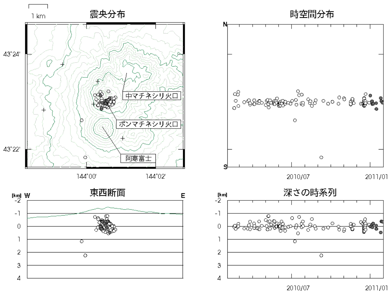
図 5 雌阿寒岳 震源分布図(2010 年 2 月～2011 年 1 月) +は地震観測点
