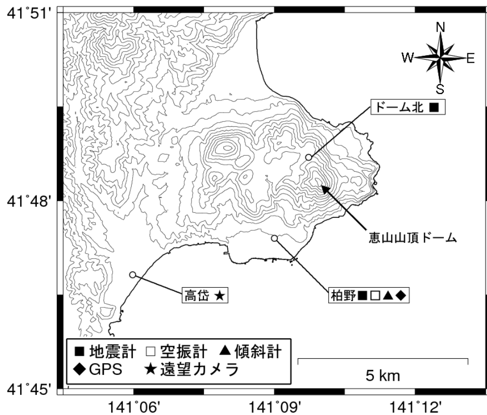
図 2 恵山 観測点配置図
