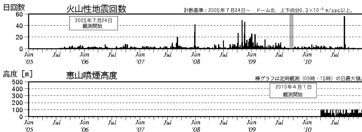
図 1 恵山 最近の火山活動経過図（2005 年 7 月～2010 年 12 月）
