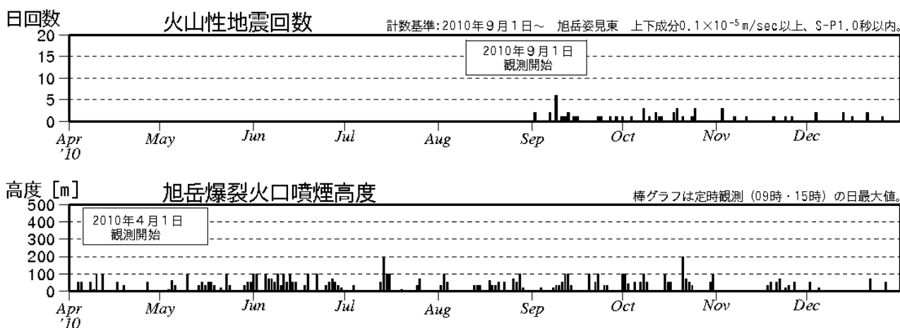
図 1 大雪山 最近の火山活動経過図（2010 年 4 月～12 月）
