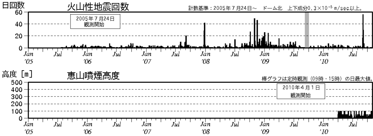
図 2 恵山 最近の火山活動経過図 (2005 年 7 月～2010 年 10 月) 図の灰色の期間は欠測
