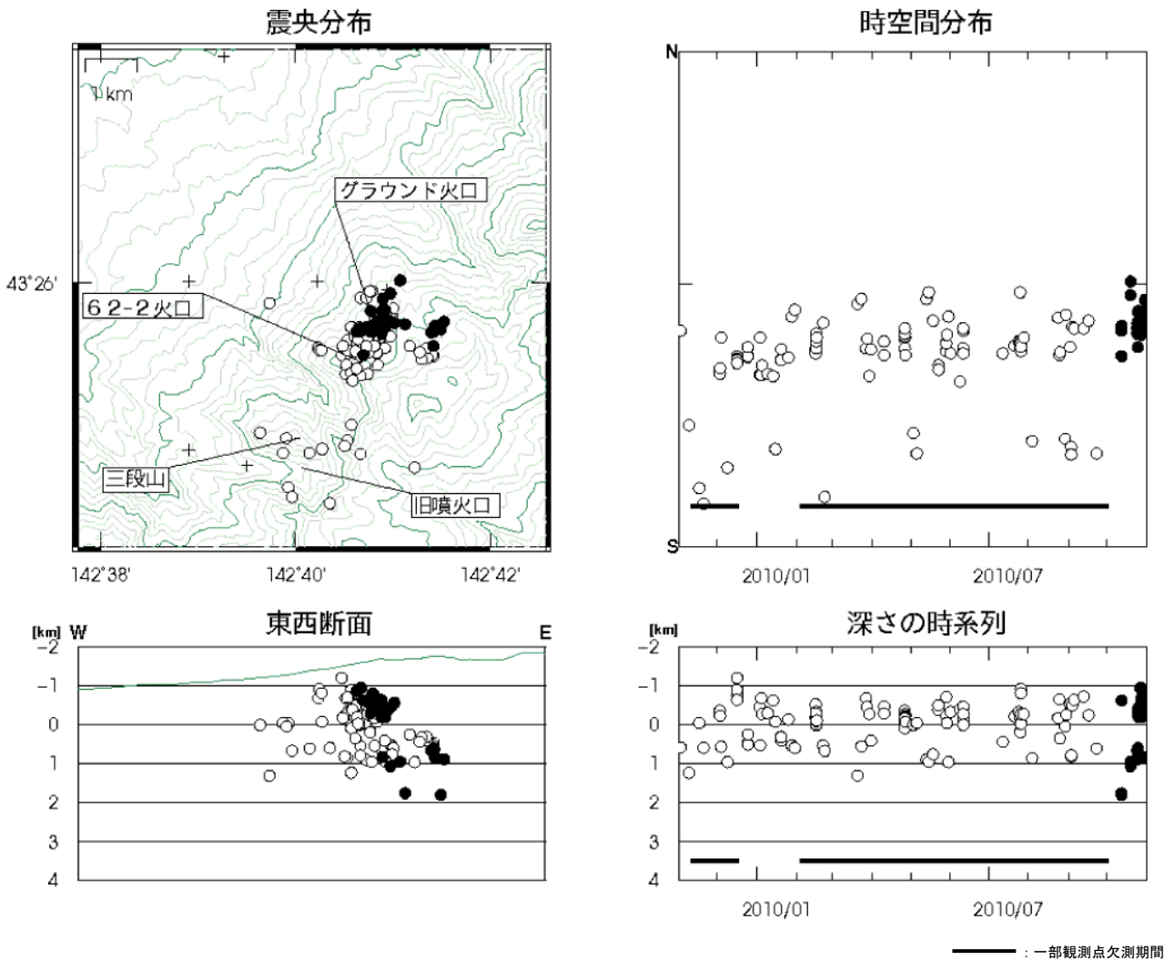
図 3※ 十勝岳 震源分布図 (2009 年 11 月～2010 年 10 月、+は地震観測点)
