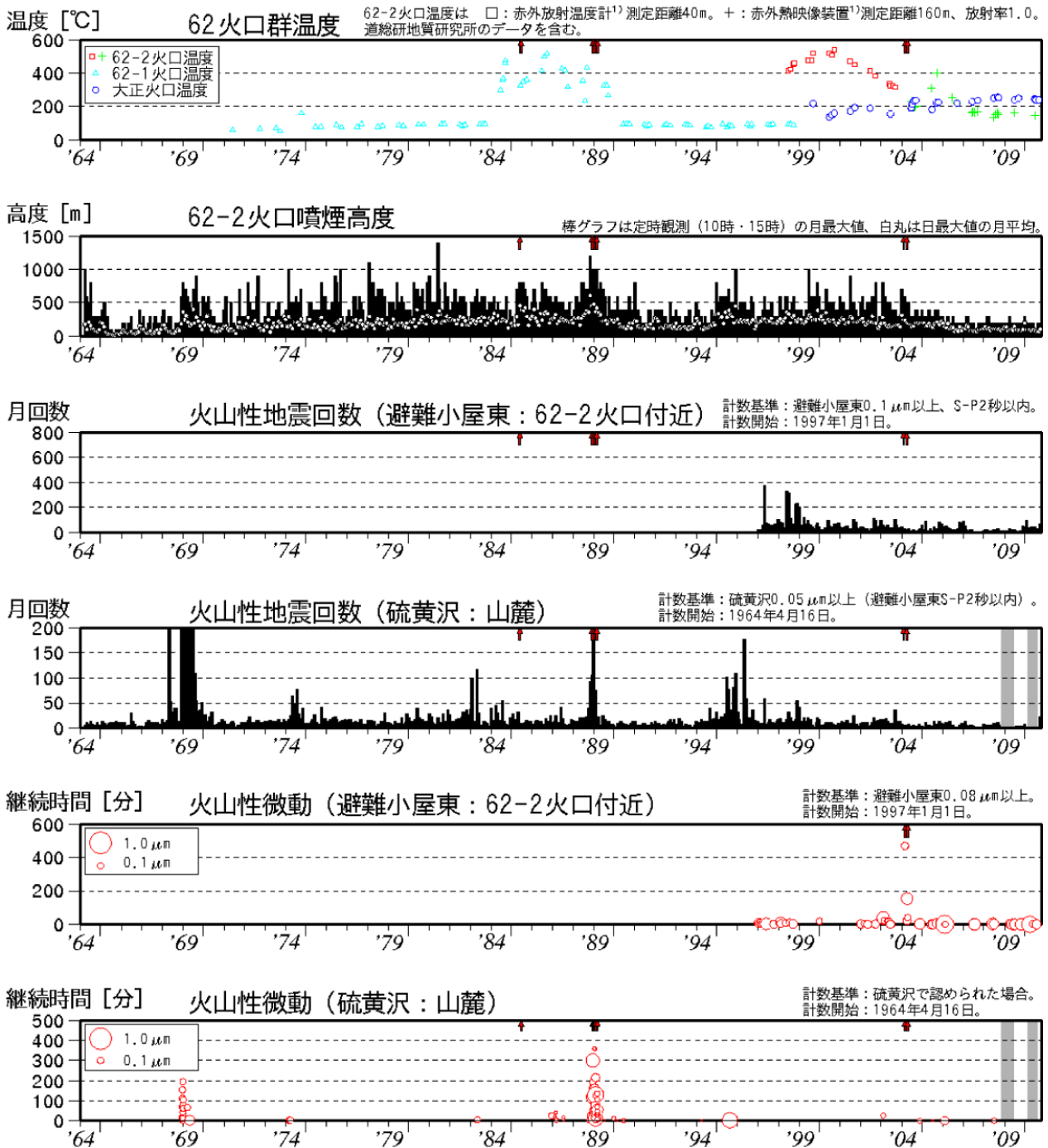
図 1 ※ 十勝岳 長期の火山活動経過図 (1964 年 1 月～2010 年 10 月)
