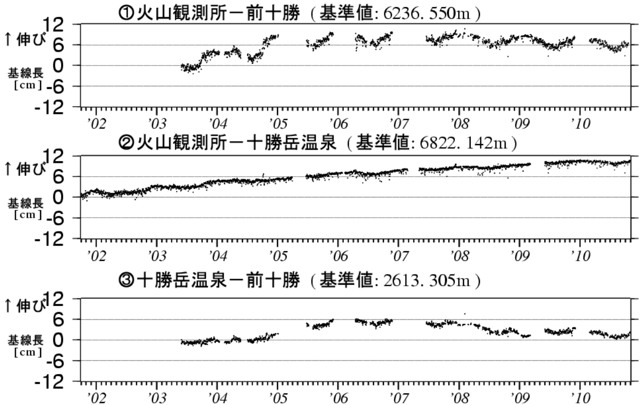
図 4※ 十勝岳 GPS 連続観測による基線長変化 (2001 年 10 月～2010 年 10 月)
