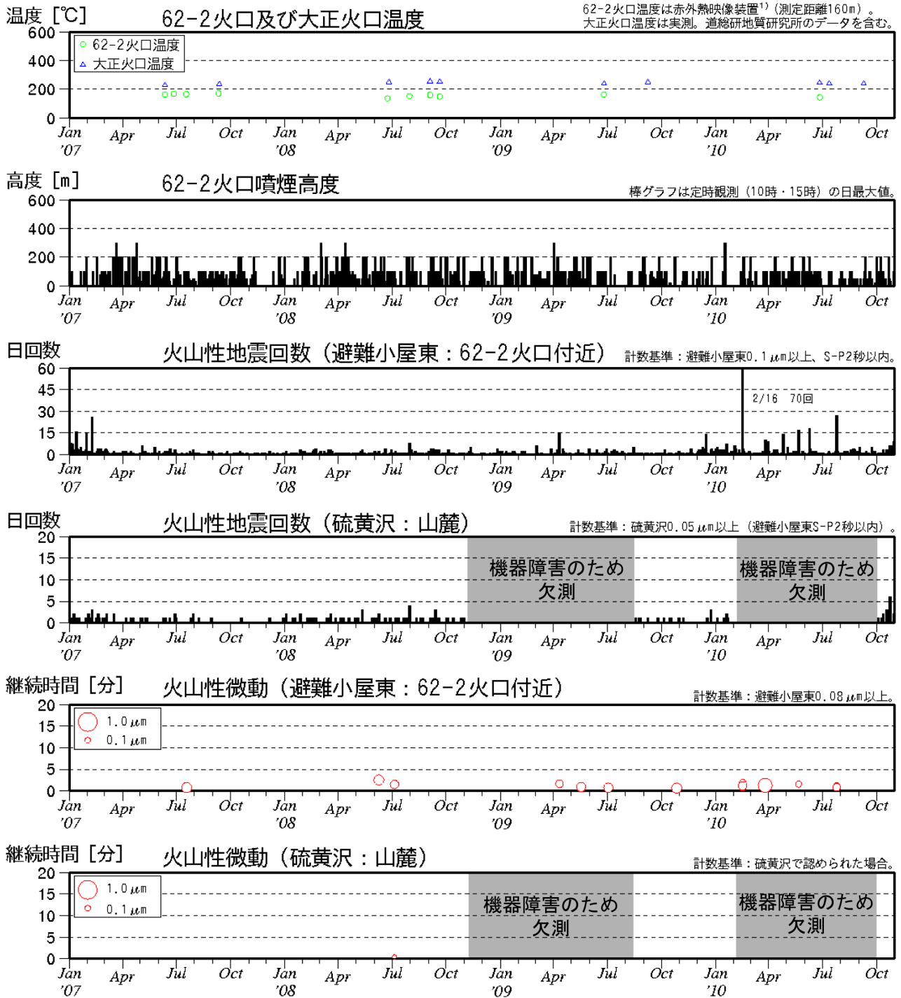
図 2※ 十勝岳 最近の火山活動経過図 (2007 年 1 月～2010 年 10 月)
