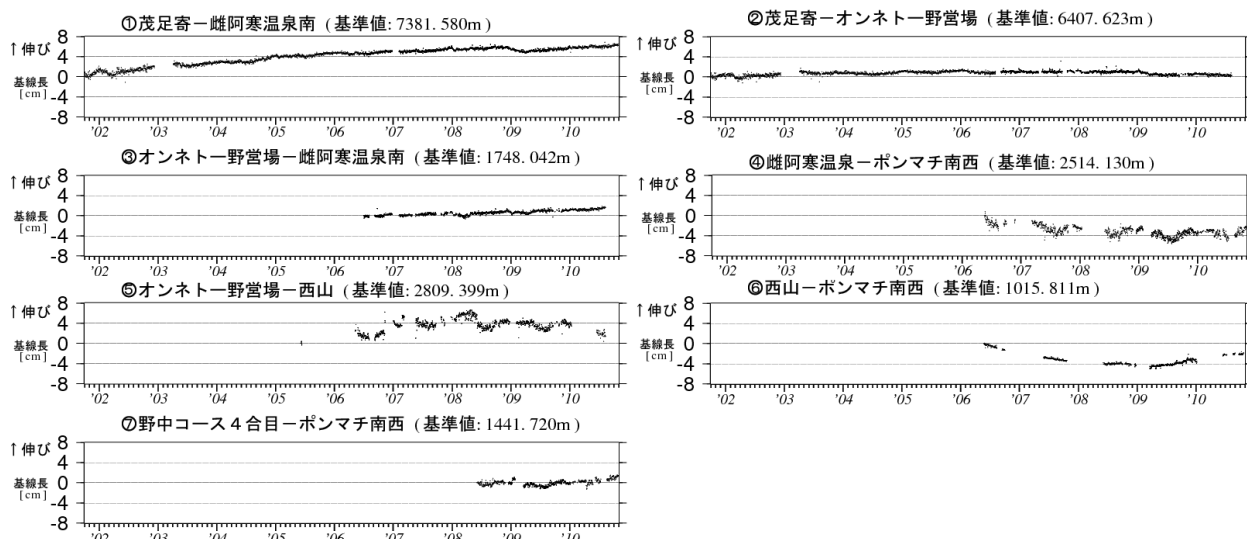
図 6※ 雌阿寒岳 GPS 連続観測による基線長変化（2001 年 10 月～2010 年 10 月） グラフの空白部分は欠測 図 6 の①～⑦は、図 7 の GPS 基線①～⑦に対応しています。
