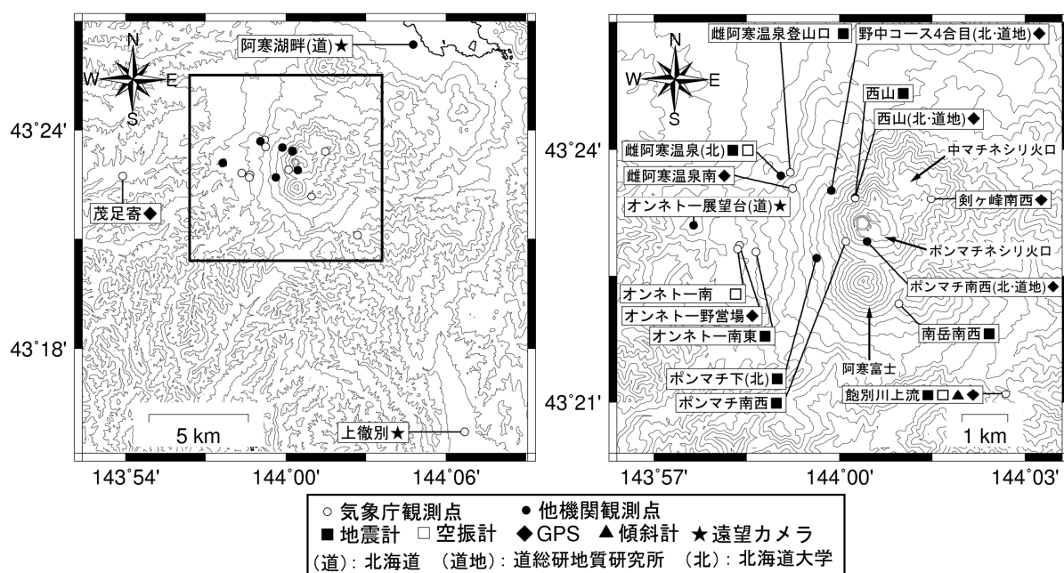
図 8 雌阿寒岳 観測点配置図
