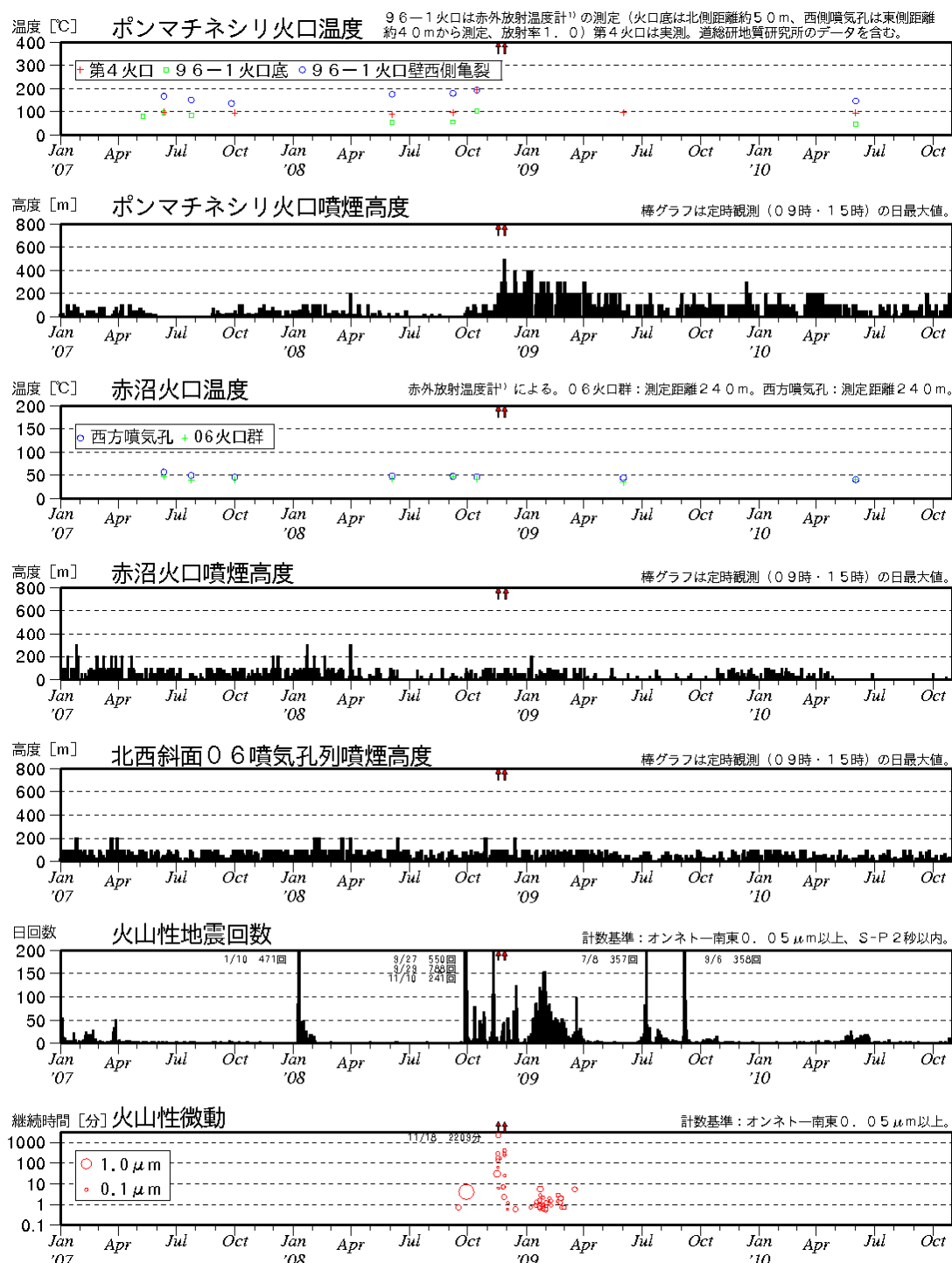
図 2 ※ 雌阿寒岳 最近の火山活動経過図（2007 年 1 月～2010 年 10 月） ↑印は噴火
