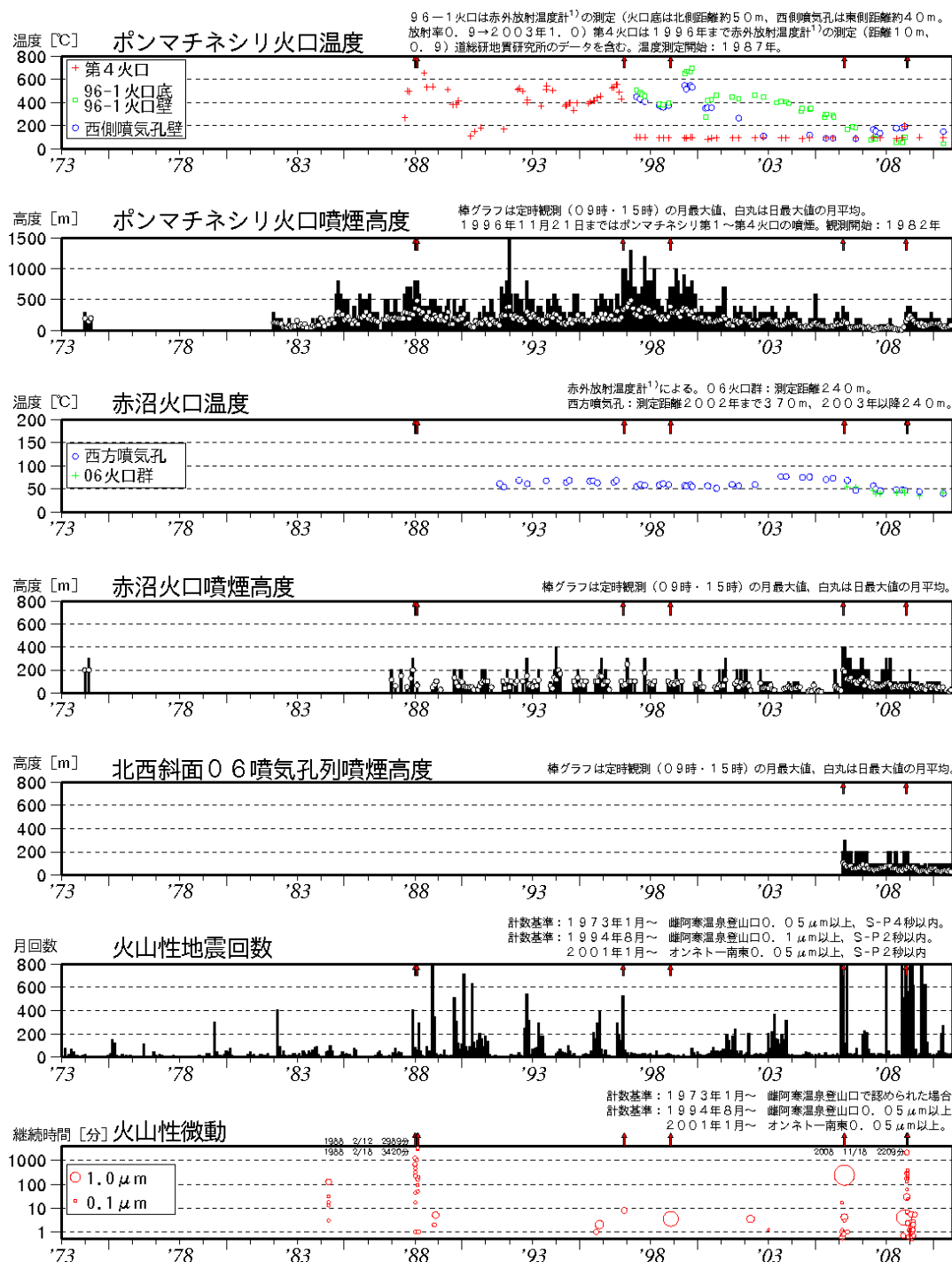
図 1 ※ 雌阿寒岳 長期の火山活動経過図（1973 年 1 月～2010 年 10 月） ↑印は噴火 （1988 年、1996 年、1998 年、2008 年：ポンマチネシリ火口南東側からの噴火、2006 年：赤沼火口からの噴火）
