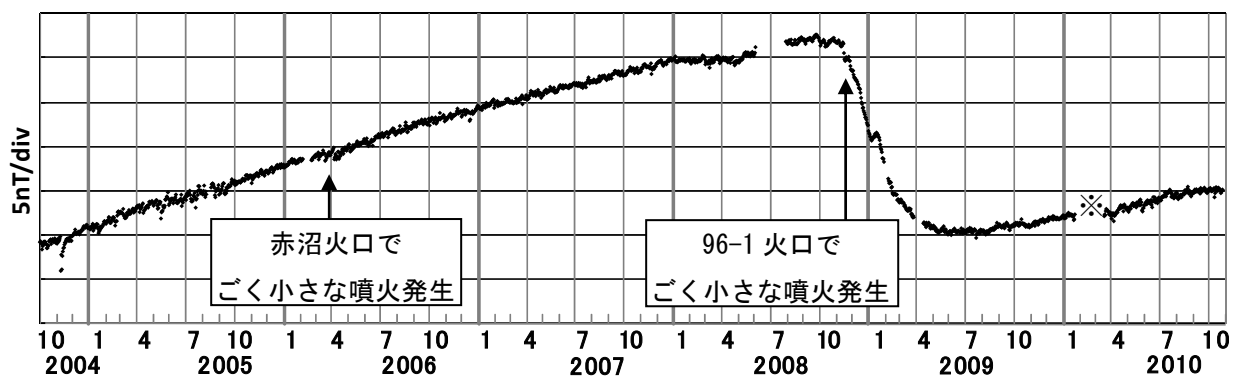
図3 雌阿寒岳 全磁力連続観測結果（2004年10月1日～2010年10月27日） MEAと地磁気観測所女満別出張所の全磁力単純差（日平均値、年周変化補正） 図4のMEA（◎）にて測定 ※ソーラーパネルへの着雪によりバッテリー電圧が低下し、欠測。
