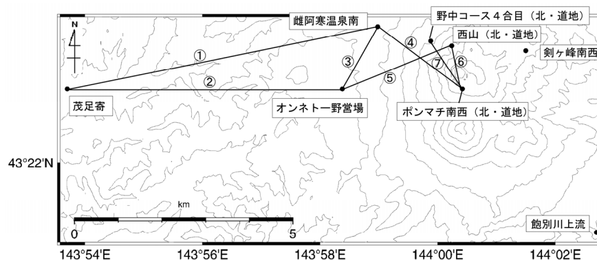
図 7※ 雌阿寒岳 GPS 連続観測点配置図
