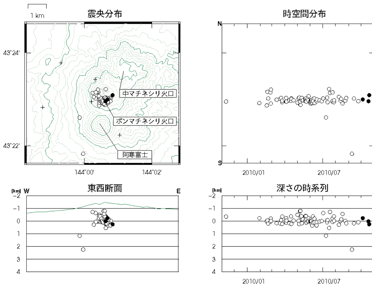
図 5 雌阿寒岳 震源分布図(2009 年 11 月～2010 年 10 月) +は地震観測点
