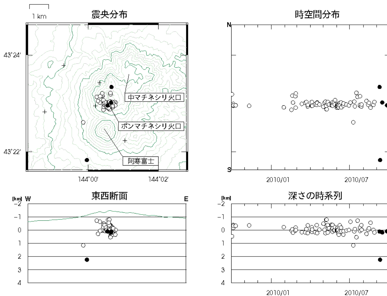
図 5 雌阿寒岳 震源分布図(2009 年 10 月～2010 年 9 月) +は地震観測点
