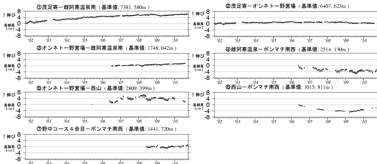
図6※ 雌阿寒岳 GPS 連続観測による基線長変化（2001年10月～2010年9月） グラフの空白部分は欠測 図6の①～⑦は、図7のGPS基線①～⑦に対応しています。
