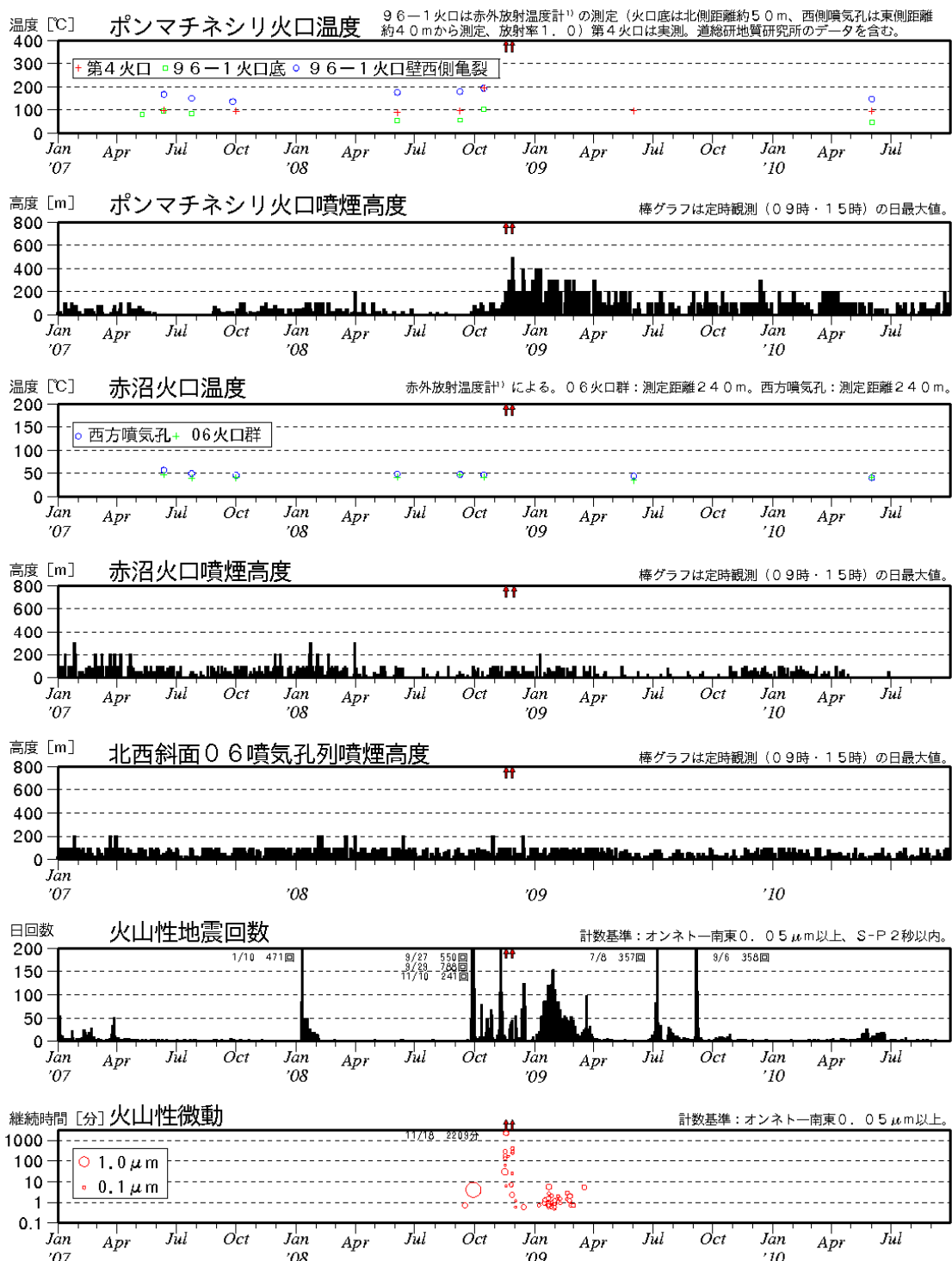
図2※ 雌阿寒岳 最近の火山活動経過図（2007年1月～2010年9月） ↑印は噴火
