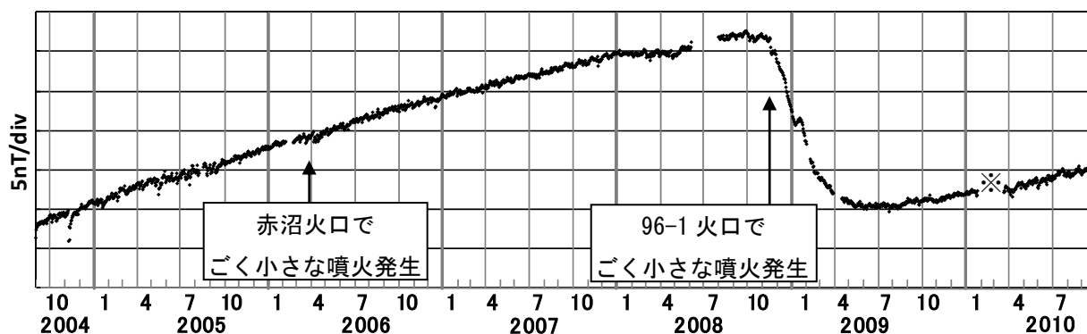
図3 雌阿寒岳 全磁力連続観測結果（2004年7月1日～2010年9月23日） MEAと地磁気観測所女満別出張所の全磁力単純差（日平均値、年周変化補正） 図4のMEA（◎）にて測定 ※ソーラーパネルへの着雪によりバッテリー電圧が低下し、欠測。
