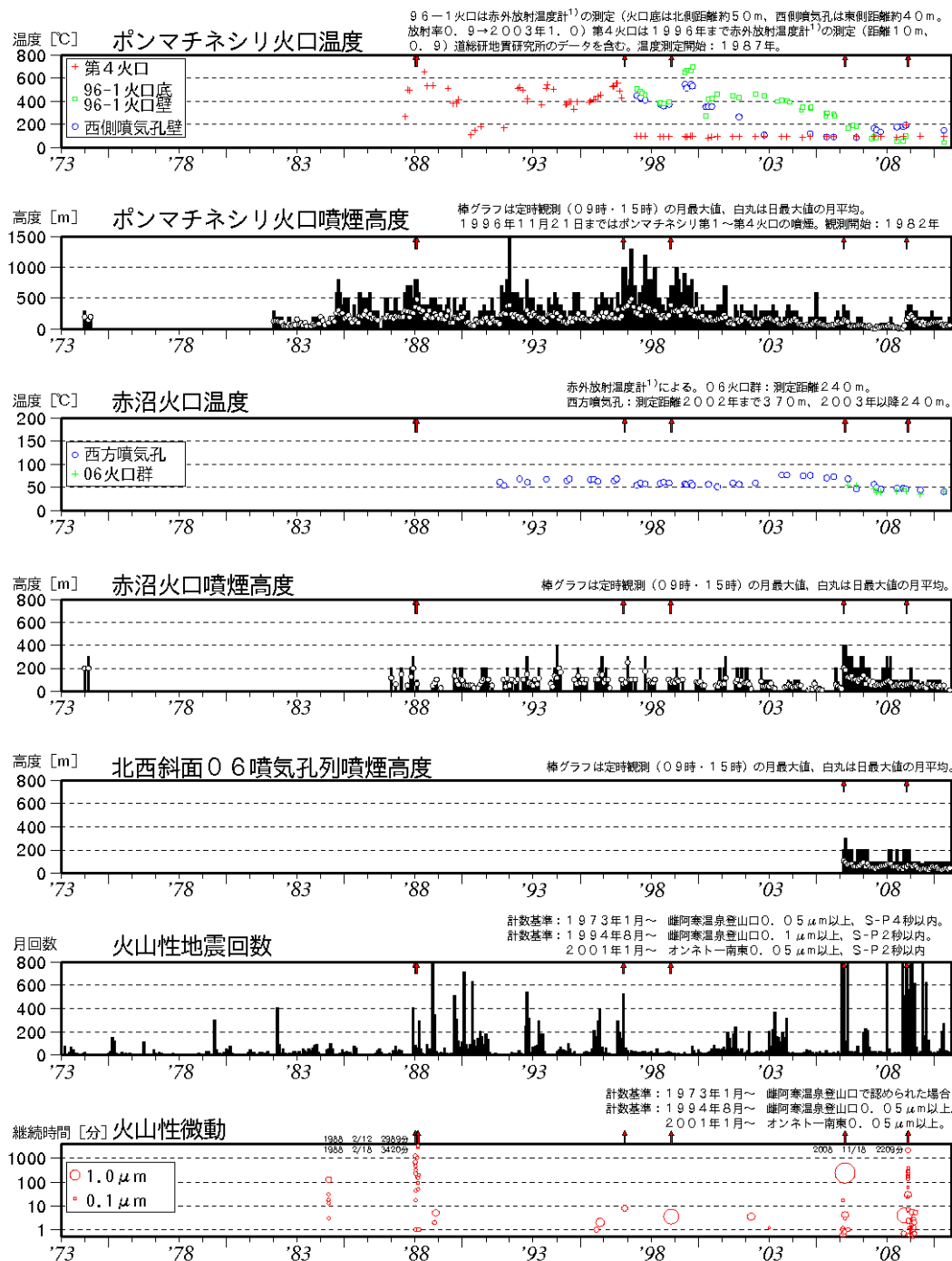
図 1 ※ 雌阿寒岳 長期の火山活動経過図（1973 年 1 月～2010 年 9 月） ↑印は噴火 （1988 年、1996 年、1998 年、2008 年：ポンマチネシリ火口南東側からの噴火、2006 年：赤沼火口からの噴火）
