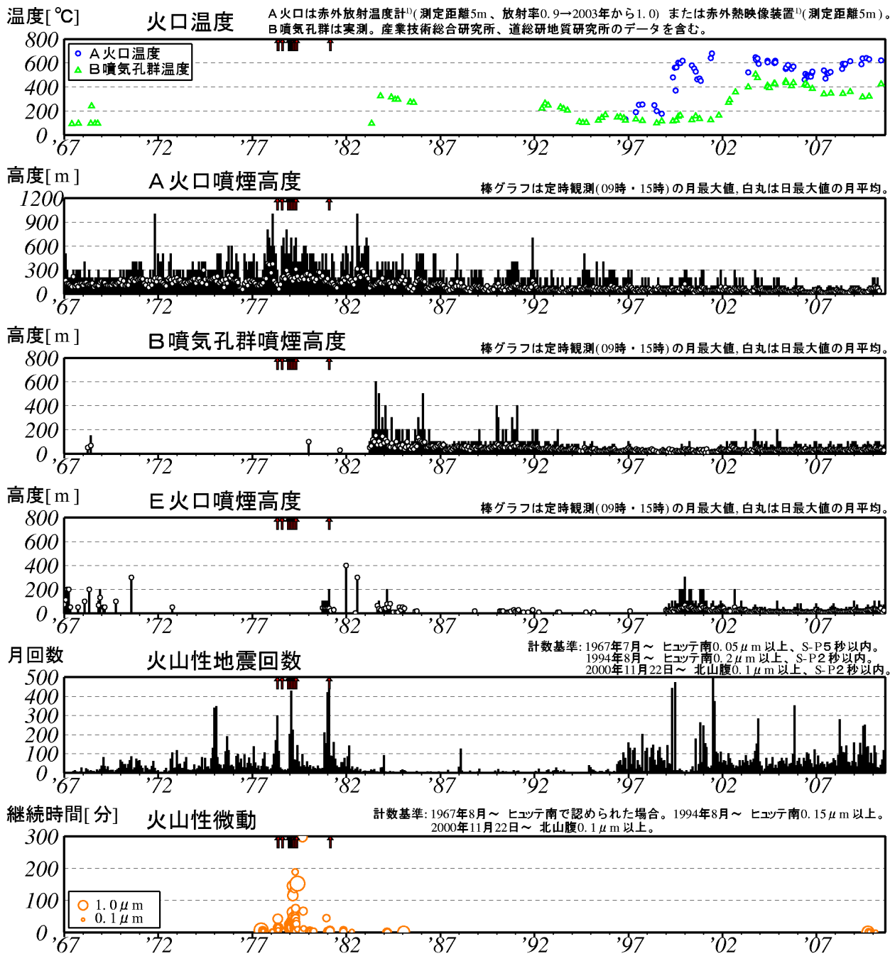
図 1※ 樽前山 長期の火山活動経過図 (1967年 1 月～2010年 8 月) ↑印は噴火
