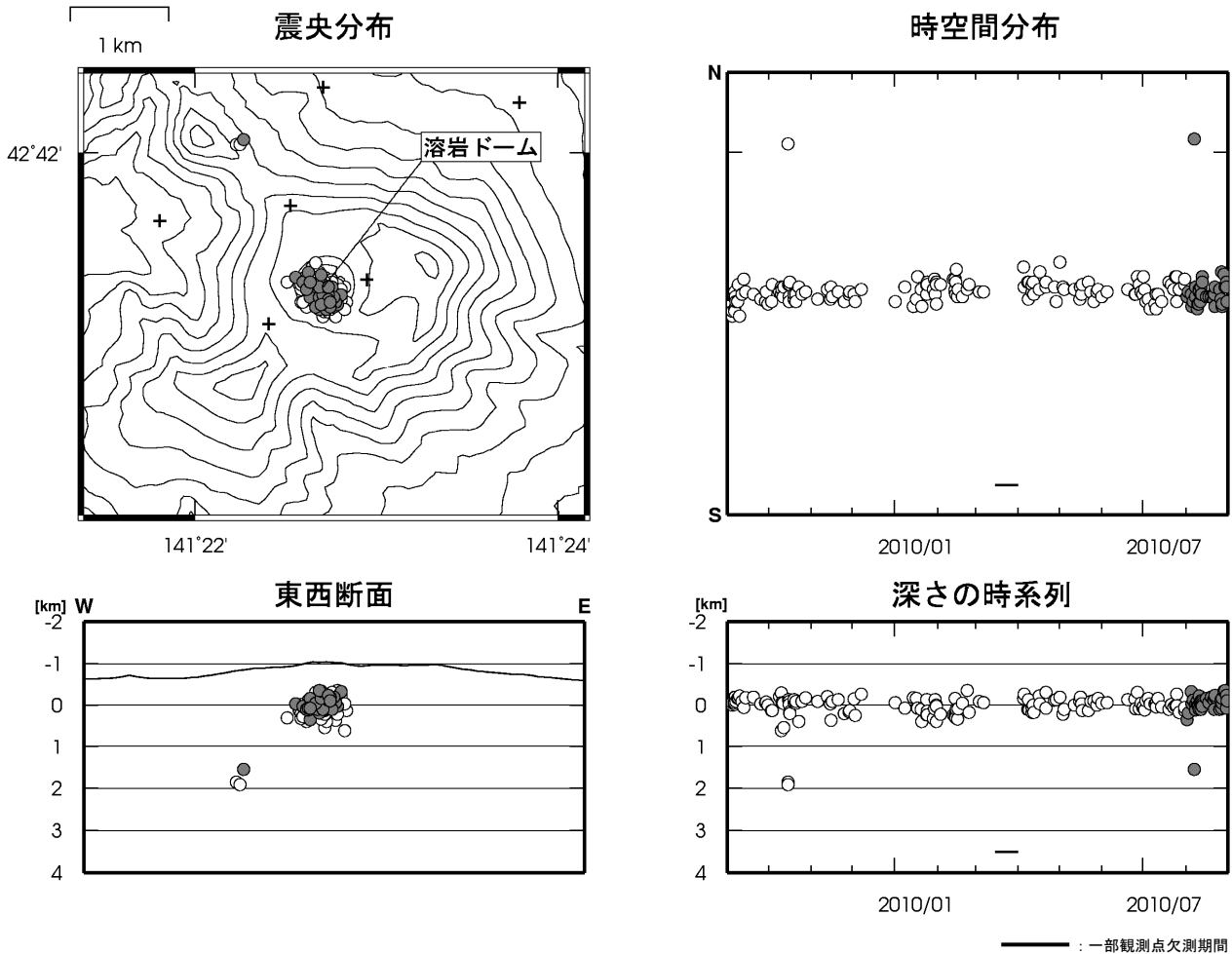
図 3※ 樽前山 震源分布図 (2009 年 9 月~2010 年 8 月、+は地震観測点)
