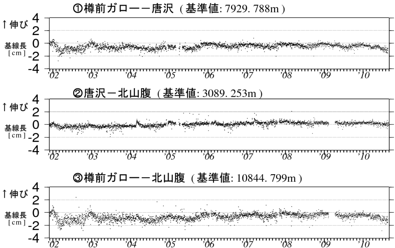
図 4 樽前山 GPS 連続観測による基線長変化 (2001 年 12 月～2010 年 8 月)
