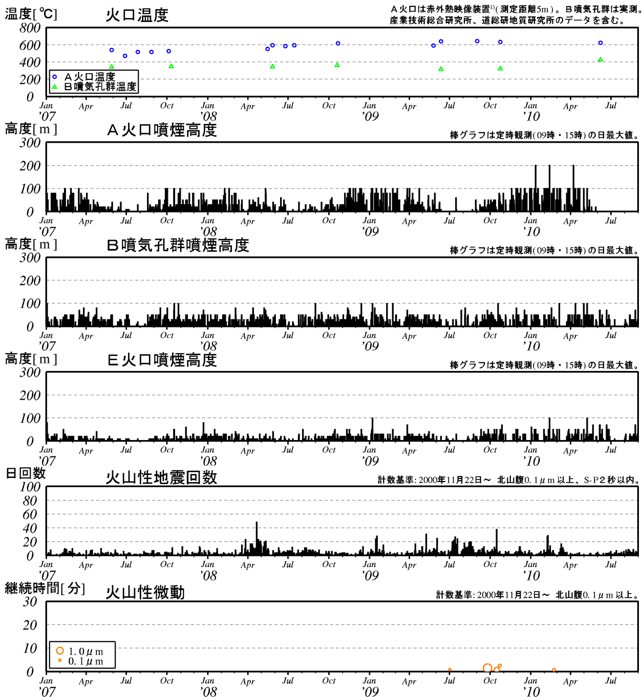
図 2※ 樽前山 最近の火山活動経過図 (2007 年 1 月～2010 年 8 月)
