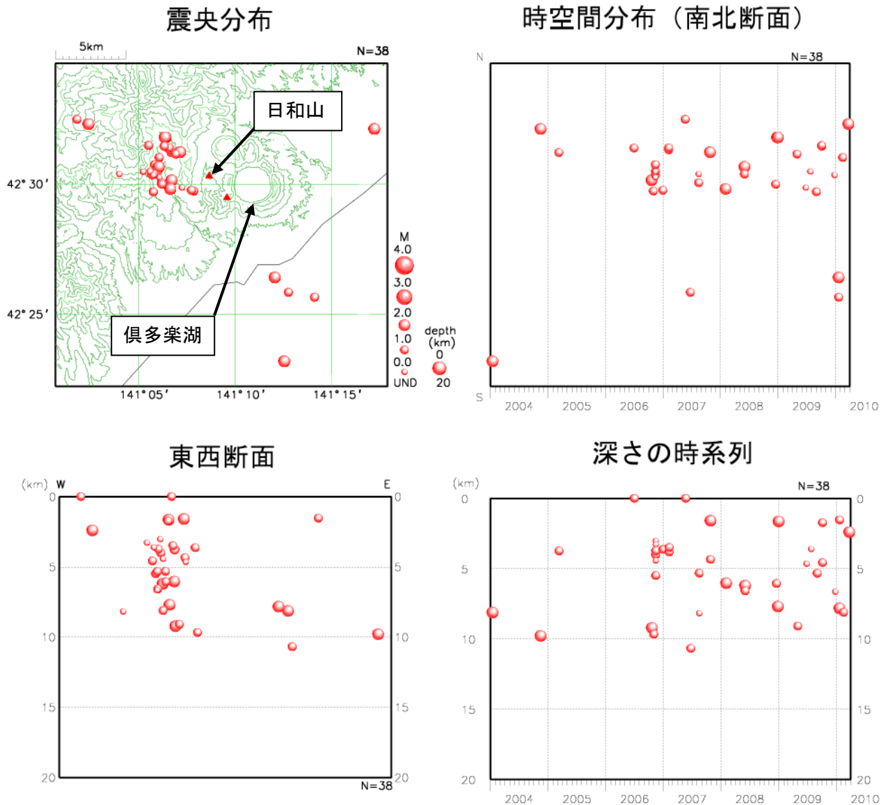
図 2 広域ネットによる倶多楽周辺の地震活動 (2004 年 1 月～2010 年 3 月)
