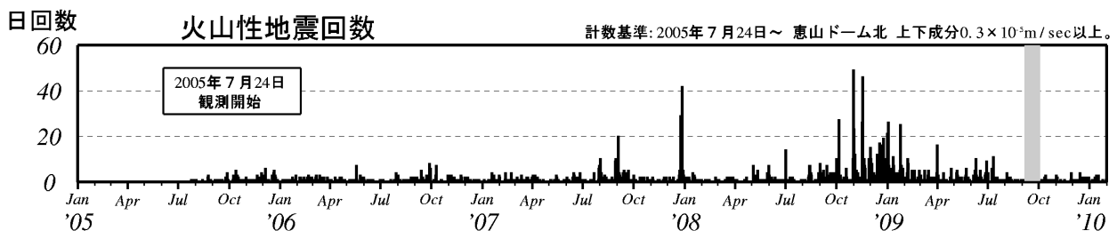
図 2 恵山 日別地震回数（2005 年 7 月～2010 年 1 月）
