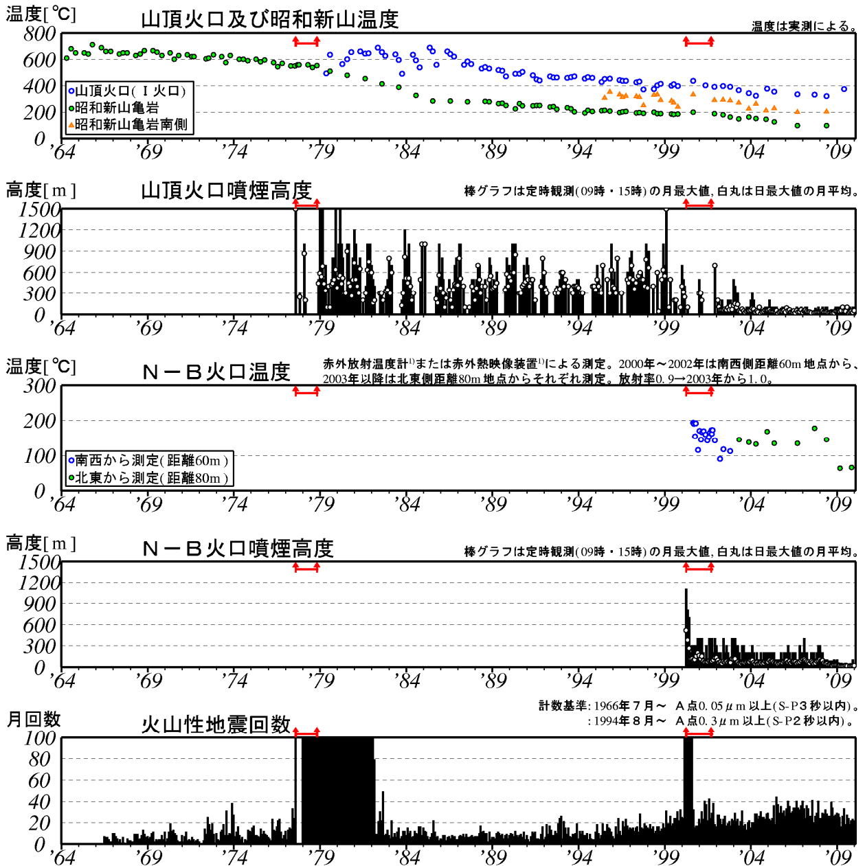
図 2 有珠山 長期の火山活動経過図（1964 年 1 月～2010 年 1 月）
