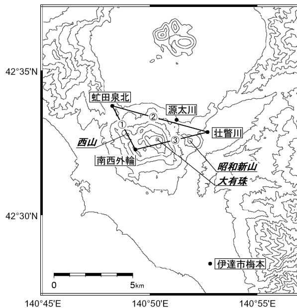
図6 有珠山 GPS 連続観測点配置図
