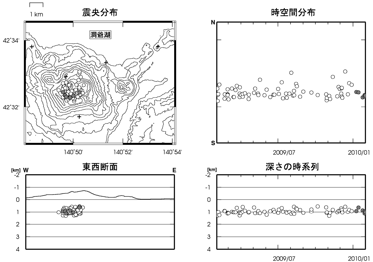
図 4 有珠山 震源分布図（2009 年 2 月～2010 年 1 月、+は地震観測点）
