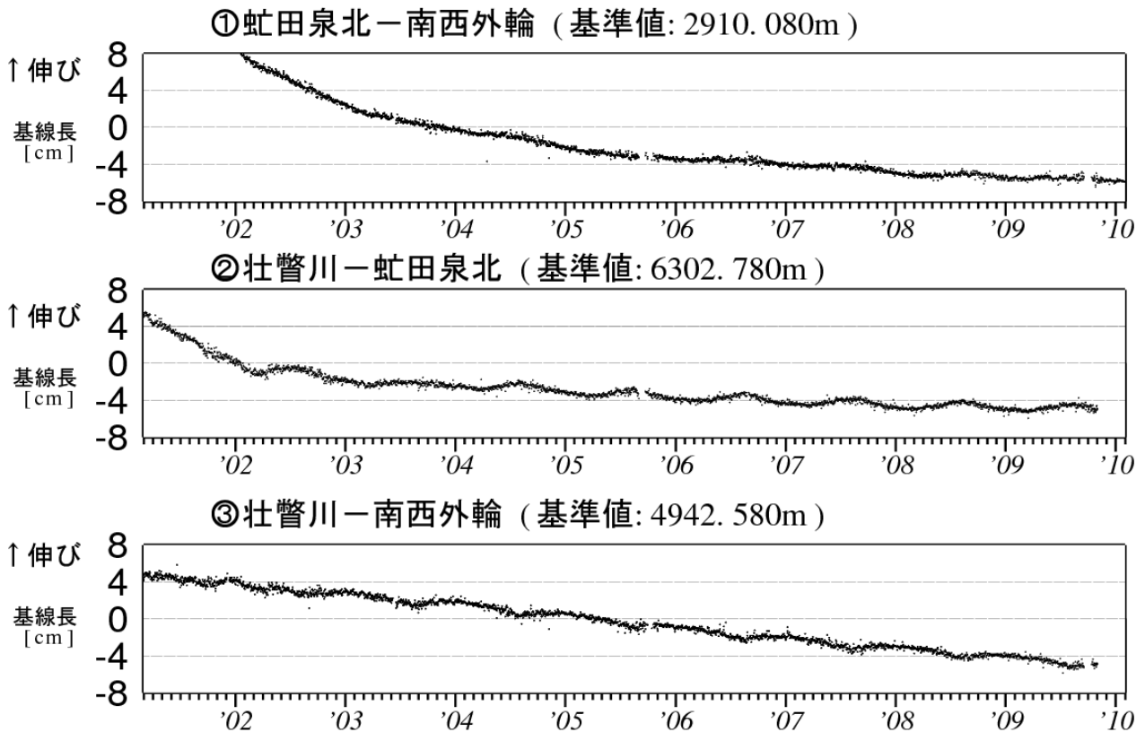
図5 有珠山 GPS 連続観測による基線長変化（2001年3月～2010年1月）
