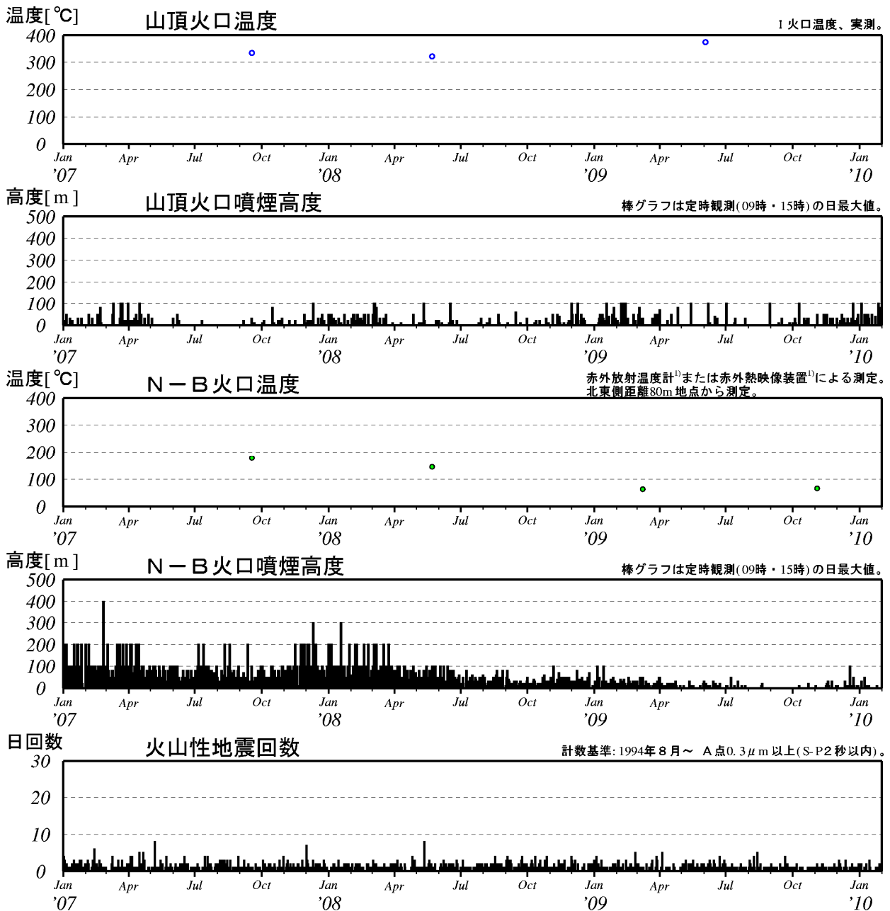
図3 有珠山 最近の火山活動経過図（2007年1月～2010年1月）
