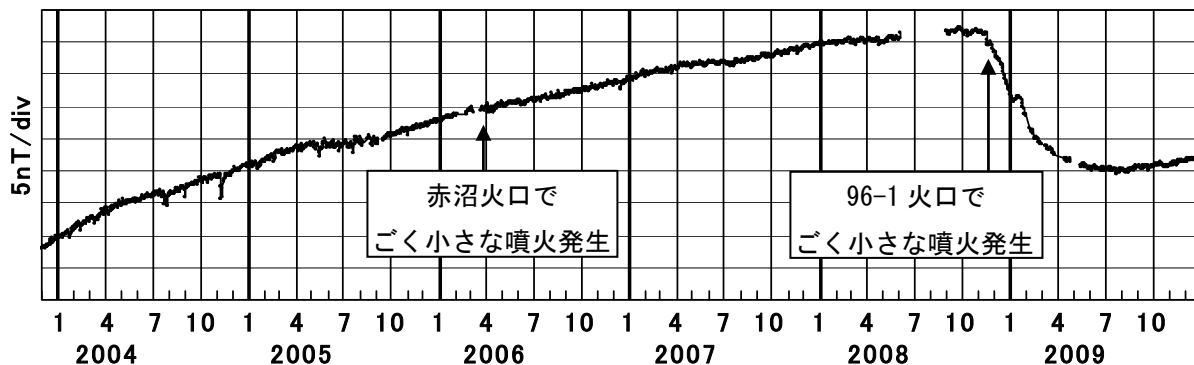
図 4 雌阿寒岳 全磁力連続観測結果（2003 年 12 月 1 日～2009 年 12 月 31 日） MEA と地磁気観測所女満別出張所の全磁力単純差（日平均値） 図 5 の MEA (◎) にて測定
