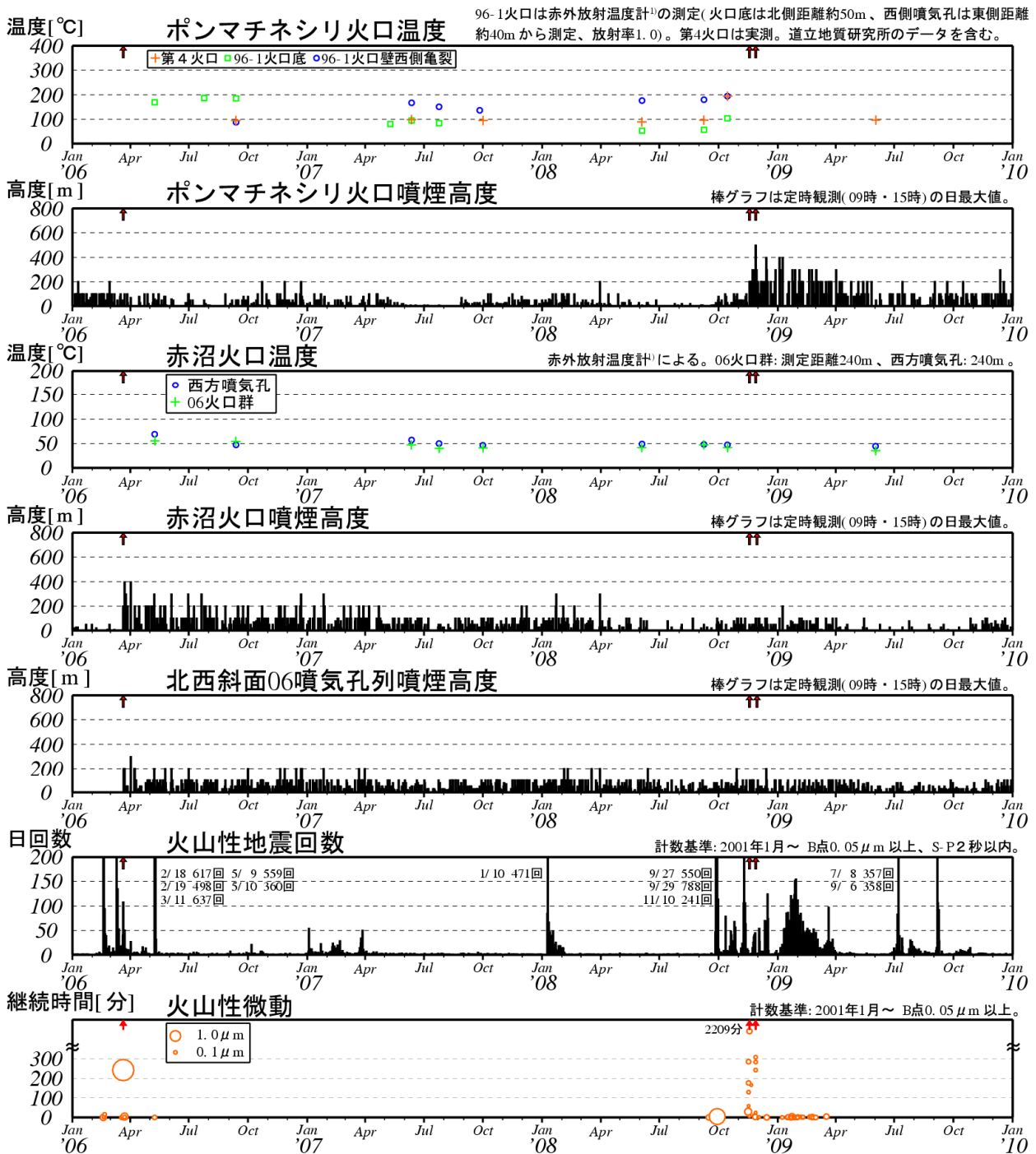
図3※ 雌阿寒岳 最近の火山活動経過図（2006年1月～2009年12月） ↑印は噴火
