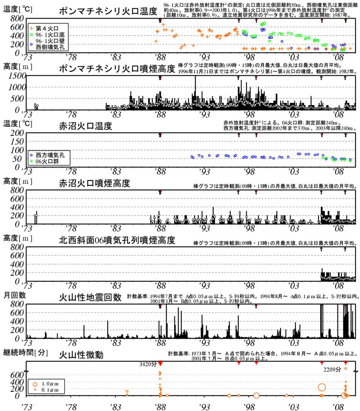
図 2 ※ 雌阿寒岳 長期の火山活動経過図（1973 年 1 月～2009 年 12 月） ↑印は噴火 （1988 年、1996 年、1998 年、2008 年：ポンマチネシリ火口南東側からの噴火、2006 年：赤沼火口からの噴火）
