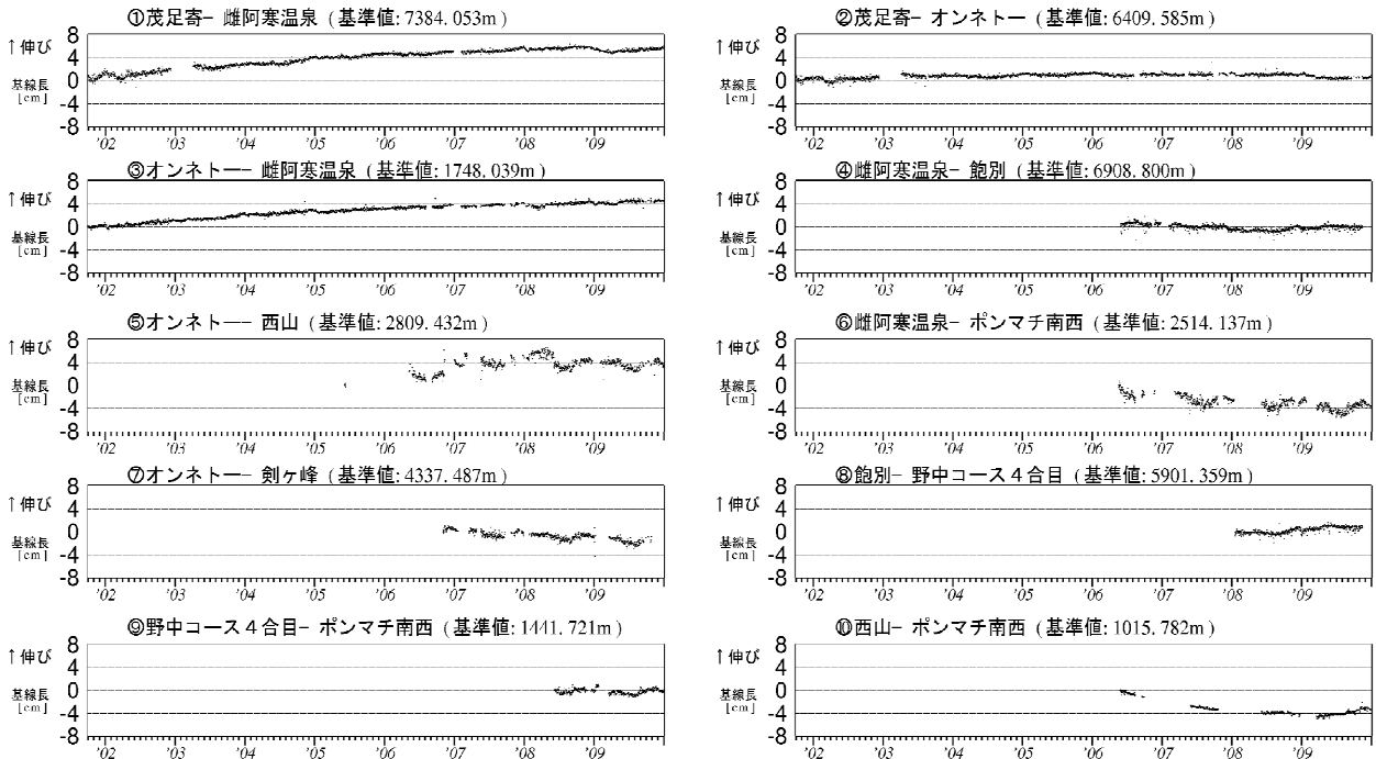
図 7※ 雌阿寒岳 GPS 連続観測による基線長変化（2001 年 10 月～2009 年 12 月） グラフの空白部分は欠測 図 7 の①～⑩は、図 8 の GPS 基線①～⑩に対応しています。
