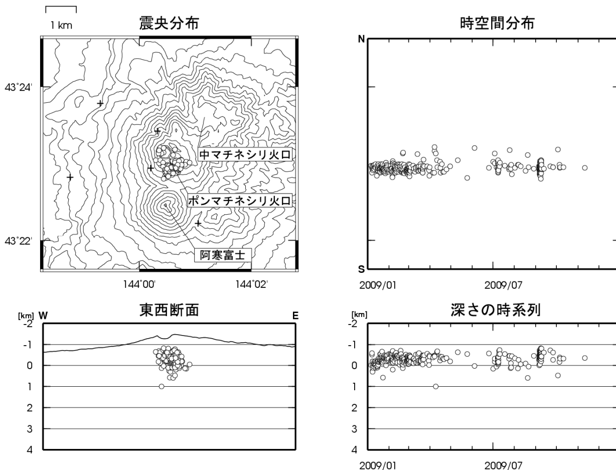
図 6 雌阿寒岳 震源分布図(2009 年 1 月～2009 年 12 月) +は地震観測点
