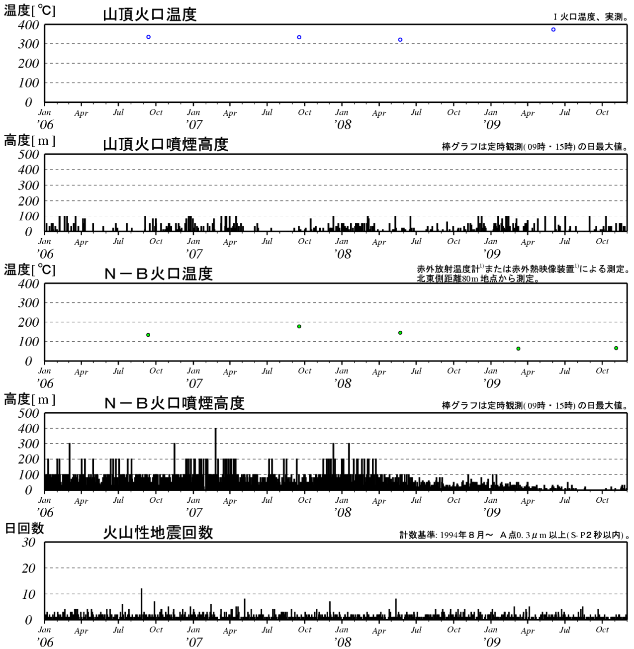
図3 有珠山 最近の火山活動経過図（2006年1月～2009年11月）
