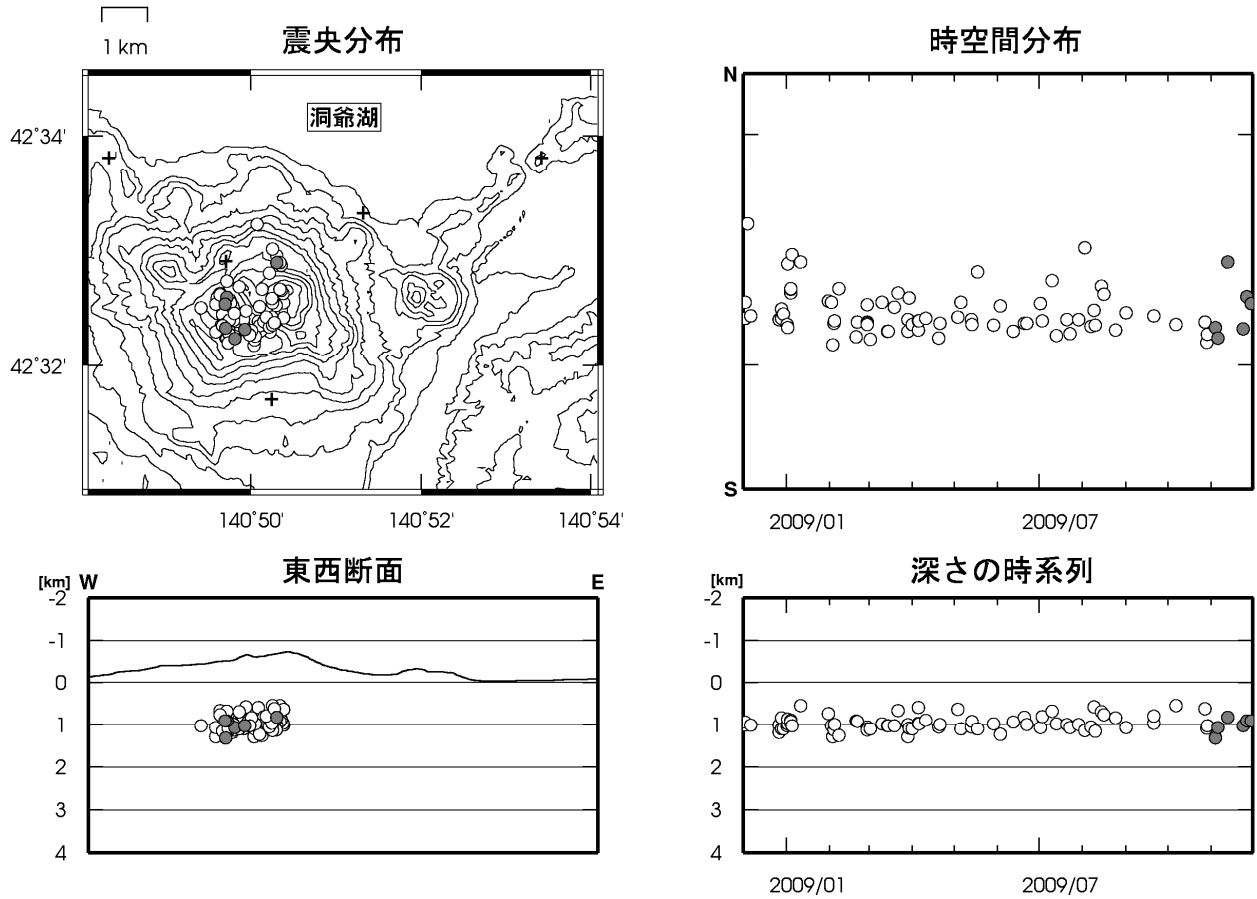
図 7 有珠山 震源分布図（2008 年 12 月～2009 年 11 月、+は地震観測点）
