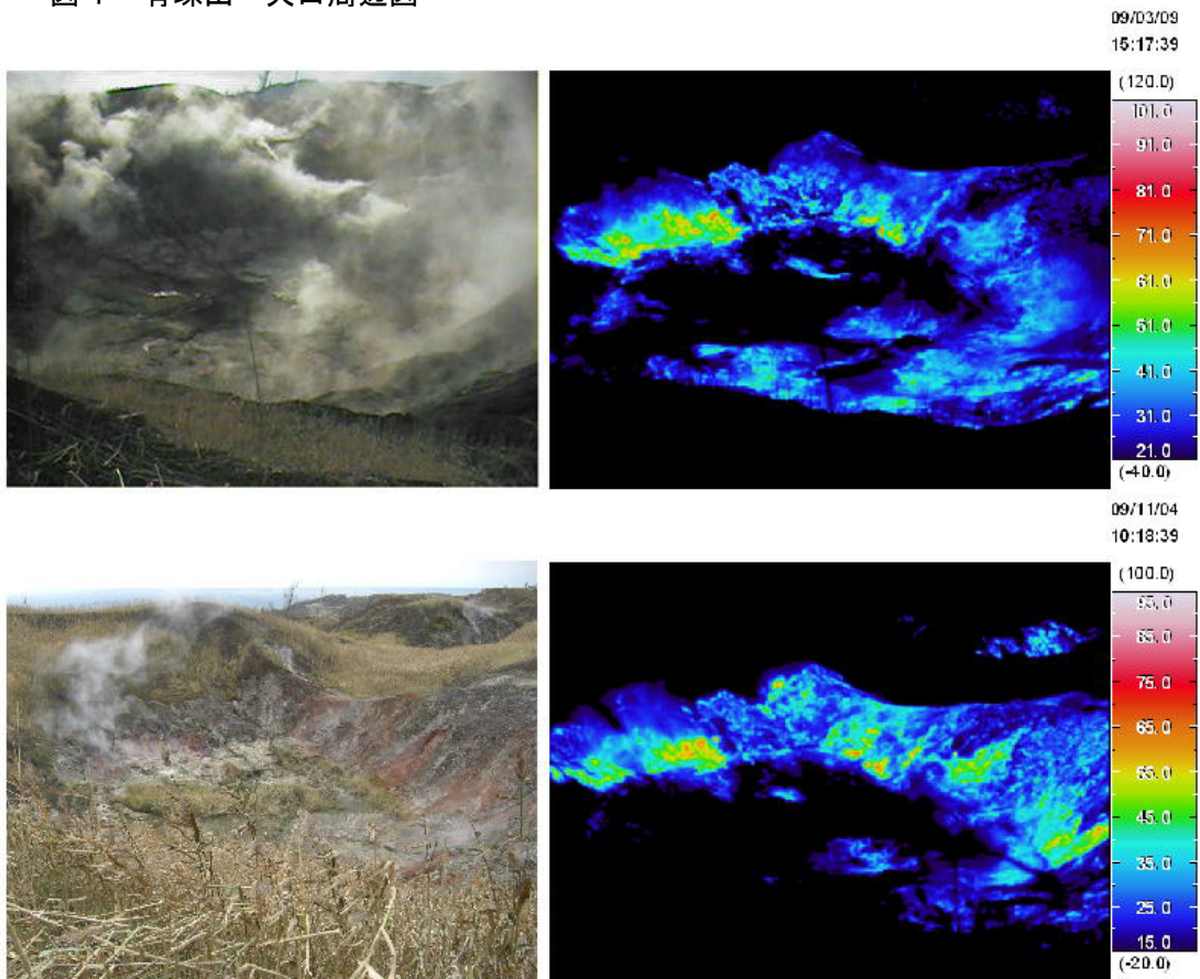
図 5 有珠山 赤外熱映像装置 1) による N-B 火口内部の地表面温度分布 (上段: 2009 年 3 月 9 日 下段: 2009 年 11 月 4 日 図 4 の①より撮影)
