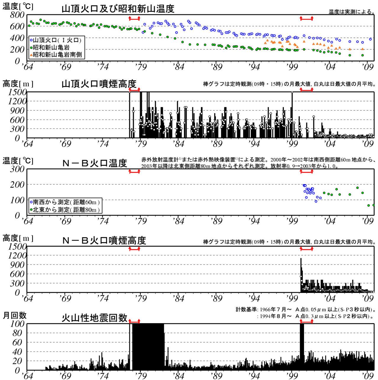
図2 有珠山 長期の火山活動経過図 (1964年1月～2009年11月)
