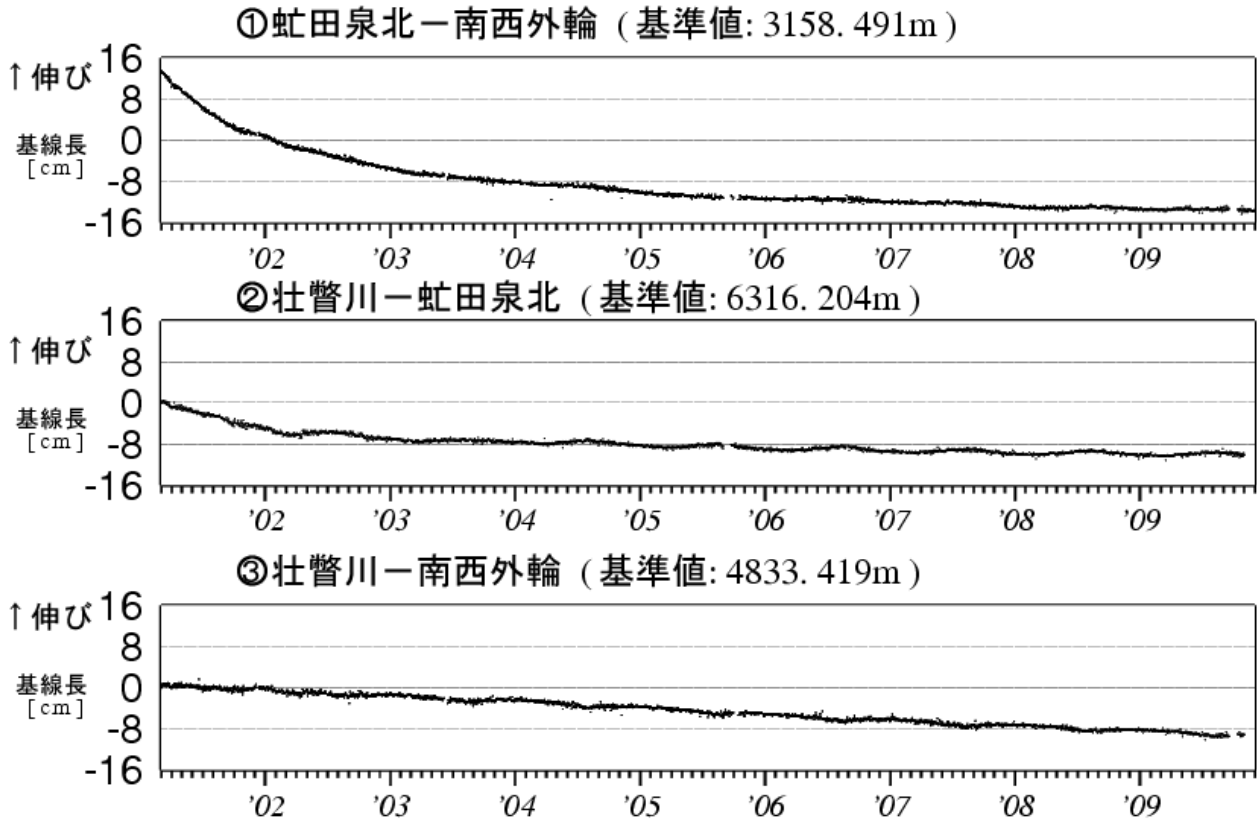
図 8 有珠山 GPS 連続観測による基線長変化（2001 年 3 月～2009 年 11 月） グラフの空白部分は欠測 図 8 の①～③は、図 9 の GPS 基線①～③に対応しています。
