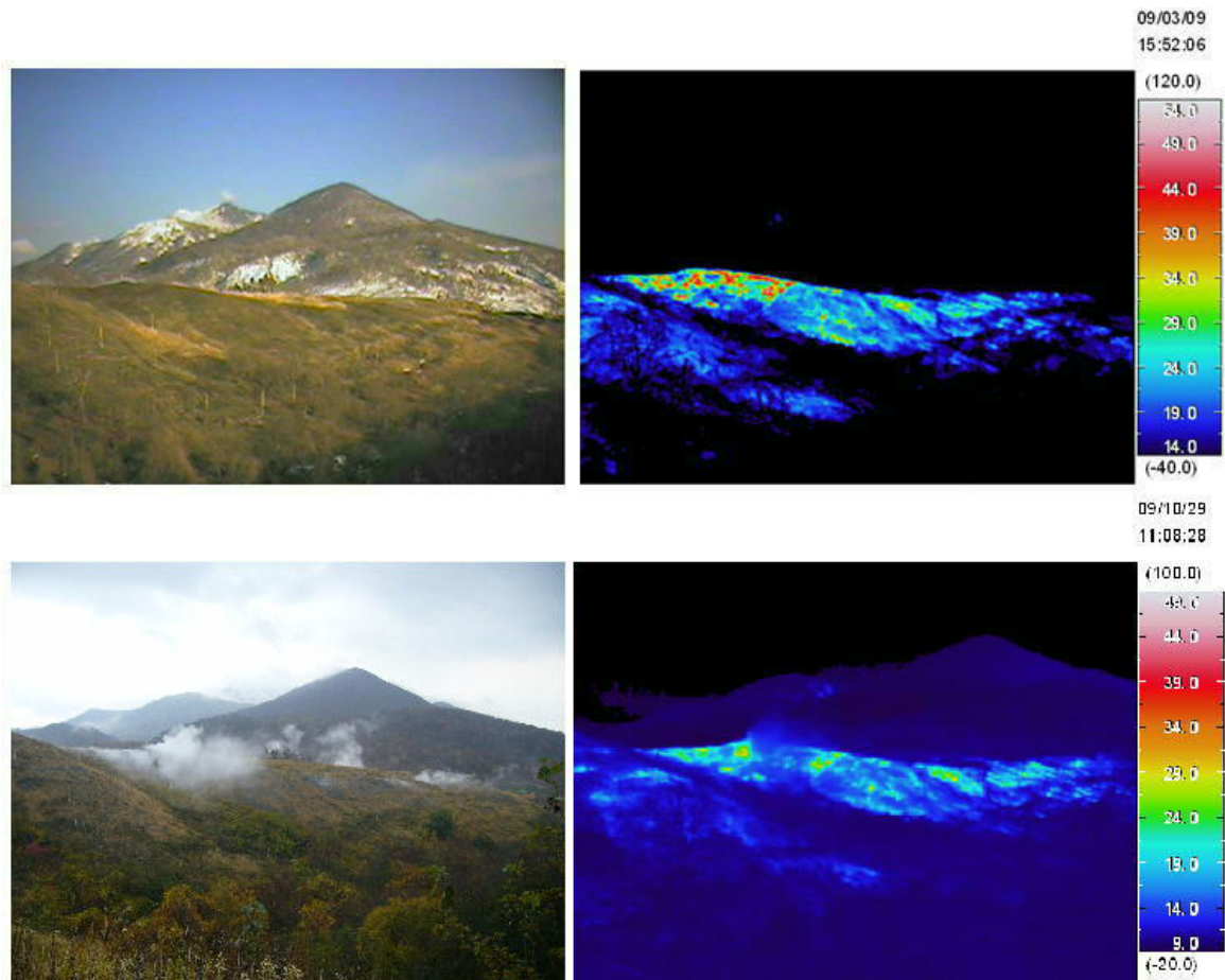
図6 有珠山 赤外熱映像装置 1) によるN-B火口北西側地熱域の地表面温度分布 (上段：2009年3月9日 下段：2009年10月29日 図4の②より撮影)
