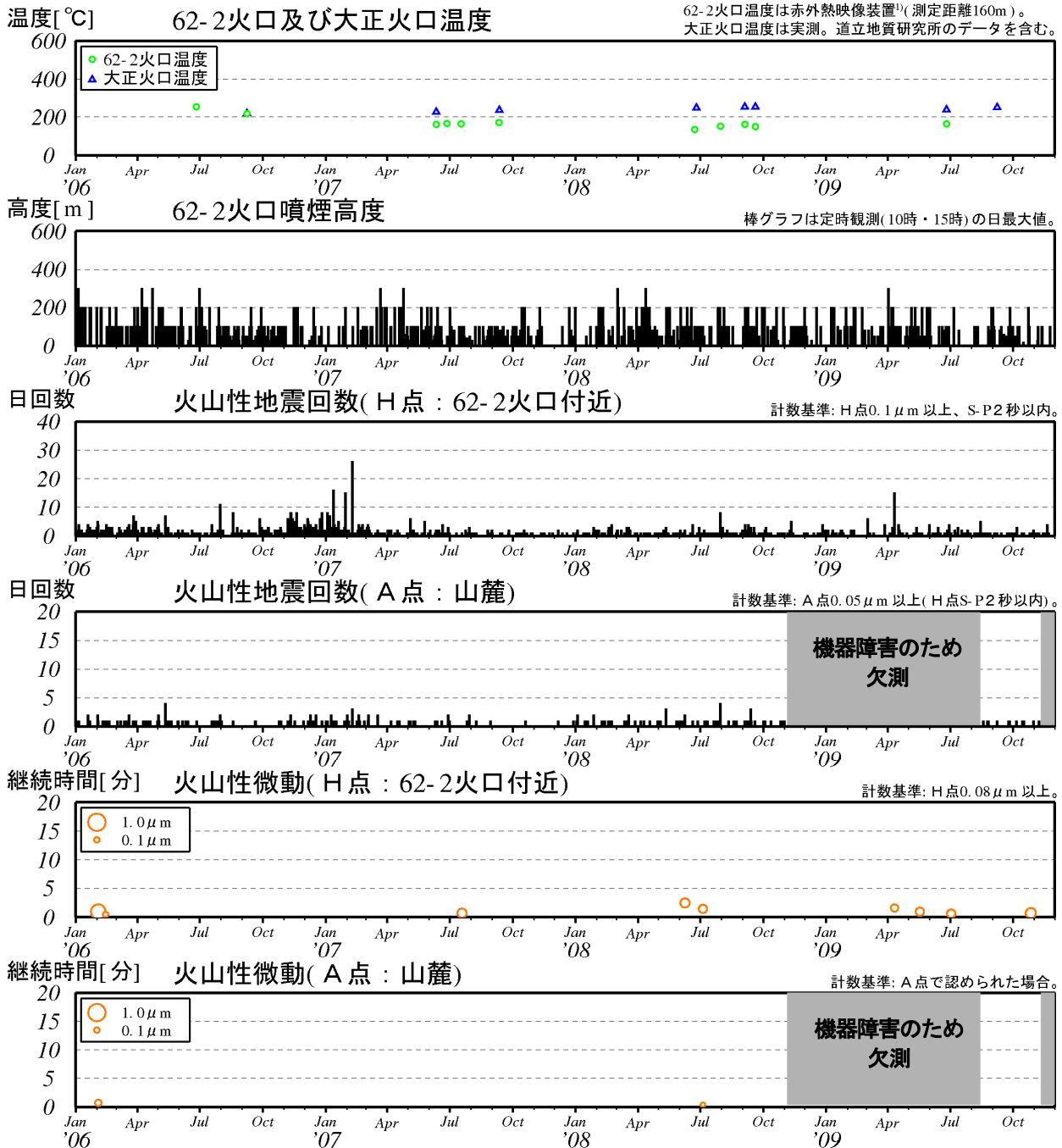
図3※ 十勝岳 最近の火山活動経過図 (2006年1月～2009年11月)
