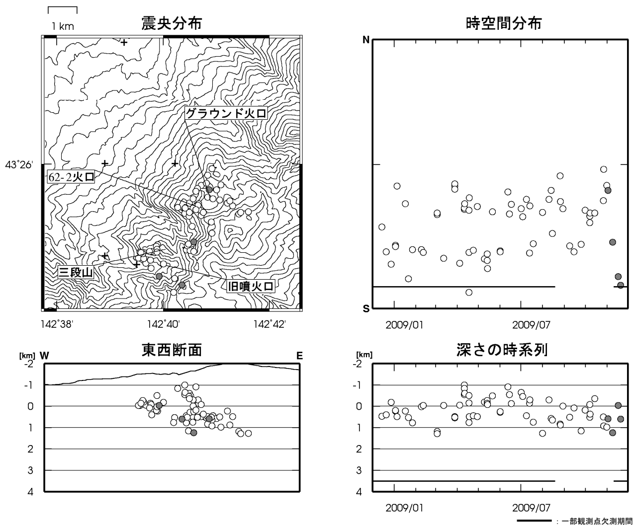
図 4※ 十勝岳 震源分布図 (2008年12月~2009年11月、+は地震観測点)
