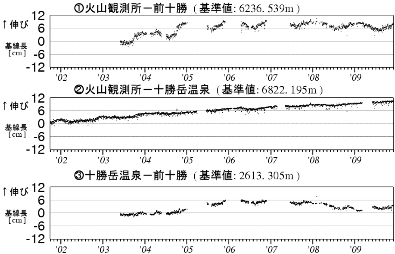
図5※ 十勝岳 GPS 連続観測による基線長変化 (2001 年 10 月～2009 年 11 月) グラフの空白部分は欠測。
