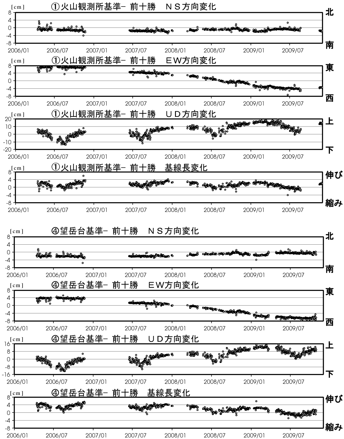
図7※ 十勝岳 GPS 連続観測による成分変化 (2006 年 1 月～2009 年 11 月) 図7は、図6の GPS 基線①、④に対応しています。火山観測所及び望岳台を基準として、 前十勝の変化を示しています。 UD方向のみスケールが異なっています。
