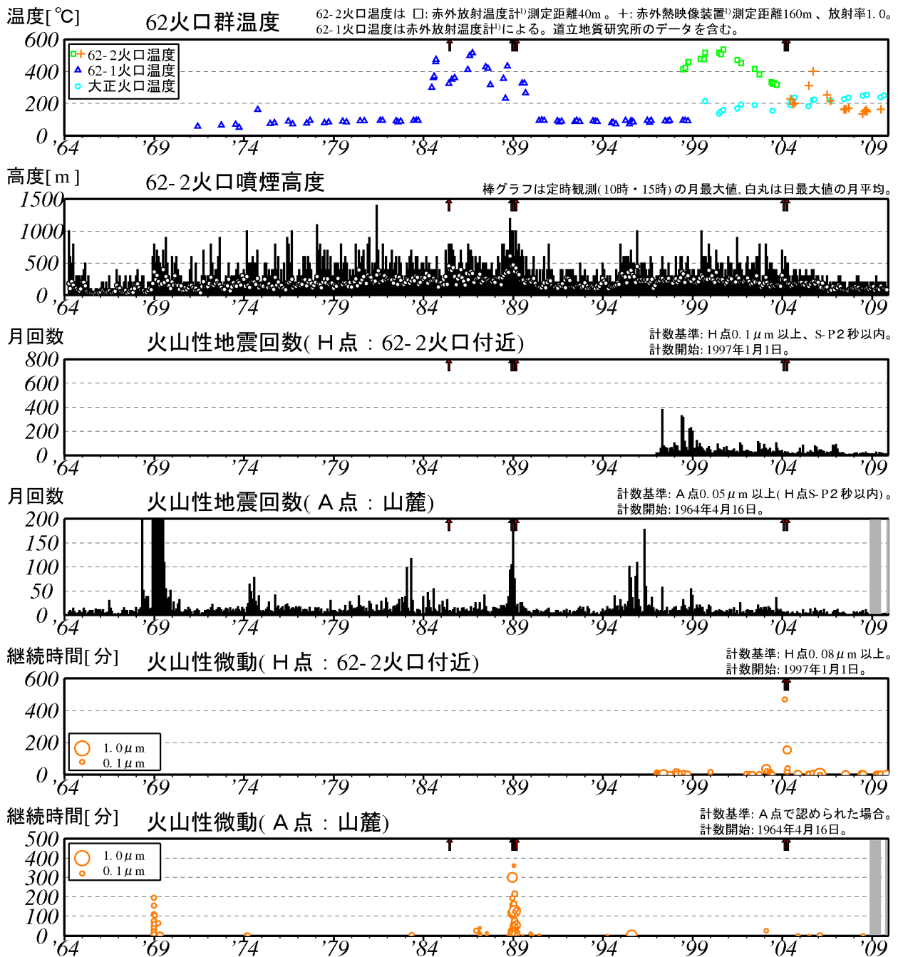
図 2※ 十勝岳 長期の火山活動経過図 (1964 年 1 月～2009 年 11 月)
