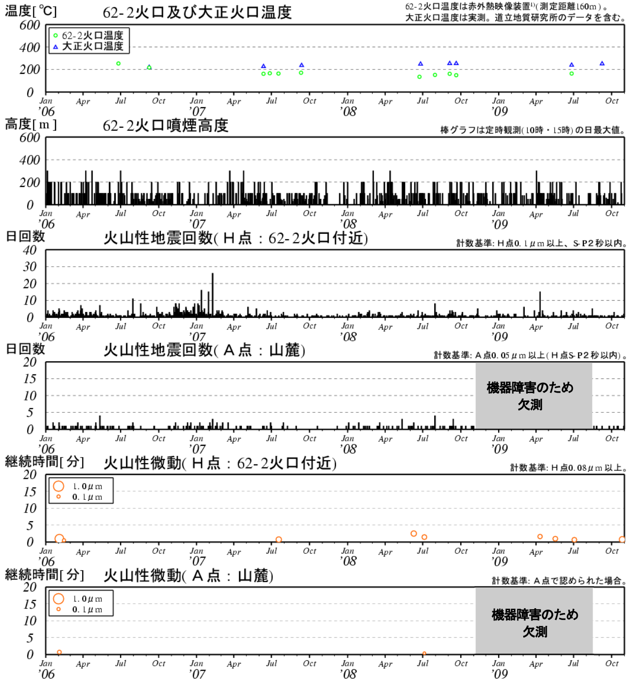
図3※ 十勝岳 最近の火山活動経過図（2006年1月～2009年10月） （A点の地震計は機器障害のため2009年8月19日から希望橋で代替観測しています）
