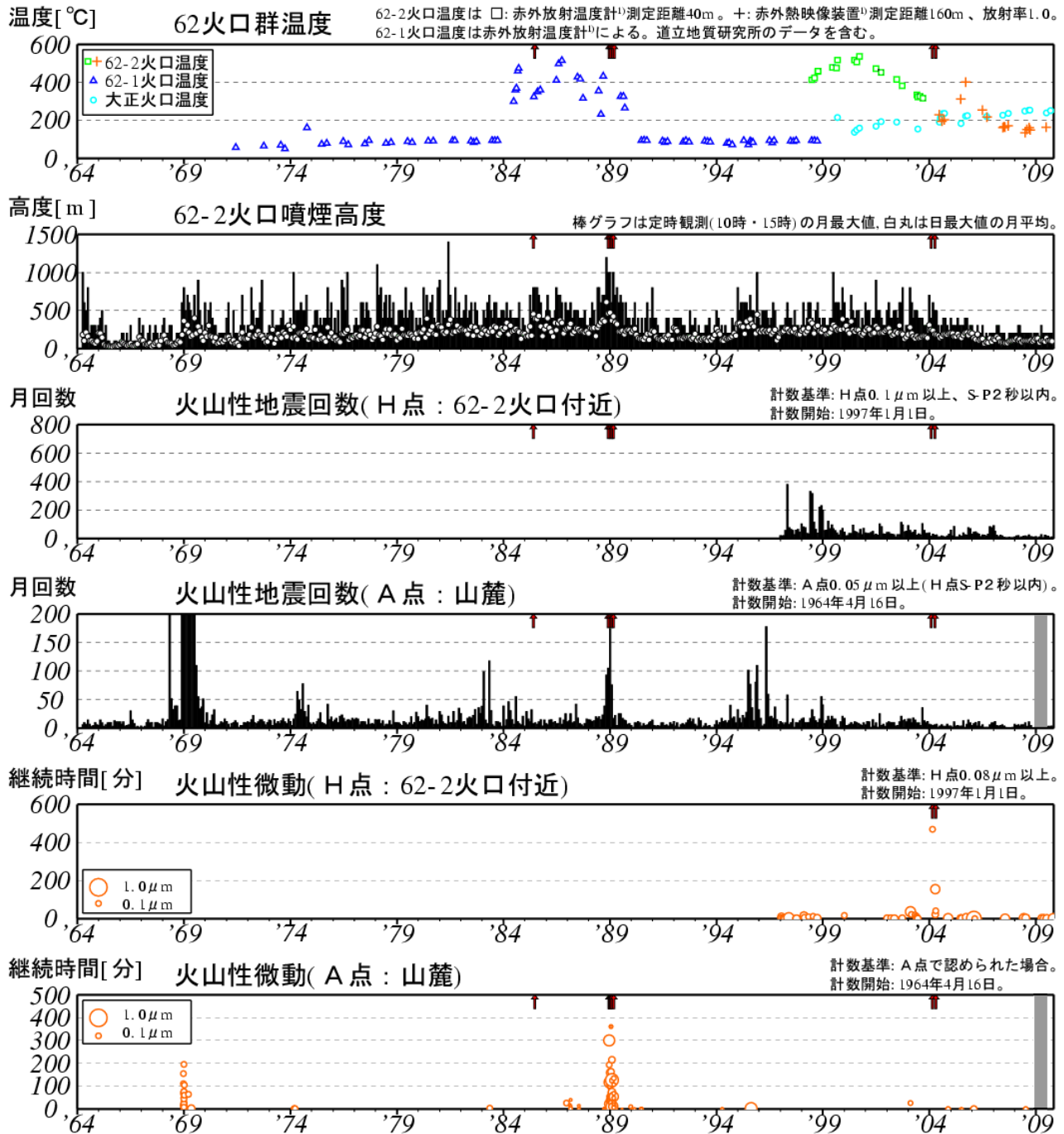
図 2※ 十勝岳 長期の火山活動経過図（1964 年 1 月～2009 年 10 月）
