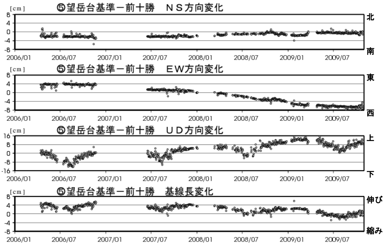
図 6※ 十勝岳 GPS 連続観測による成分変化（2006 年 1 月～2009 年 10 月）
