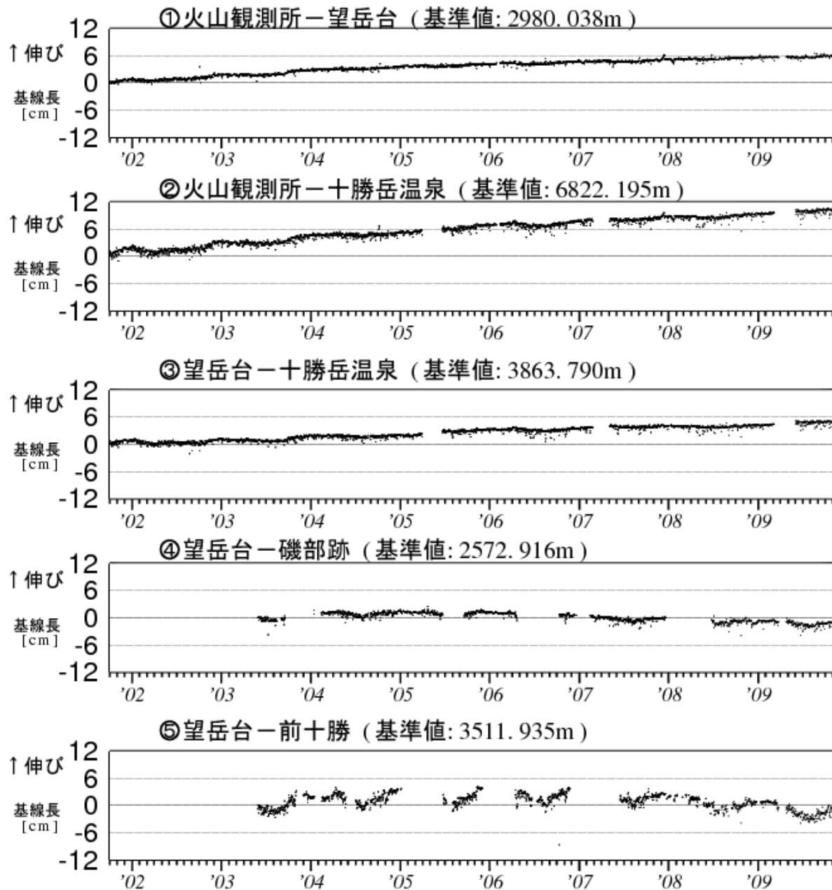
図5※ 十勝岳 GPS 連続観測による基線長変化（2001 年 10 月～2009 年 10 月） グラフの空白部分は欠測。
