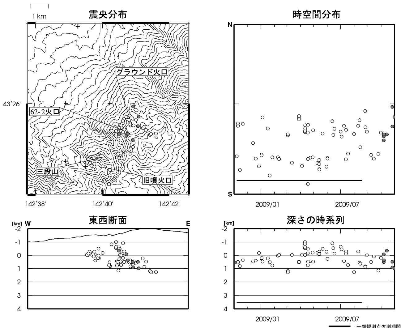
図 4 ※ 十勝岳 震源分布図（2008 年 11 月～2009 年 10 月、+は地震観測点）
