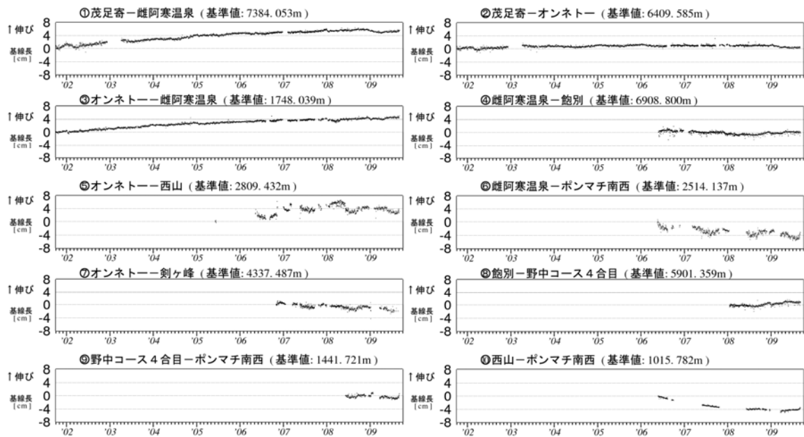
図3※ 雌阿寒岳 GPS 連続観測による基線長変化 (2001 年 10 月 1 日～2009 年 9 月 7 日) ・ 火山活動によると考えられる変動は観測されていません。
