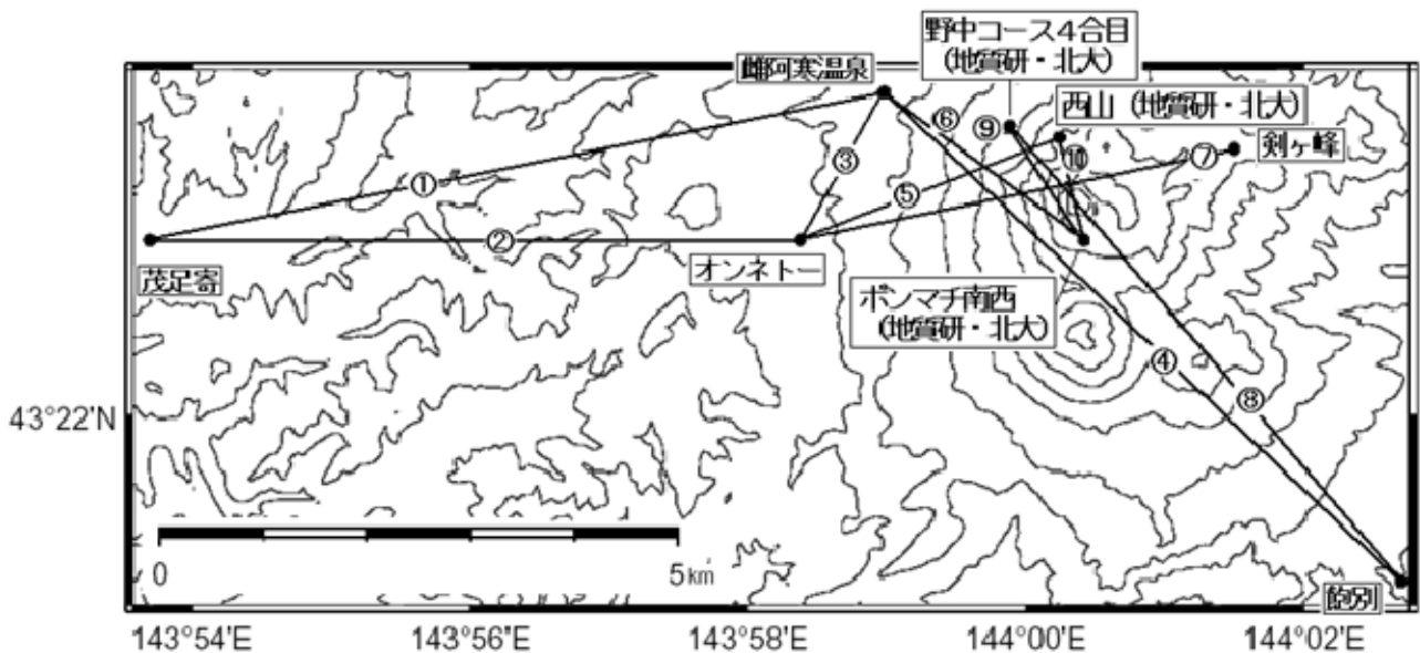
図4 雌阿寒岳 GPS 連続観測点配置図
