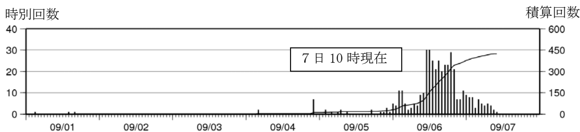
図 1 雌阿寒岳 火山性地震の時間別回数及び積算回数（2009 年 9 月 1 日～9 月 7 日）
