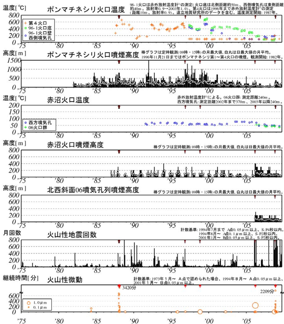
図 5 雌阿寒岳の火山活動経過図
