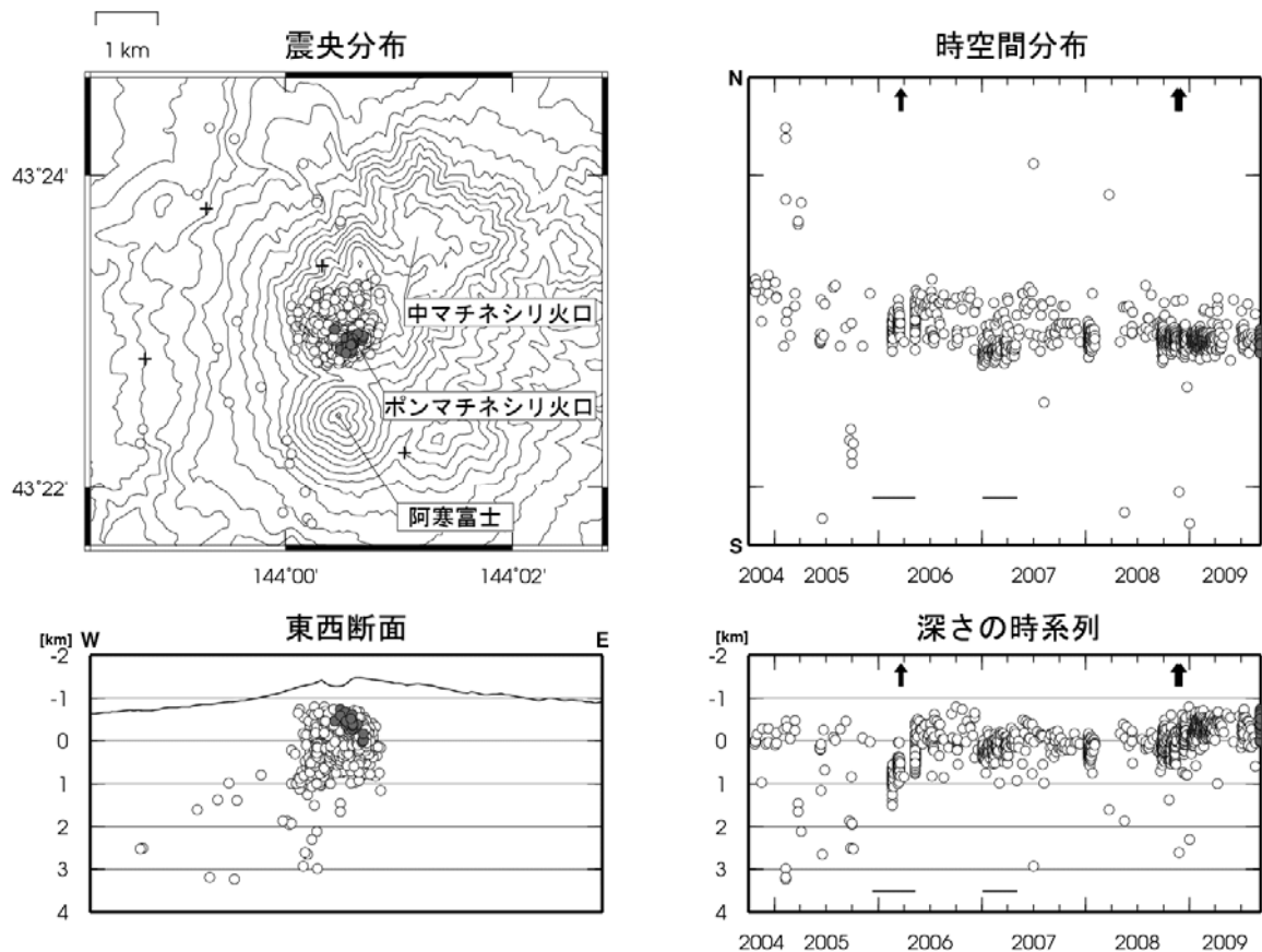
図 2 雌阿寒岳 火山性地震の震源分布（2004 年 10 月 1 日～2009 年 9 月 7 日 10 時現在） （丸印：震源、+印：地震観測点 ↑印は噴火を示す）
