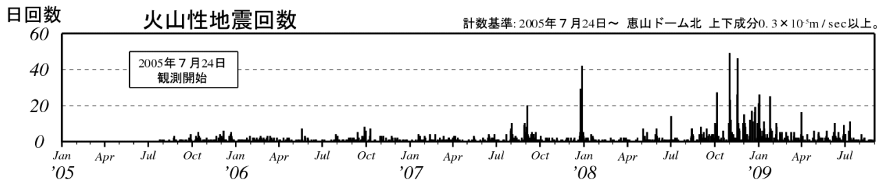
図 2 恵山 日別地震回数（2005 年 7 月～2009 年 8 月）
