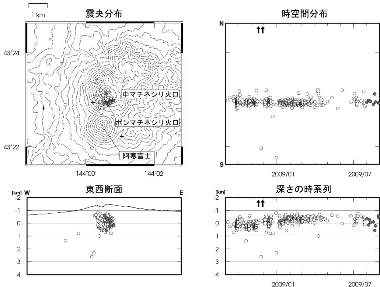
図 5 雌阿寒岳 震源分布図(2008 年 9 月～2009 年 8 月) +は地震観測点 ↑印は噴火
