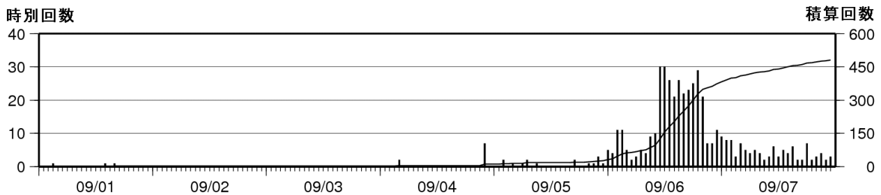
図 4 雌阿寒岳 火山性地震の時間別回数及び積算回数 (2009 年 9 月 1 日～9 月 7 日)
