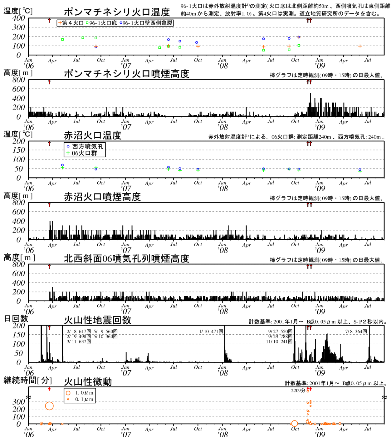
図3※ 雌阿寒岳 最近の火山活動経過図（2006年1月～2009年8月） ↑印は噴火
