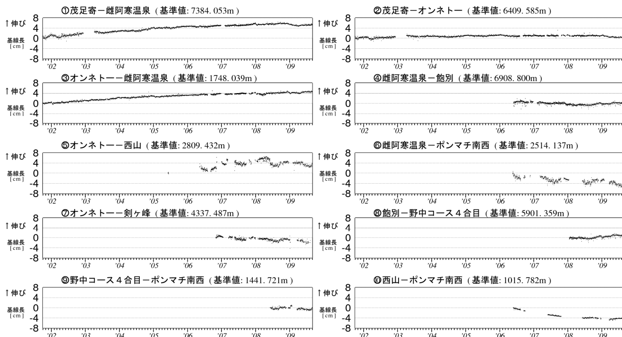
図 6※ 雌阿寒岳 GPS 連続観測による基線長変化（2001 年 10 月～2009 年 8 月） グラフの空白部分は欠測 図 6 の①～⑩は、図 7 の GPS 基線①～⑩に対応しています。
