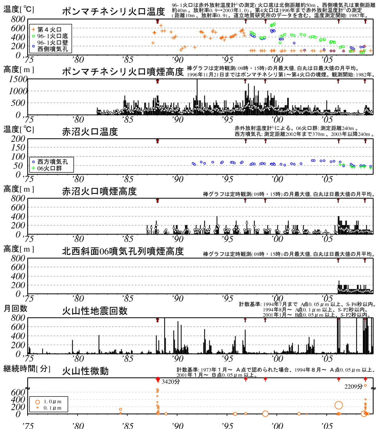
図2※ 雌阿寒岳 長期の火山活動経過図(1975年1月～2009年8月) ↑印は噴火 (1988年、1996年、1998年、2008年: ポンマチネシリ火口からの噴火、2006年: 赤沼火口からの噴火)
