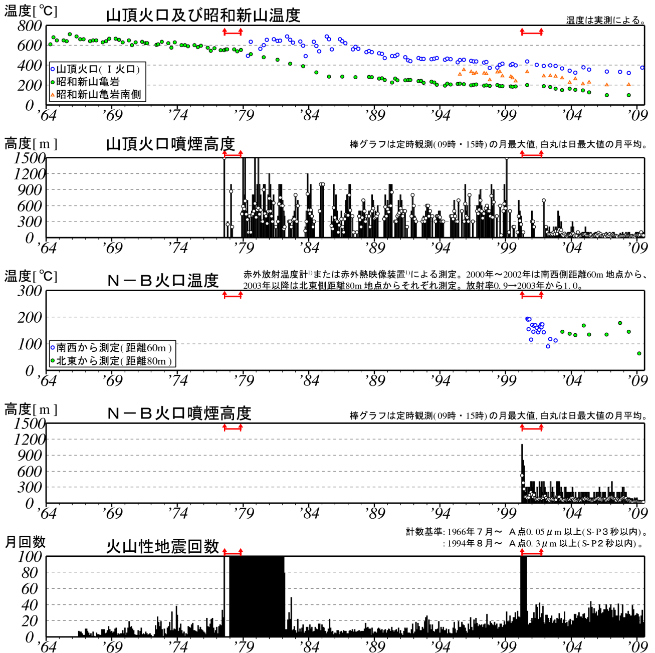
図 2 有珠山 長期の火山活動経過図（1964 年 1 月～2009 年 7 月）
