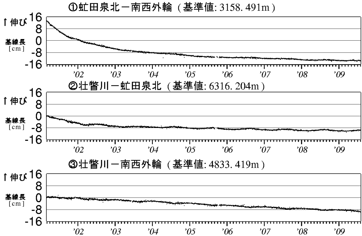
図5 有珠山 GPS 連続観測による基線長変化（2001年3月～2009年7月） グラフの空白部分は欠測 図5の①～③は、図6のGPS基線①～③に対応しています。
