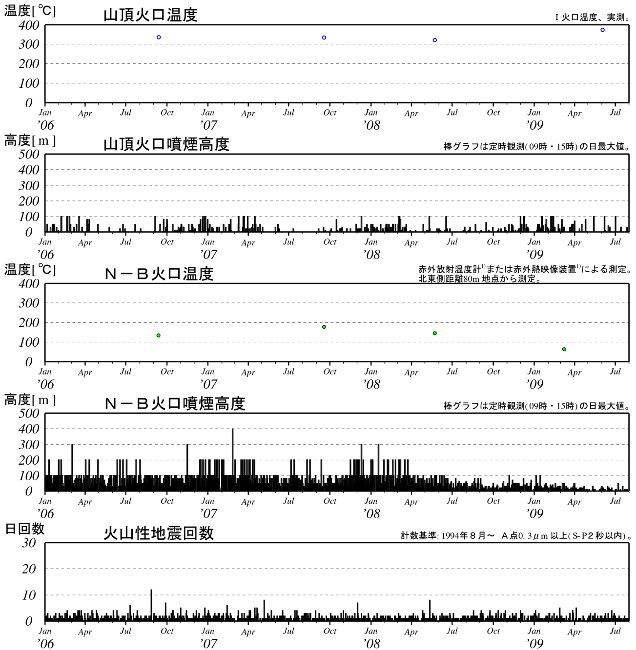
図3 有珠山 最近の火山活動経過図（2006年1月～2009年7月）
