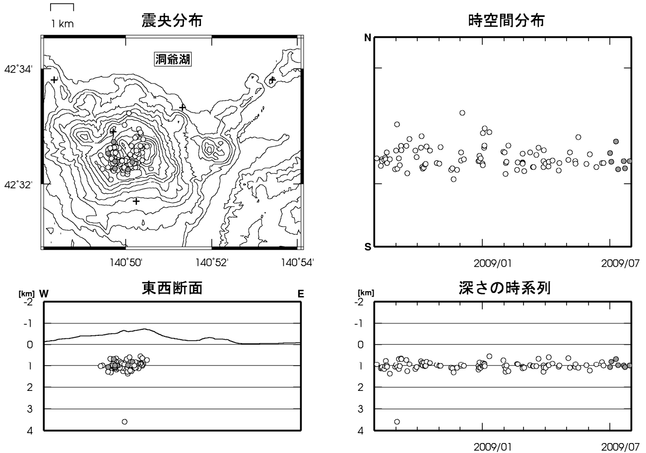
図 4 有珠山 震源分布図（2008 年 8 月～2009 年 7 月、+は地震観測点）
