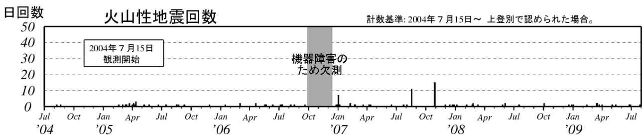
図 2 倶多楽 日別地震回数（2004 年 7 月～2009 年 7 月）
