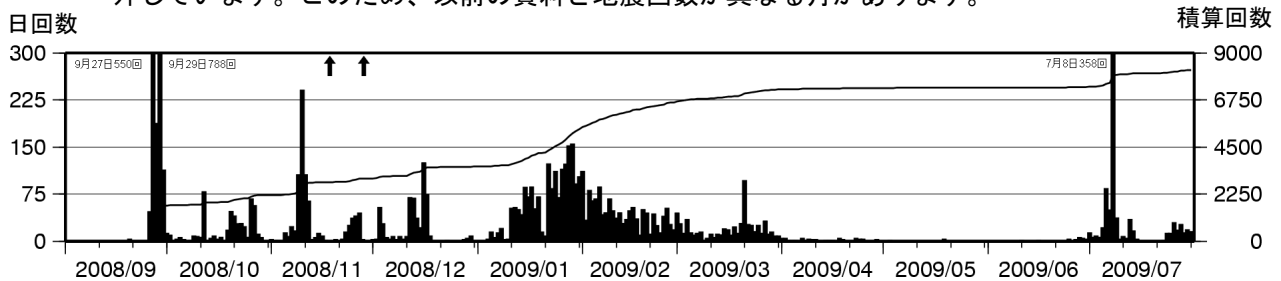
図 6 雌阿寒岳 地震活動推移（2008 年 9 月 1 日～2009 年 7 月 31 日）↑印は噴火 棒グラフは日別回数、折れ線グラフは積算回数
