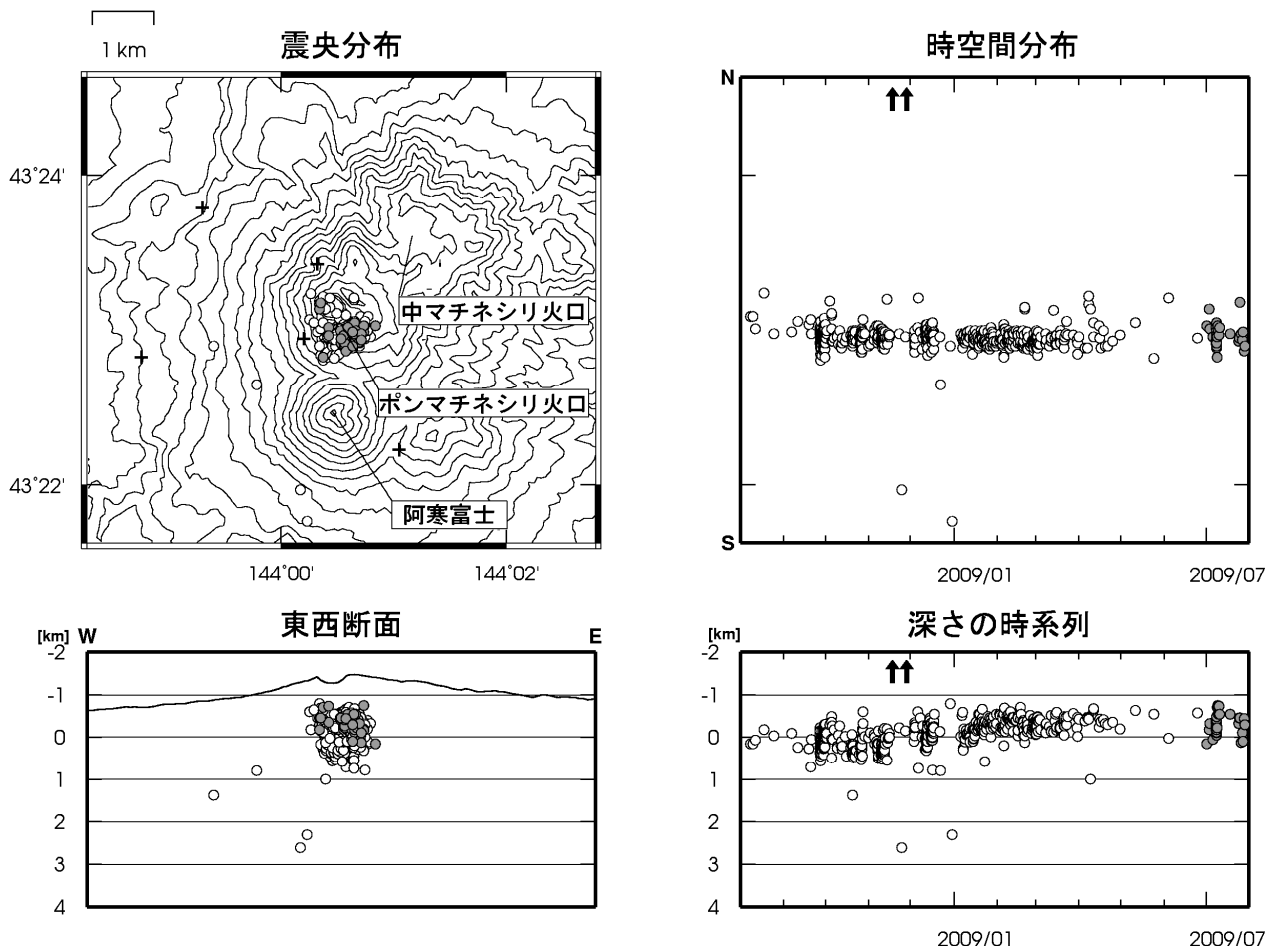
図 7 雌阿寒岳 震源分布図（2008 年 8 月～2009 年 7 月）＋は地震観測点 ↑印は噴火
