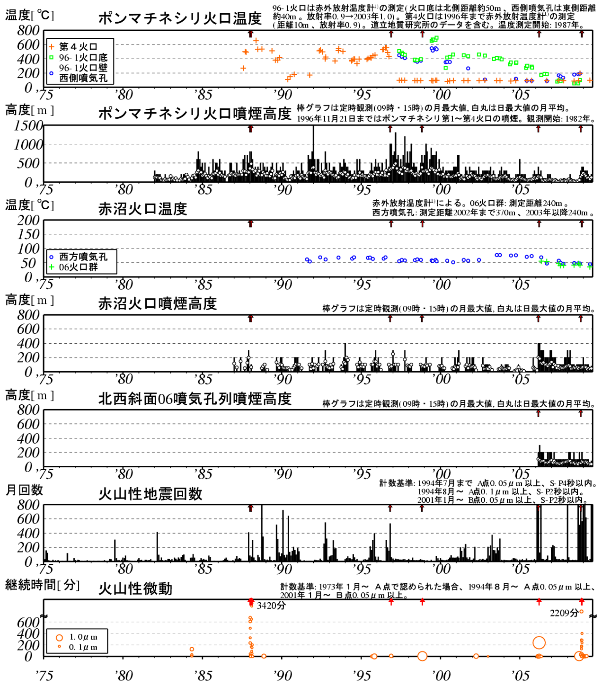
図2※ 雌阿寒岳 長期の火山活動経過図(1975年1月～2009年7月) ↑印は噴火 (1988年、1996年、1998年、2008年: ポンマチネシリ火口からの噴火、2006年: 赤沼火口からの噴火)
