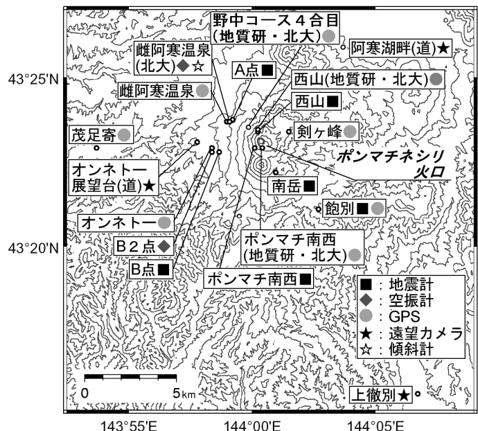
図 1 雌阿寒岳 火山観測点配置図
