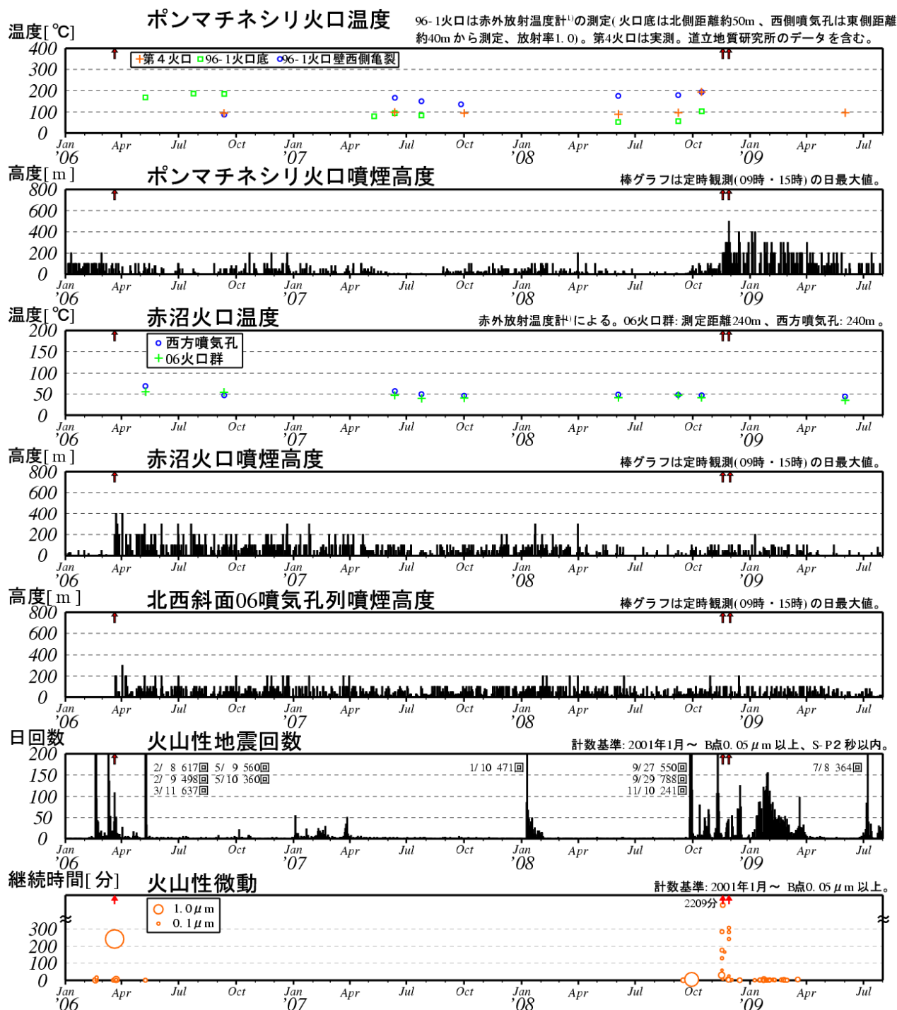
図 3※ 雌阿寒岳 最近の火山活動経過図（2006 年 1 月～2009 年 7 月） ↑印は噴火
