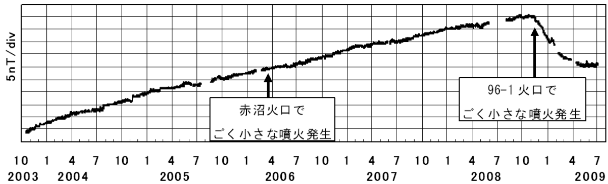
図4 雌阿寒岳 全磁力連続観測結果 図5のMEA(◎)にて測定(2003年10月~2009年7月3日) 地磁気観測所女満別出張所を基準とし広域的変動を除去した残差
