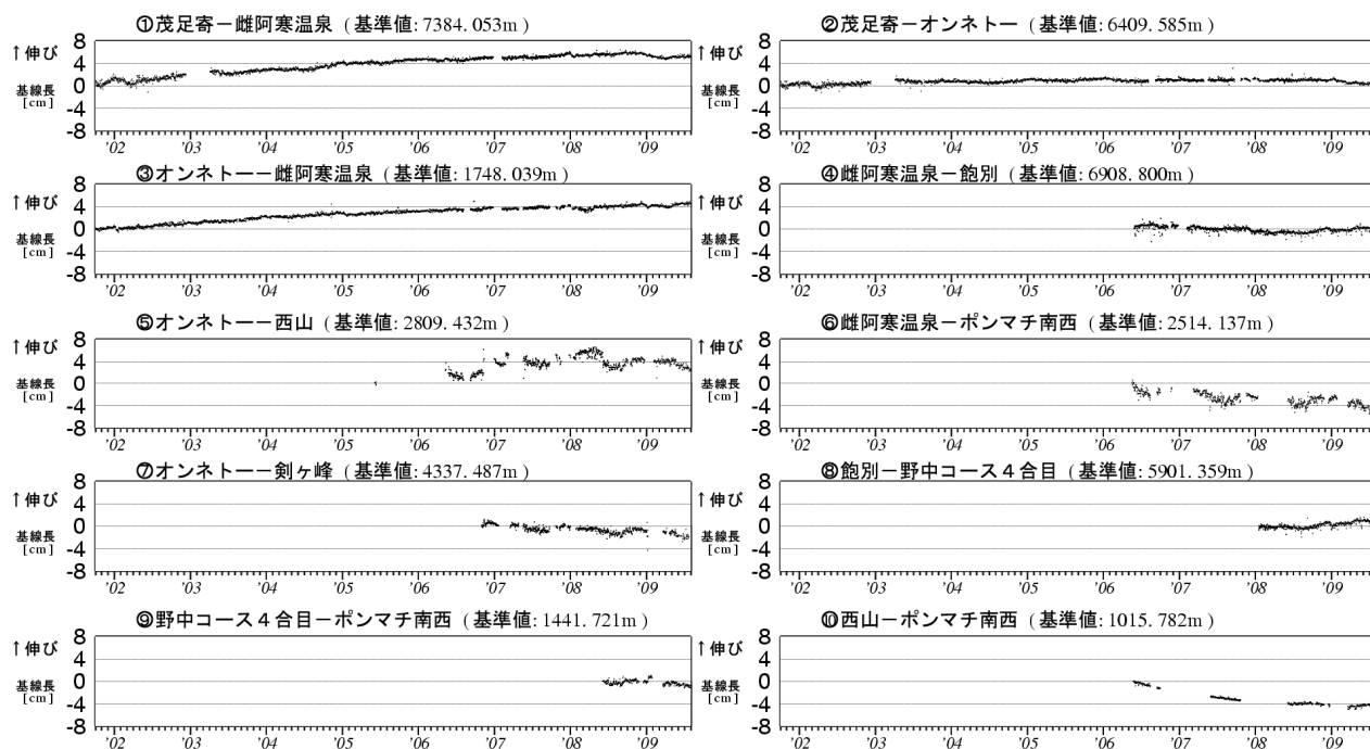
図 8※ 雌阿寒岳 GPS 連続観測による基線長変化（2001 年 10 月～2009 年 7 月）
