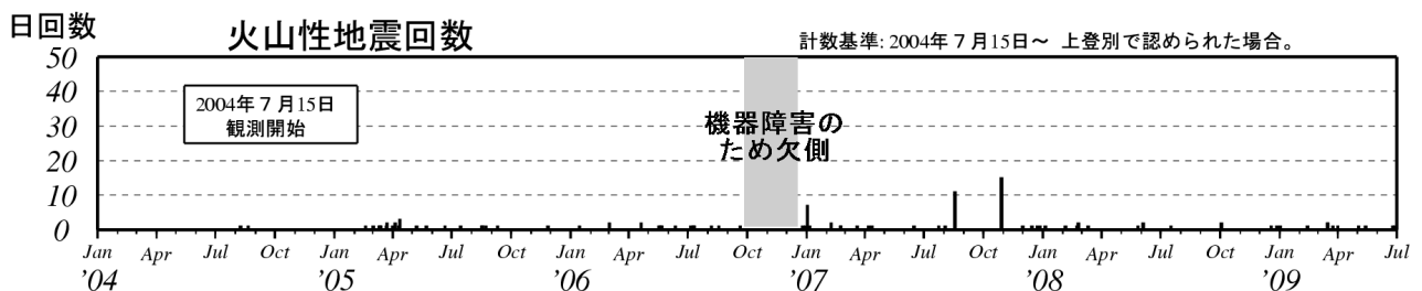
図 2 倶多楽 日別地震回数（2004 年 7 月～2009 年 6 月）
