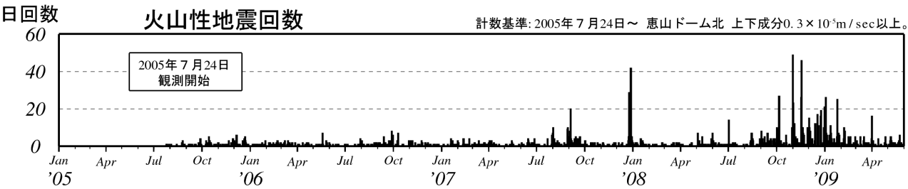
図 2 恵山 日別地震回数（2005 年 7 月～2009 年 5 月）
