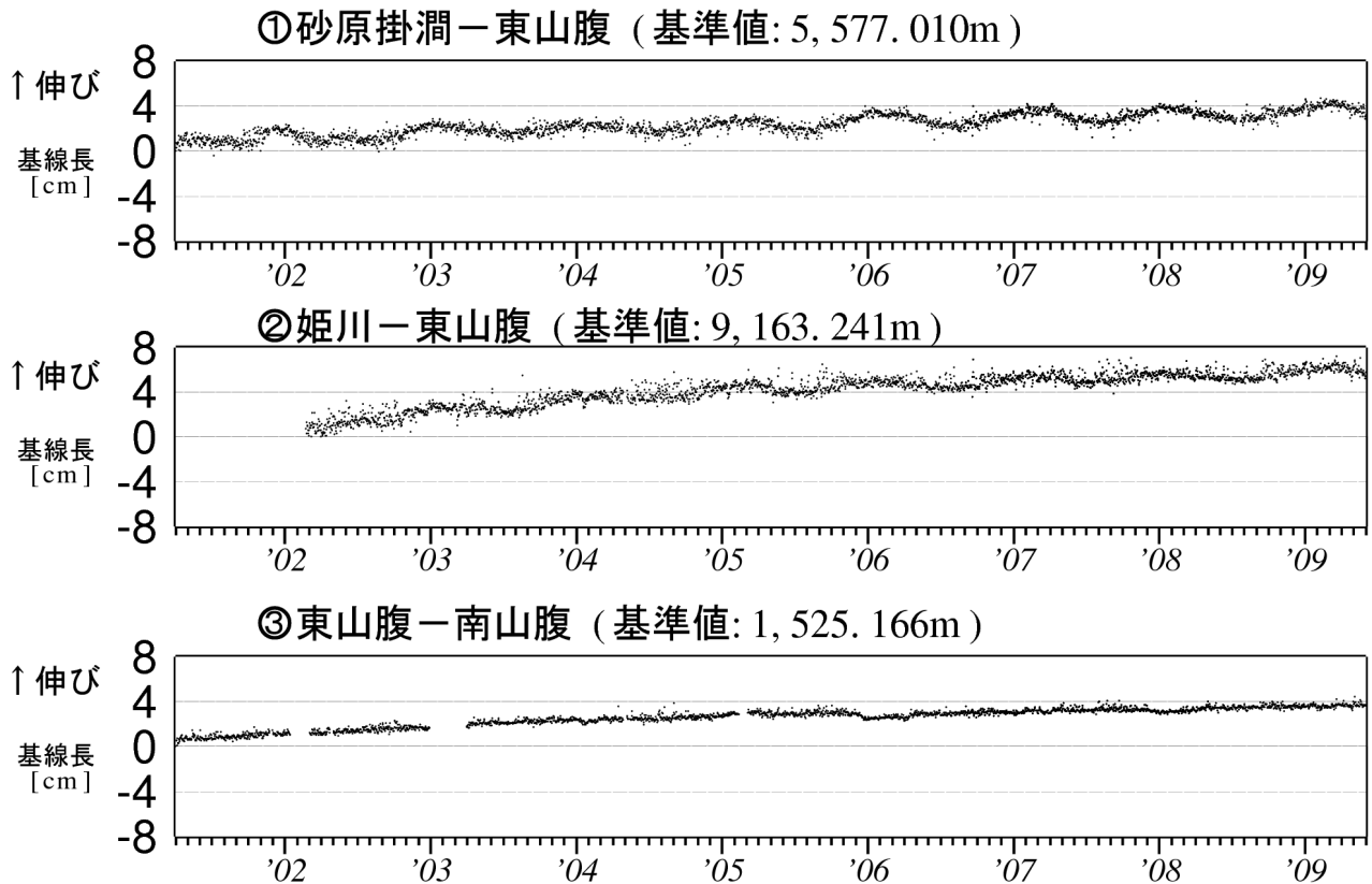
図 5 北海道駒ヶ岳 GPS 連続観測による基線長変化（2001 年 4 月～2009 年 5 月）
