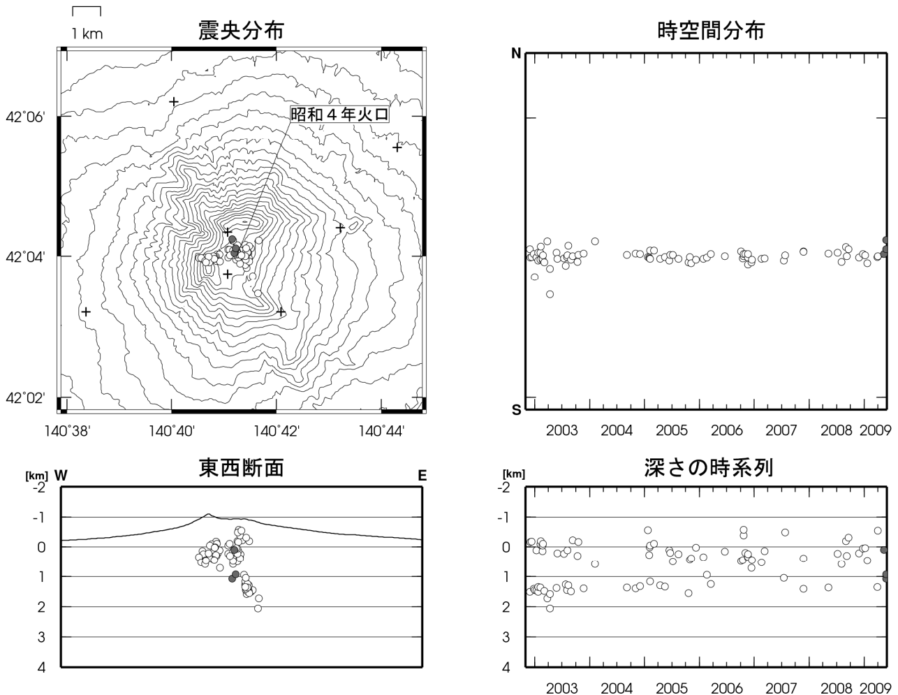
図 4 ※ 北海道駒ヶ岳 震源分布図（2002 年 11 月～2009 年 5 月、+は地震観測点）
