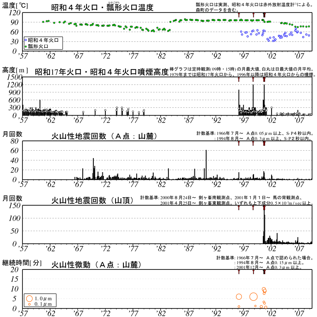
図 2※ 北海道駒ヶ岳 長期の火山活動経過図（1957 年 1 月～2009 年 5 月）↑印は噴火
