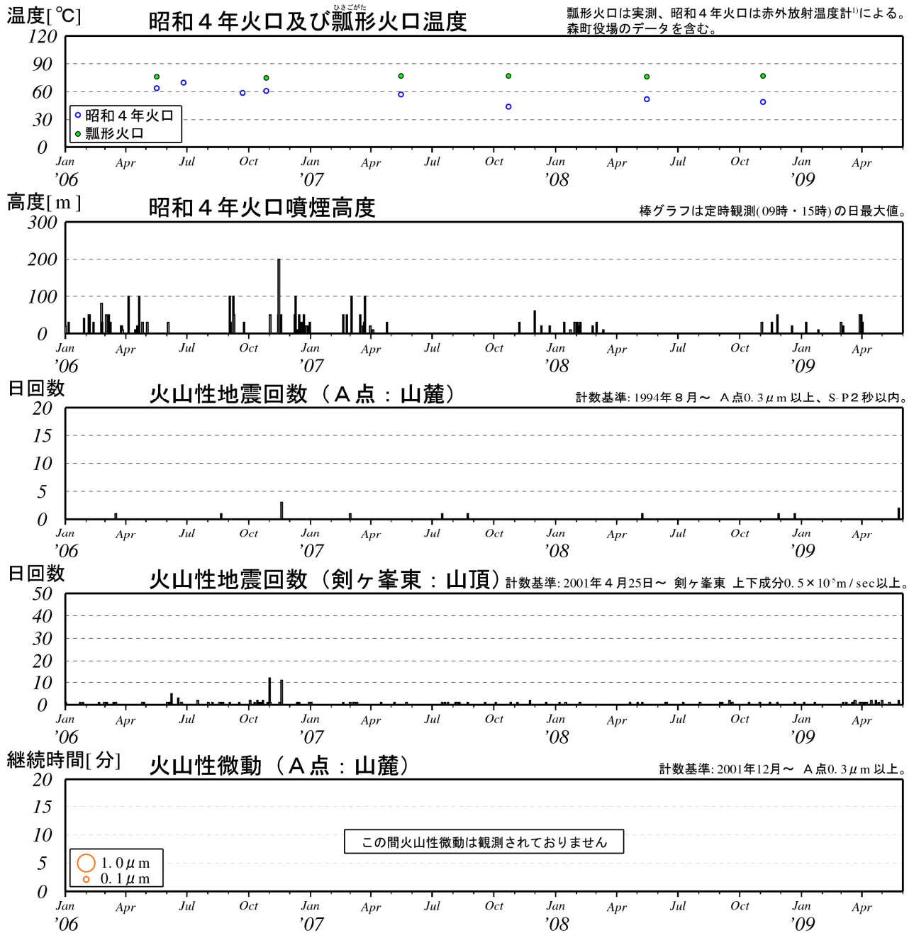
図 3※ 北海道駒ヶ岳 最近の火山活動経過図（2006 年 1 月～2009 年 5 月）
