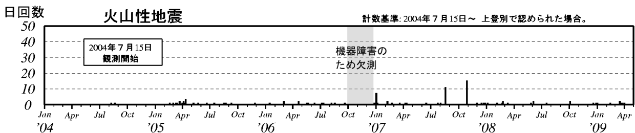
図 2 倶多楽 日別地震回数（2004 年 7 月～2009 年 4 月）
