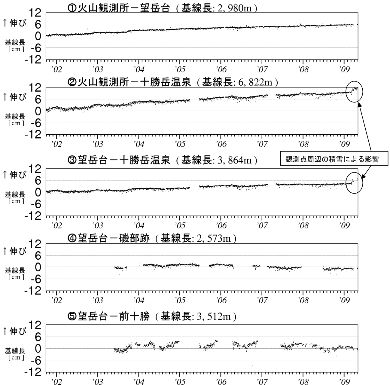
図 9※ 十勝岳 GPS 連続観測による基線長変化（2001 年 10 月～2009 年 4 月） グラフの空白部分は欠測。
