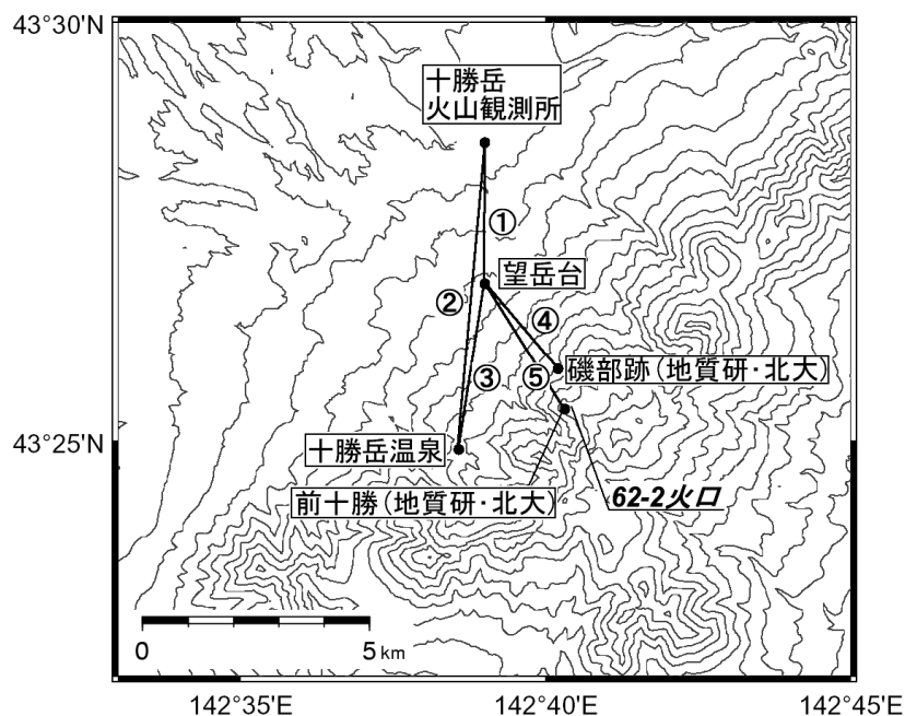
図 11※ 十勝岳 GPS 観測点配置図
