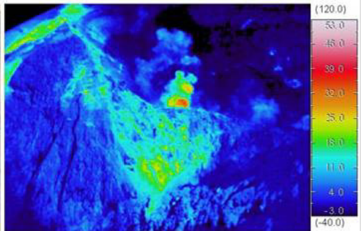
図 6 十勝岳 赤外熱映像装置 1) による 62 火口群の地表面温度分布 (図 4 矢印方向より撮影) 2009 年 4 月 17 日北海道開発局の協力による
