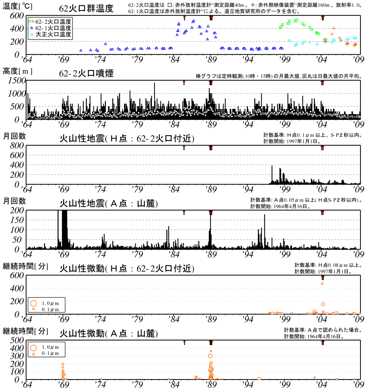
図 2 ※ 十勝岳 長期の火山活動経過図（1964 年 1 月～2009 年 4 月）
