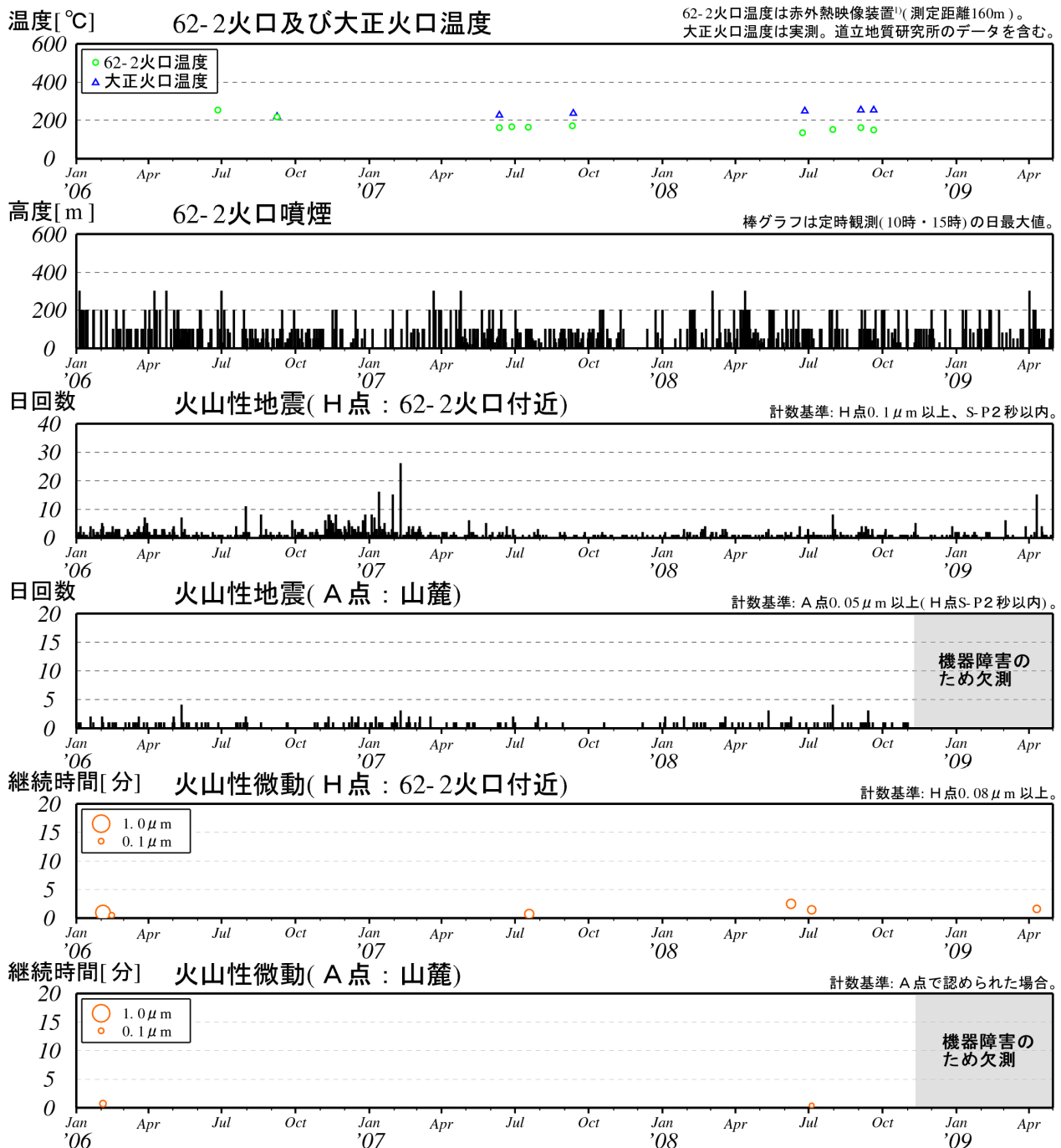
図3※ 十勝岳 最近の火山活動経過図（2006年1月～2009年4月） （A点の地震計は機器障害のため2008年11月7日から欠測しています）
