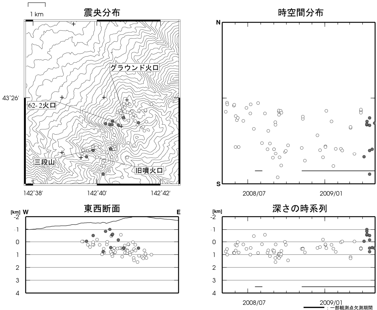
図 8※ 十勝岳 震源分布図（2008 年 5 月～2009 年 4 月、+は地震観測点）
