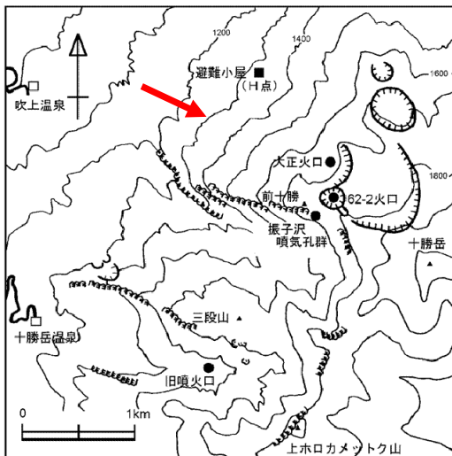
図 4 十勝岳 火口周辺図
