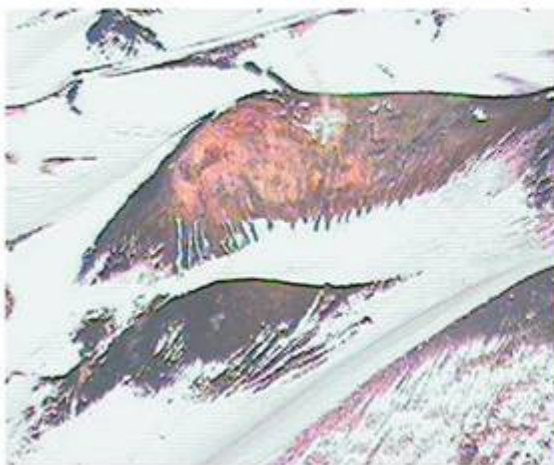
図 7 十勝岳 赤外熱映像装置 1) による大正火口の地表面温度分布 (図 4 矢印方向より撮影) 2009 年 4 月 17 日北海道開発局の協力による
