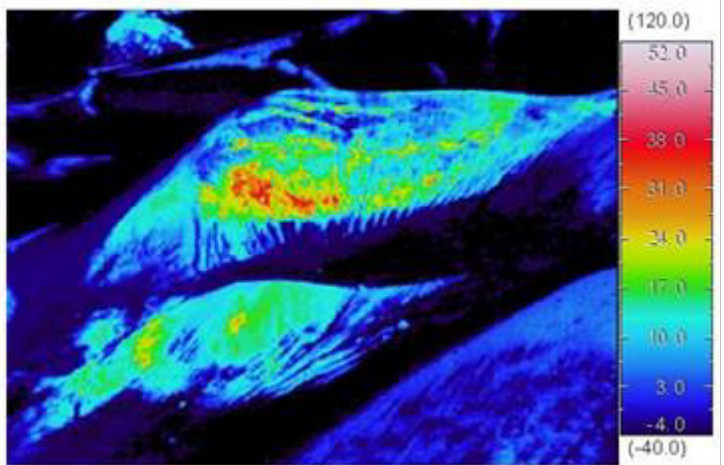
図 7 十勝岳 赤外熱映像装置 1) による大正火口の地表面温度分布 (図 4 矢印方向より撮影) 2009 年 4 月 17 日北海道開発局の協力による
