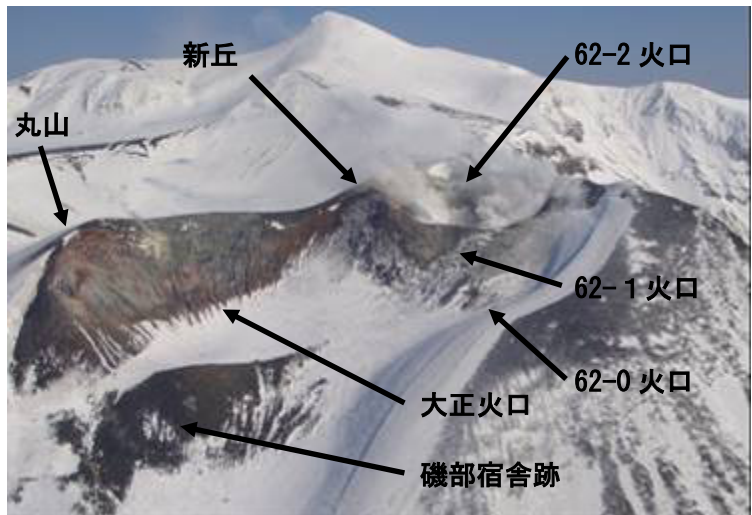
図 5 十勝岳 62 火口群・大正火口の状況
