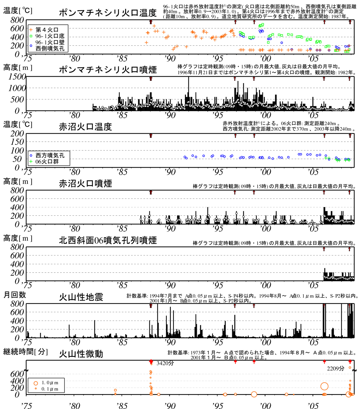
図4※ 雌阿寒岳 長期の火山活動経過図(1975年1月～2009年4月) ↑印は噴火
