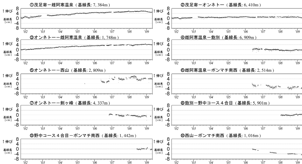
図 9 ※ 雌阿寒岳 GPS 連続観測による基線長変化（2001 年 10 月～2009 年 4 月）
