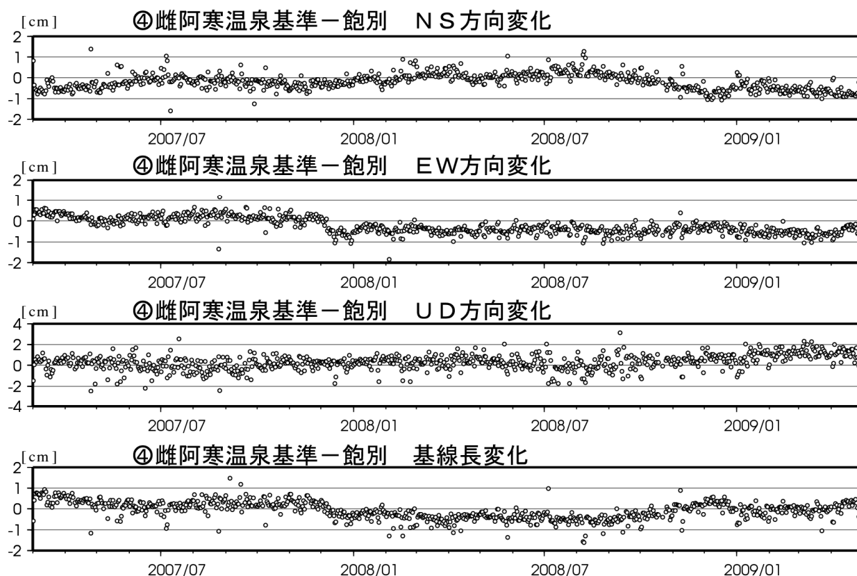
図 11 雌阿寒岳 GPS 連続観測による成分別変化（2007 年 4 月～2009 年 4 月）
