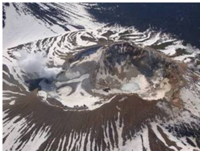
図 7 雌阿寒岳 ポンマチネシリ火口の状況
