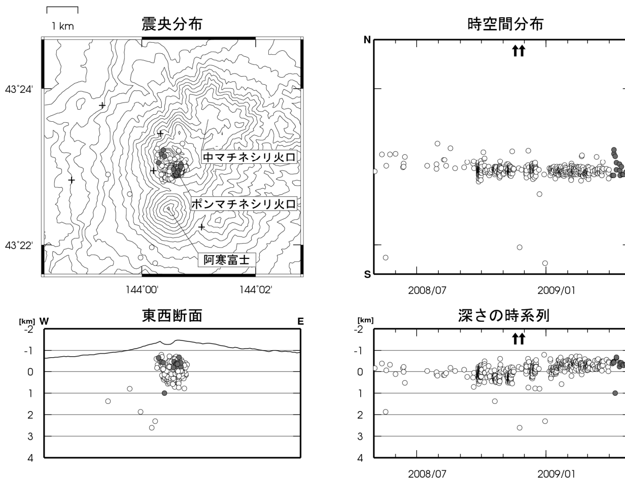
図 3 雌阿寒岳 震源分布図（2008 年 5 月～2009 年 4 月）+は地震観測点 ↑印は噴火
