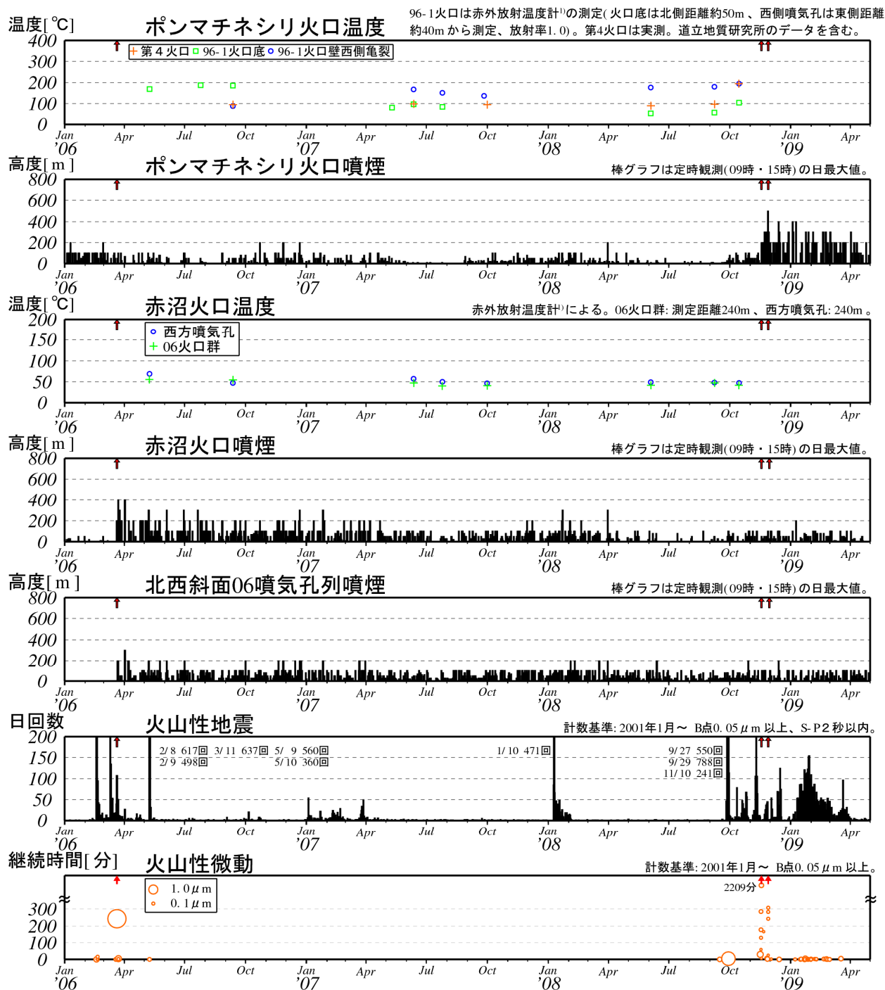
図5※ 雌阿寒岳 最近の火山活動経過図（2006年1月～2009年4月） ↑印は噴火
