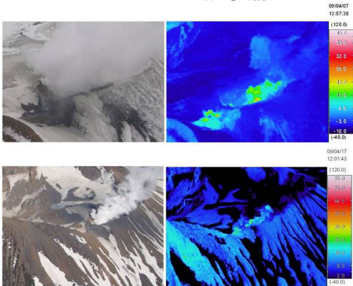
図 8 雌阿寒岳 赤外熱映像装置 1) による 96-1 火口周辺の地表面温度分布（図 6 ②より撮影）
