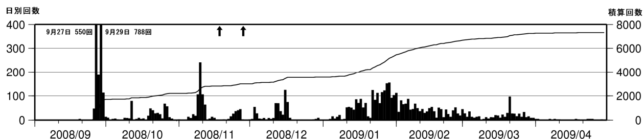
図 2 雌阿寒岳 地震活動推移（2008 年 9 月 1 日～2009 年 4 月 30 日）↑印は噴火 棒グラフは日別回数、折れ線グラフは積算回数
