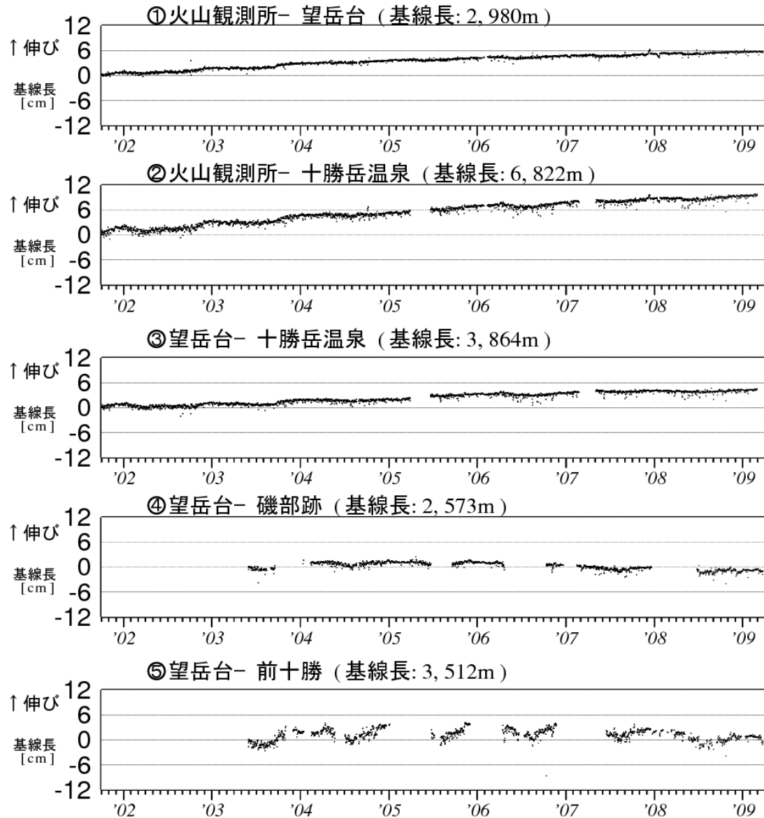
図 5※ 十勝岳 GPS 連続観測による基線長変化（2001 年 10 月～2009 年 3 月） グラフの空白部分は欠測。
