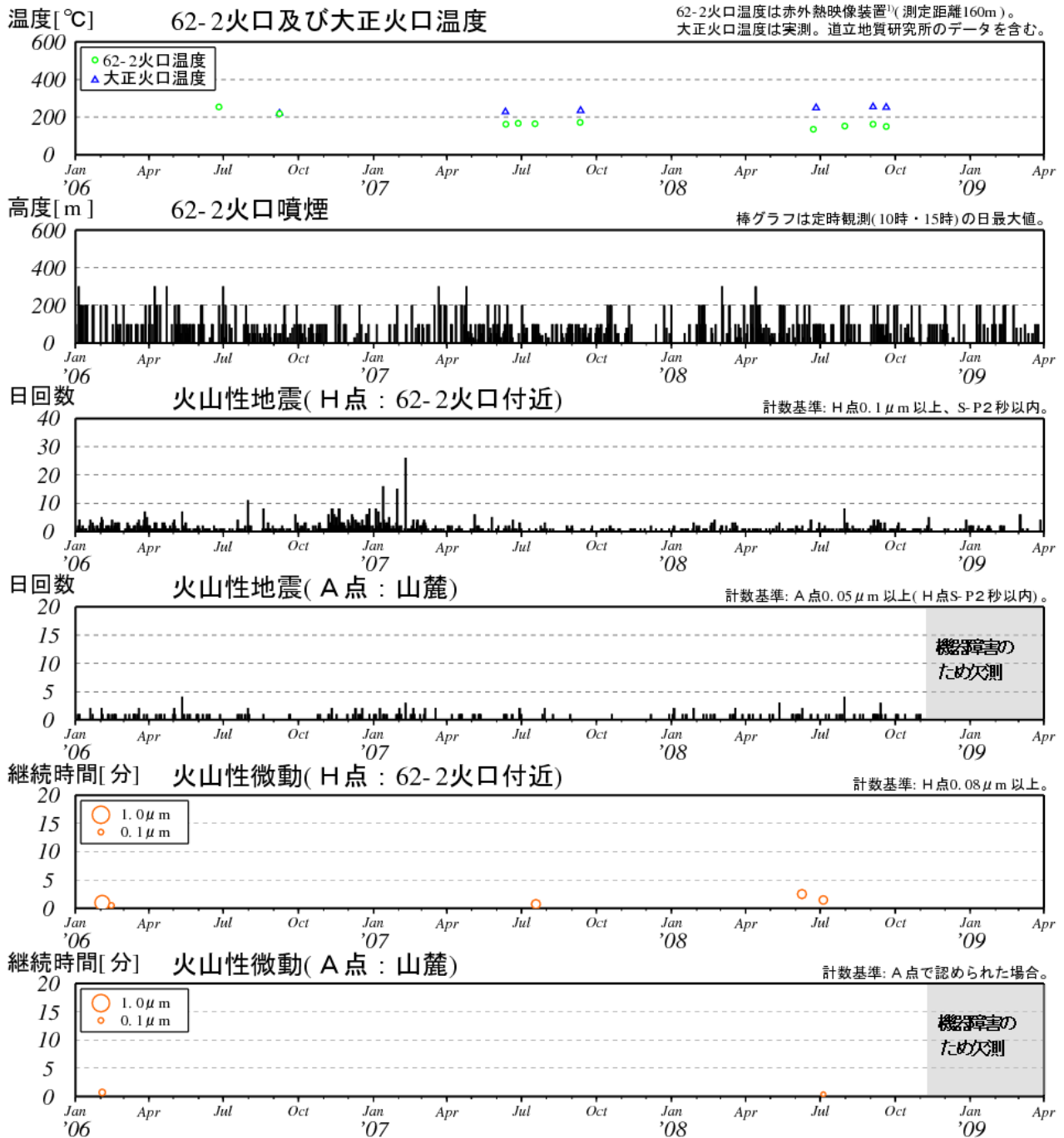
図3※ 十勝岳 最近の火山活動経過図（2006年1月～2009年3月） （A点の地震計は機器障害のため2008年11月7日から欠測しています）
