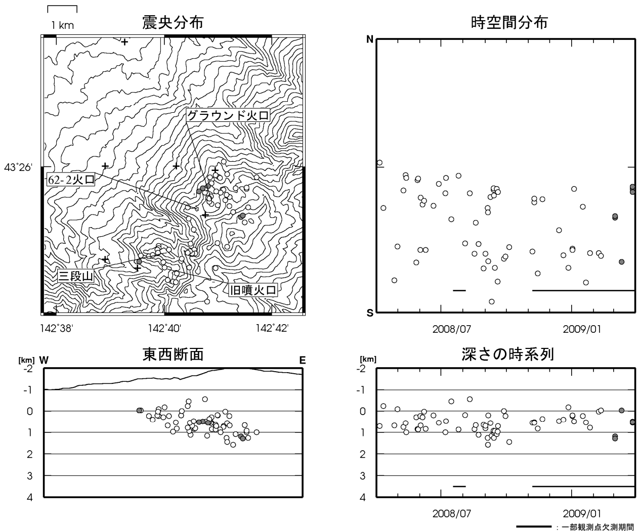
図 4 ※ 十勝岳 震源分布図（2008 年 4 月～2009 年 3 月、+は地震観測点）
