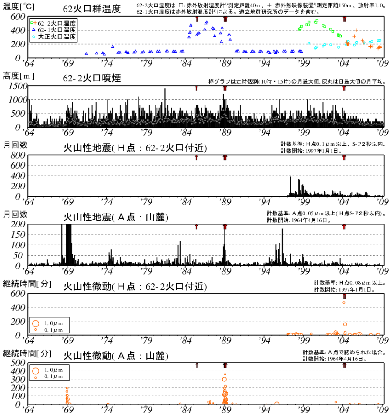
図2※ 十勝岳 長期の火山活動経過図（1964年1月～2009年3月）
