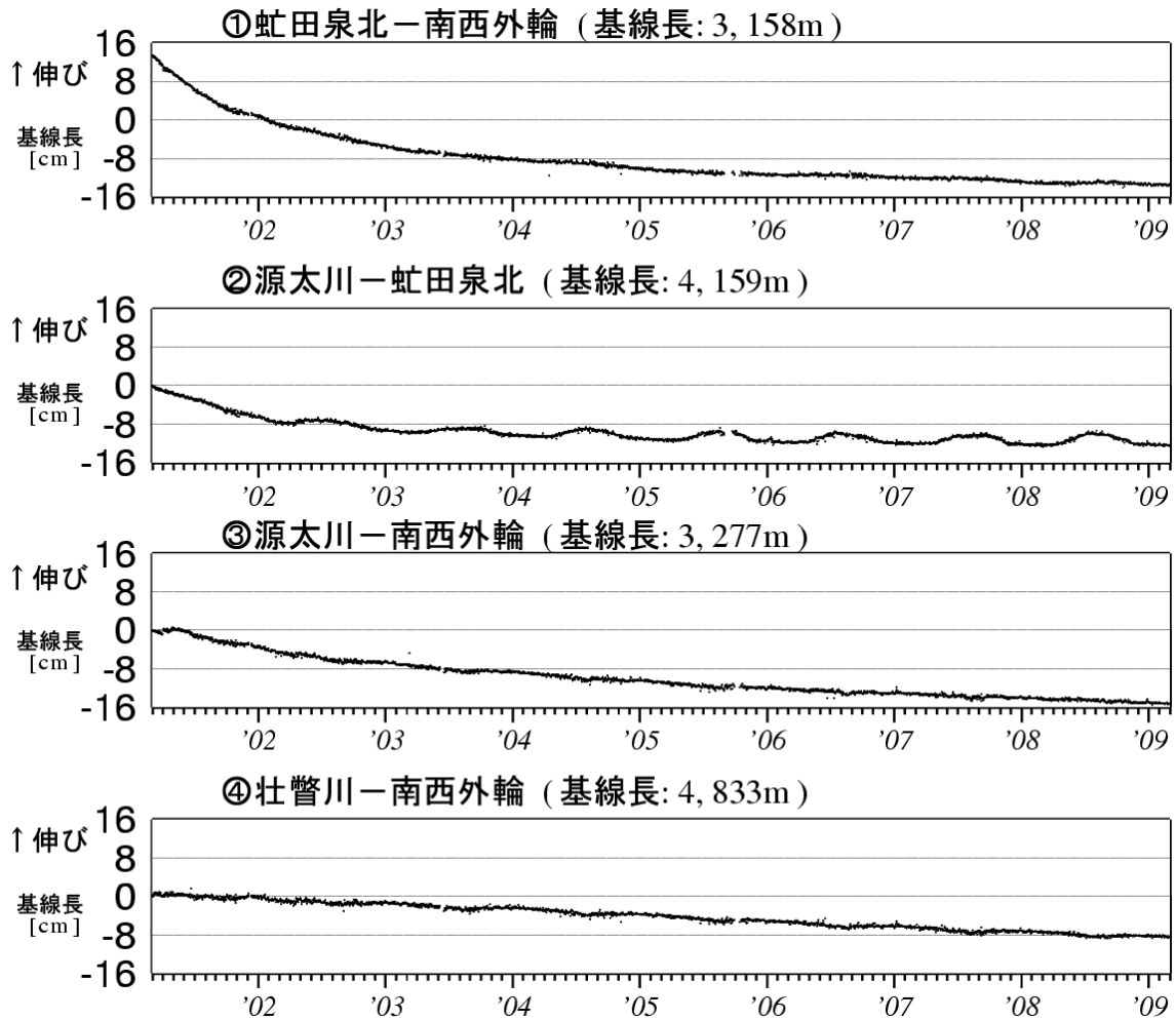
図 5 有珠山 GPS 連続観測による基線長変化（2001 年 3 月～2009 年 2 月） グラフの空白部分は欠測 図 5 の①～④は、図 6 の GPS 基線①～④に対応しています。
