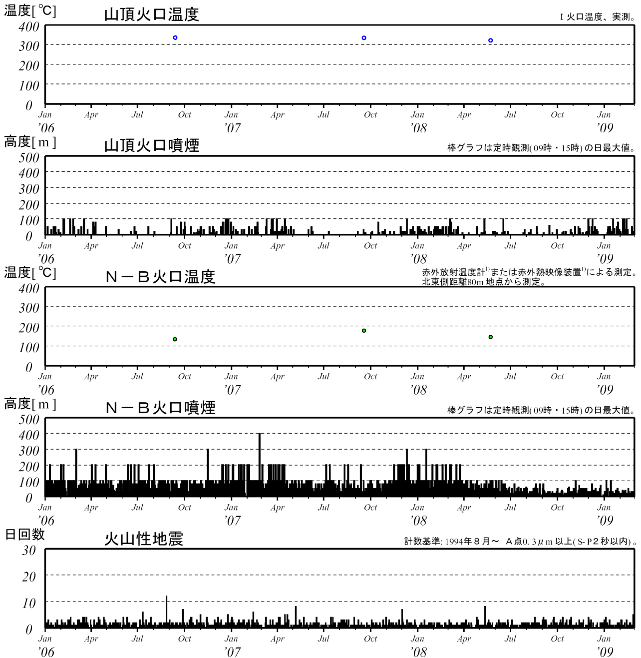
図3 有珠山 最近の火山活動経過図（2006年1月～2009年2月） ・2006年9月以降、地震回数は一日あたり概ね5回以下で推移しています。
