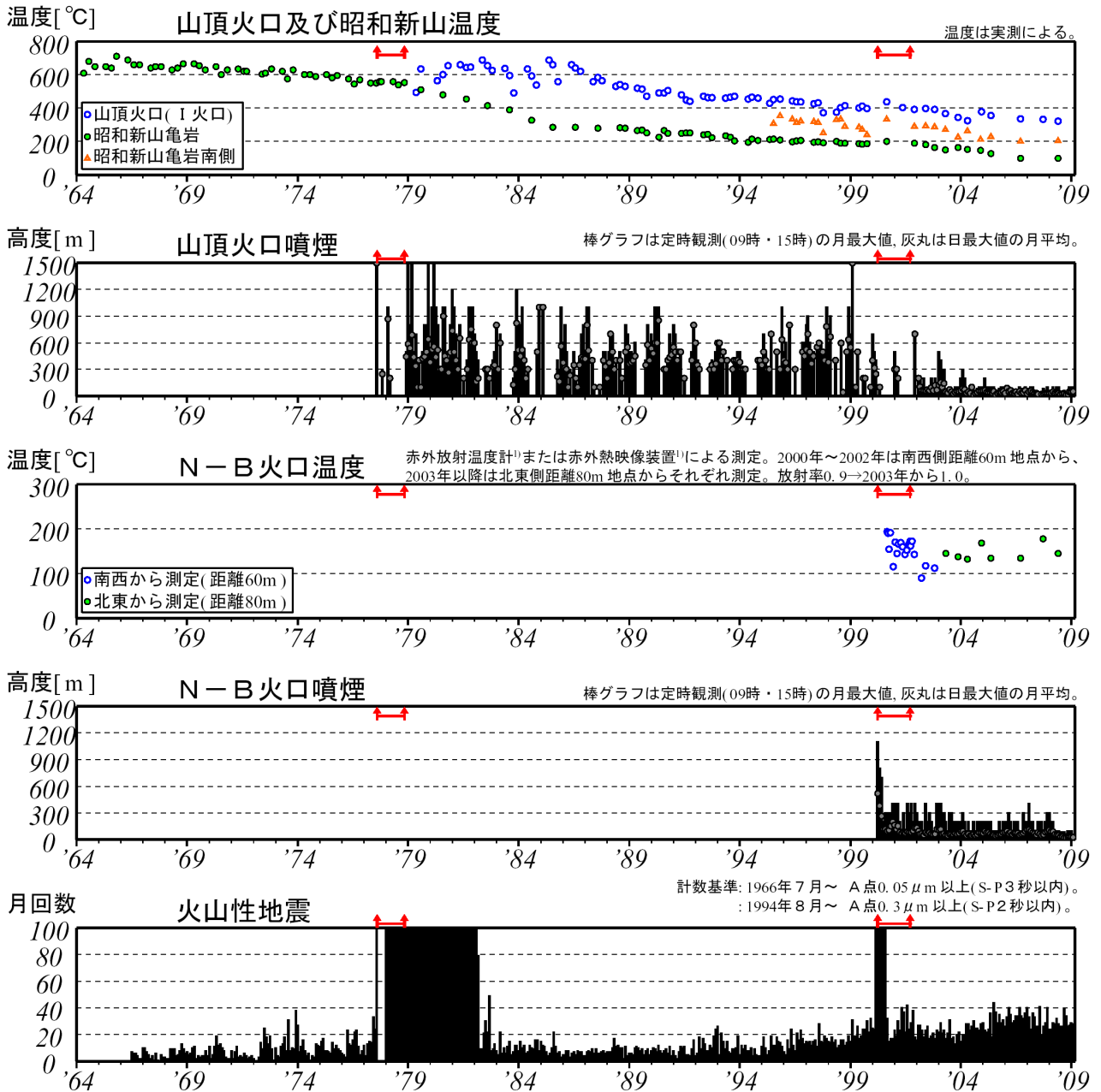
図2 有珠山 長期の火山活動経過図（1964年1月～2009年2月）
