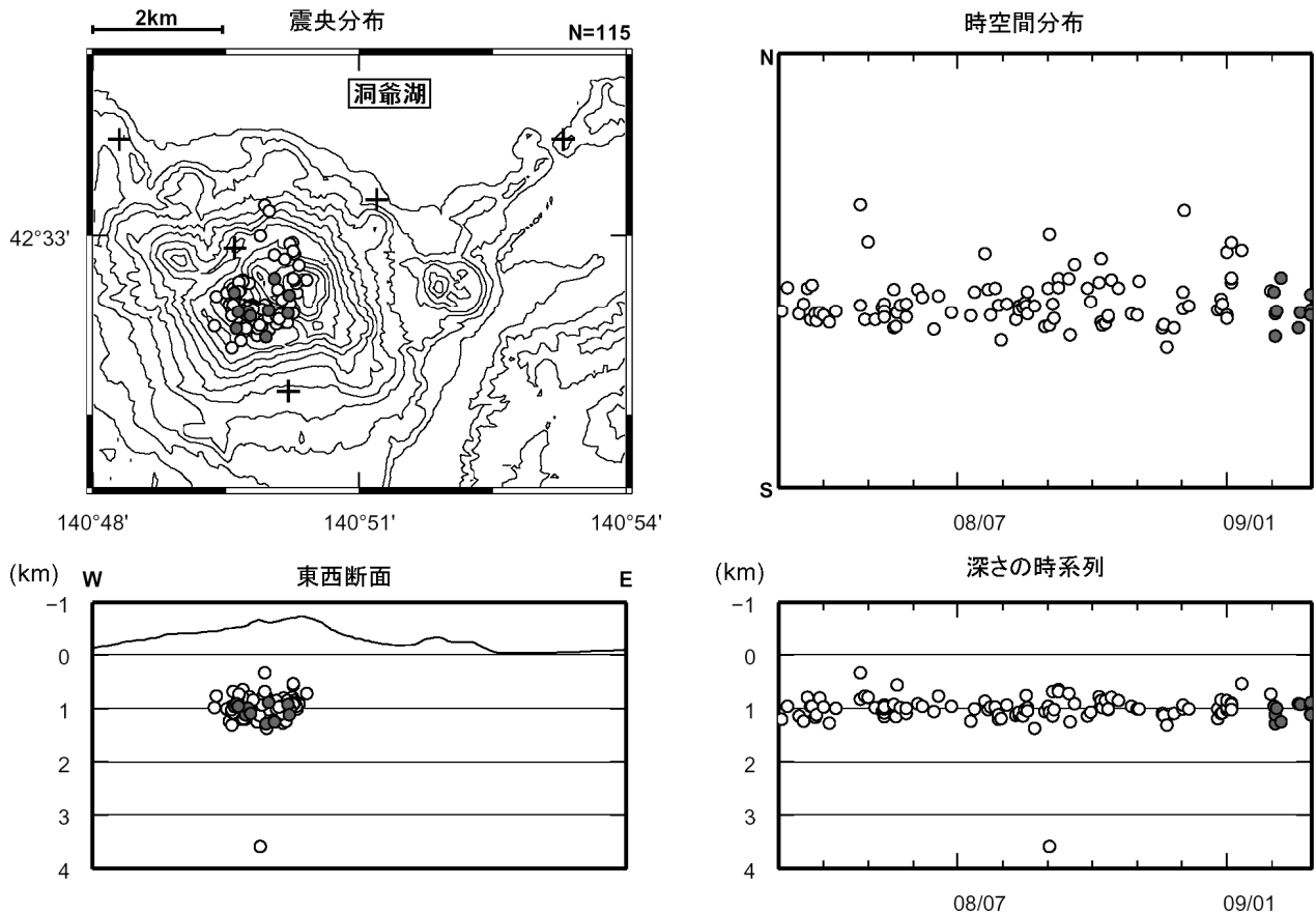
図 4 有珠山 震源分布図（2008 年 3 月～2009 年 2 月、+は地震観測点）
