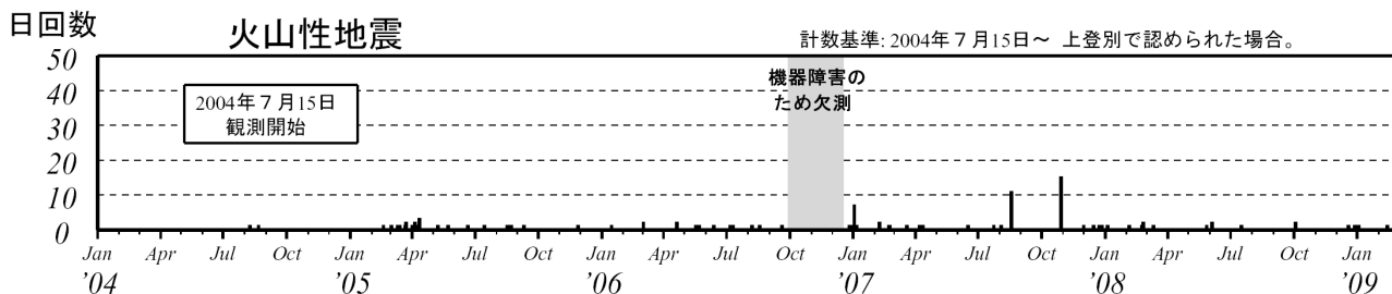
図 2 倶多楽 日別地震回数（2004 年 7 月～2009 年 2 月）
