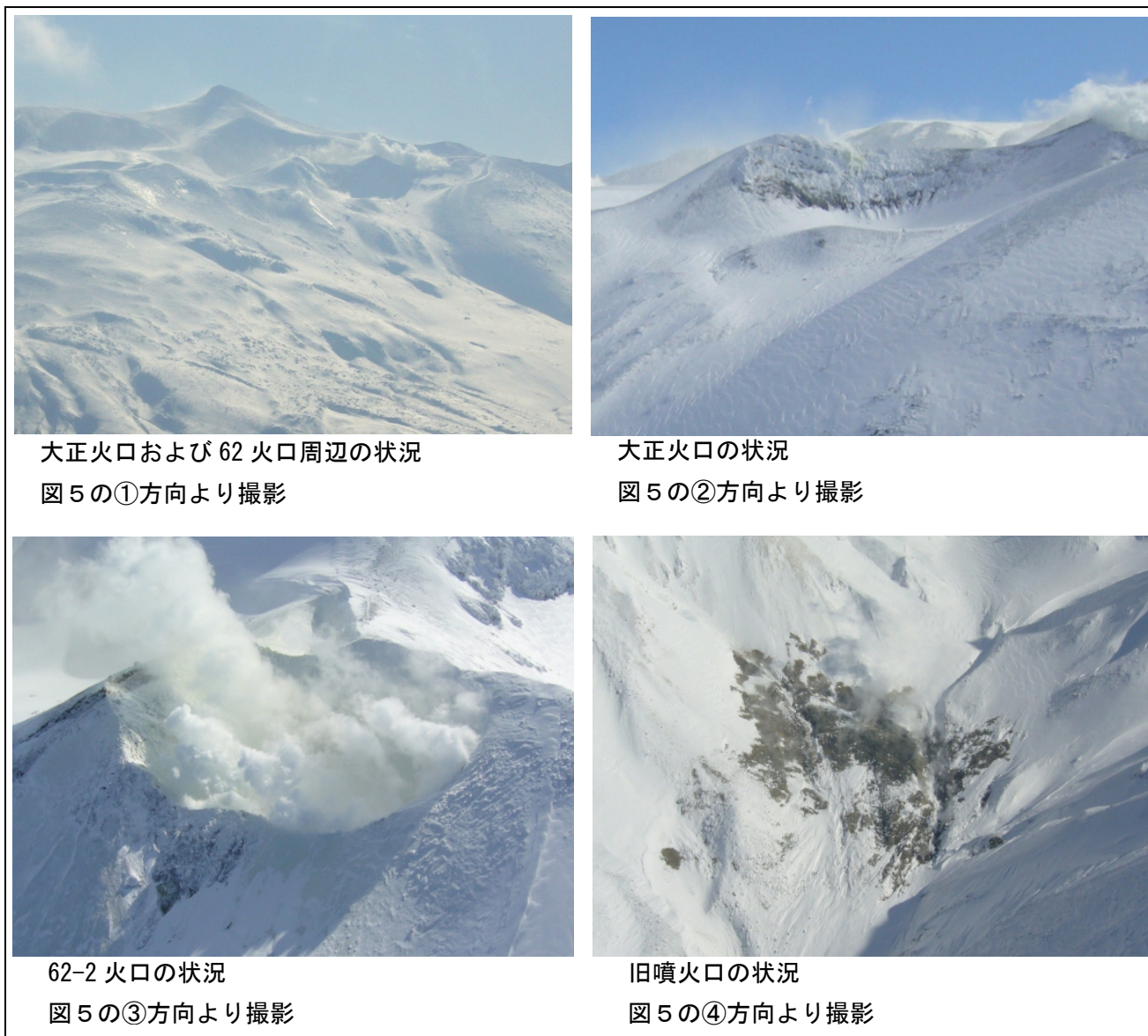
図 4 十勝岳 各火口の状況 (2009 年 2 月 9 日陸上自衛隊第 2 師団の協力により旭川地方気象台が撮影)
