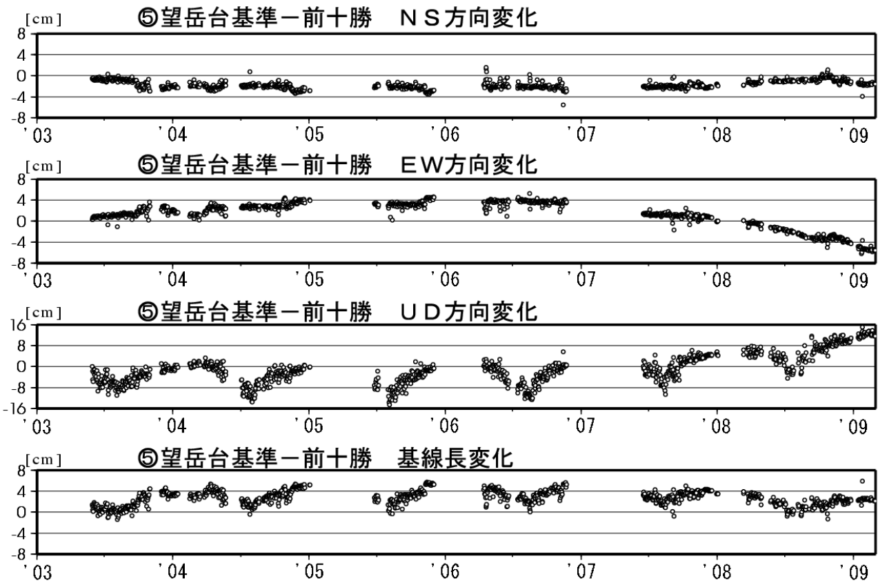
図9※ 十勝岳 GPS 連続観測による成分変化 (2003 年 5 月～2009 年 2 月)
