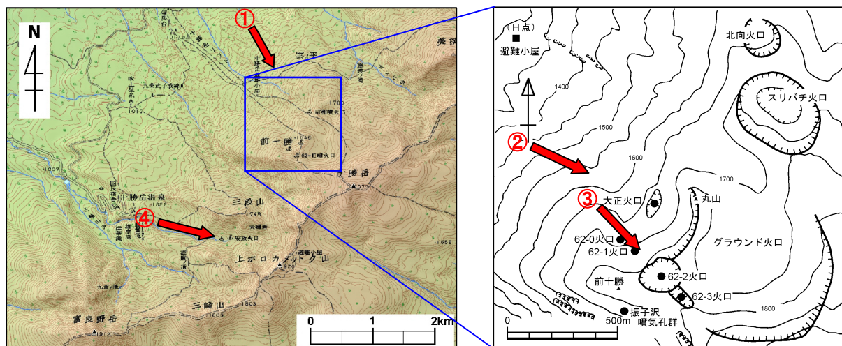
図 5 十勝岳 火口周辺図
