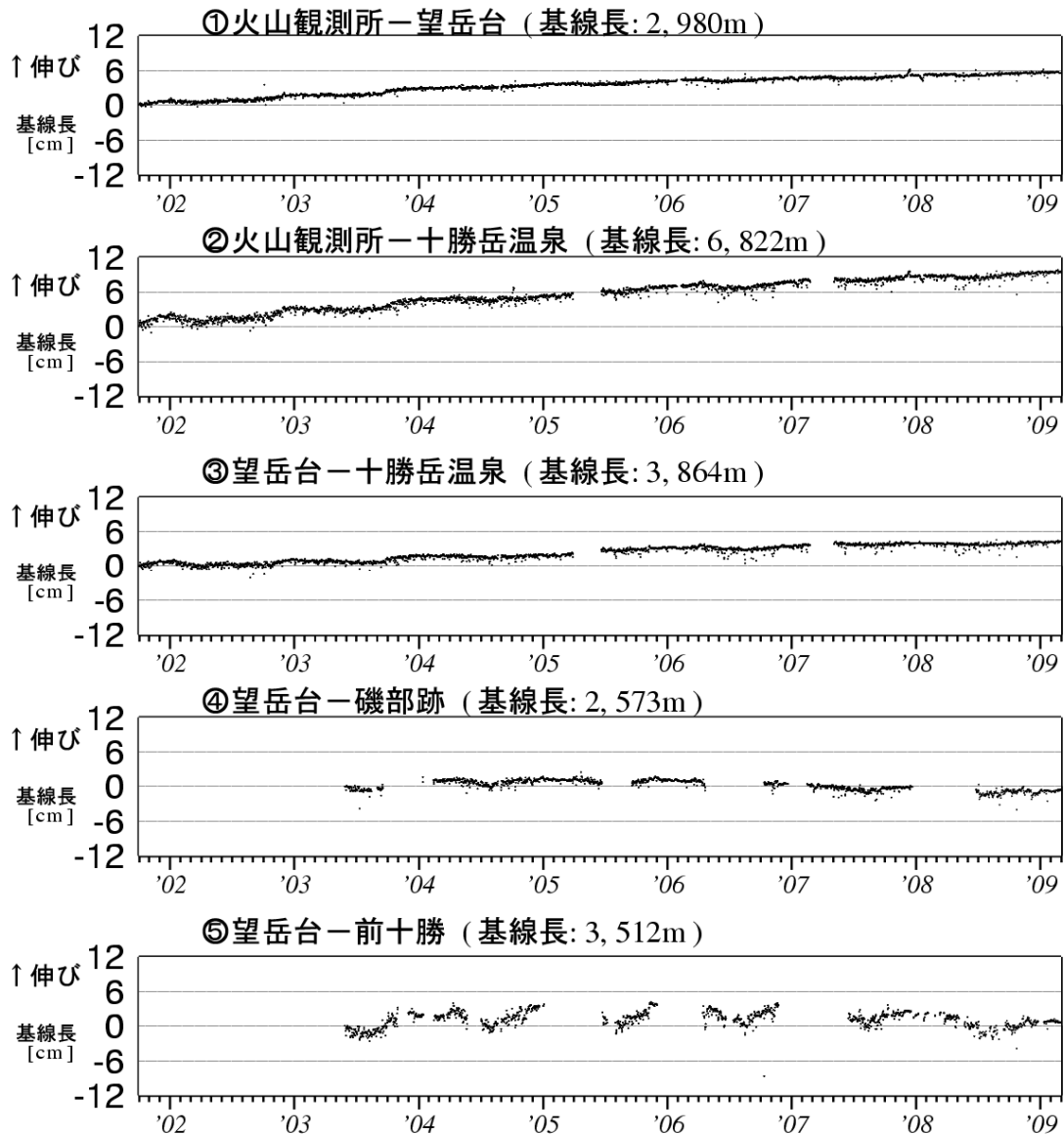
図 7※ 十勝岳 GPS 連続観測による基線長変化 (2001 年 10 月～2009 年 2 月) グラフの空白部分は欠測。
