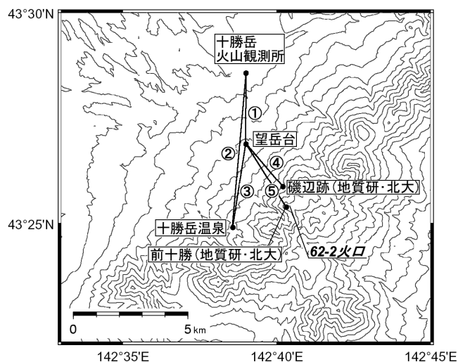
図 8※ 十勝岳 GPS 観測点配置図
