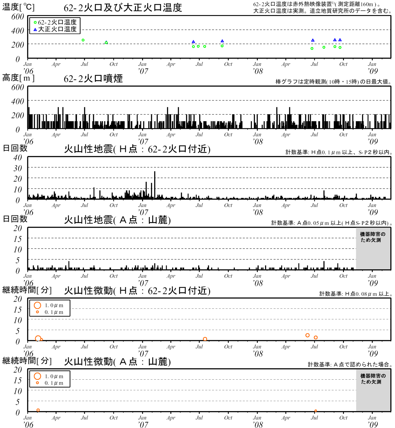
図3※ 十勝岳 最近の火山活動経過図 (2006年1月～2009年2月) (A点の地震計は機器障害のため2008年11月7日から欠測しています)
