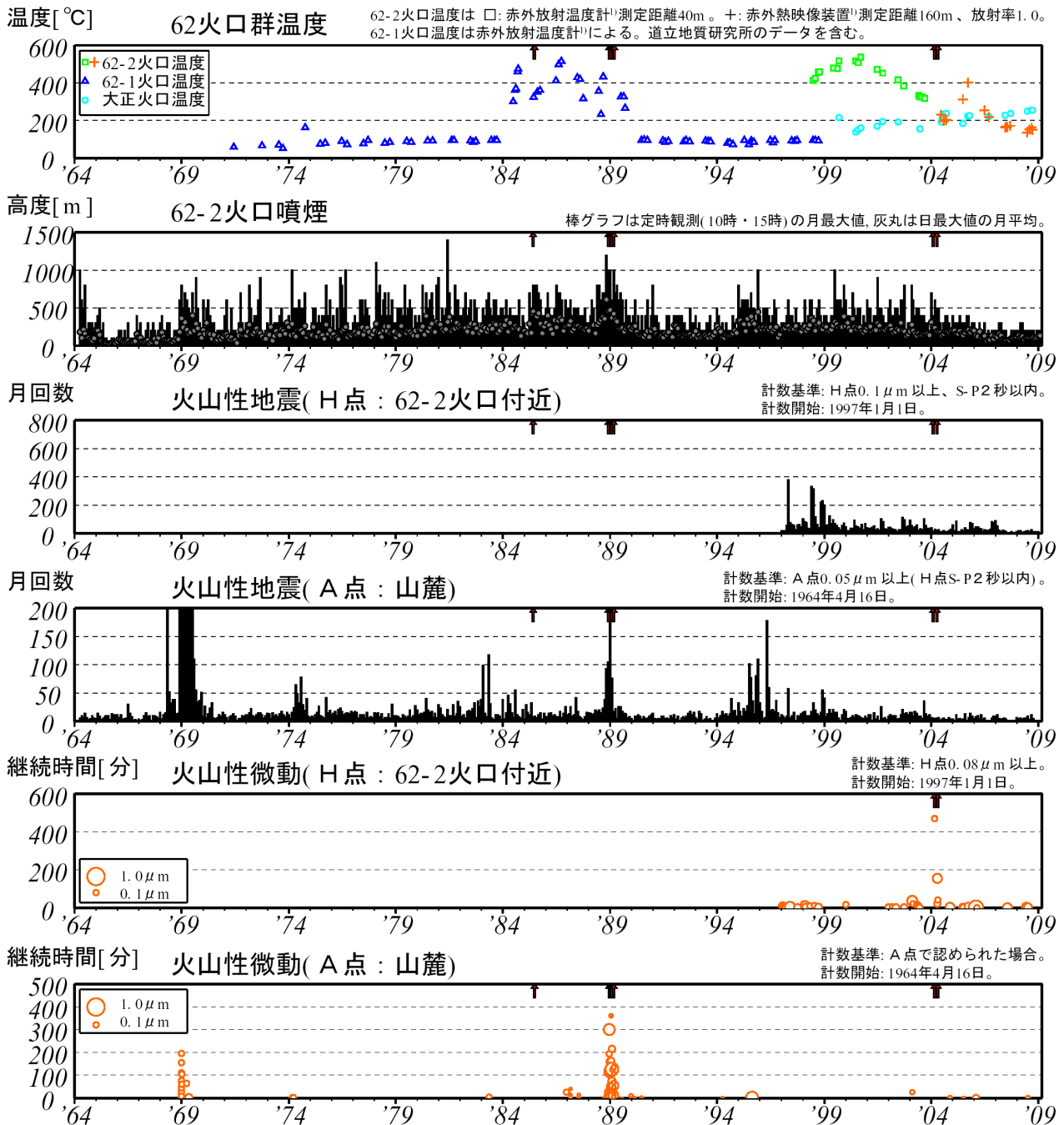
図 2 ※ 十勝岳 長期の火山活動経過図 (1964 年 1 月～2009 年 2 月)
