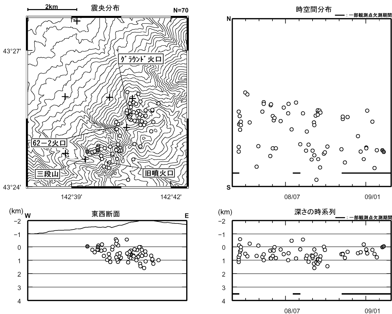
図 6※ 十勝岳 震源分布図 (2008 年 3 月～2009 年 2 月、+は地震観測点)
