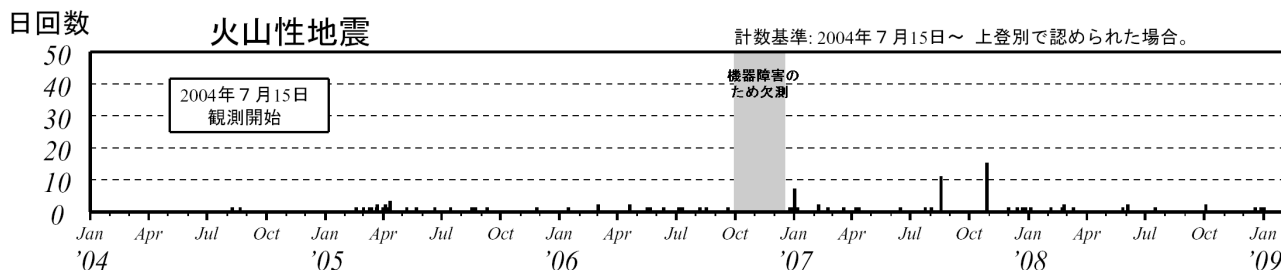
図 2 倶多楽 日別地震回数（2004 年 7 月～2009 年 1 月）
