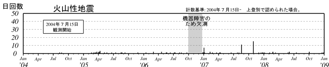
図 2 倶多楽 日別地震回数（2004 年 7 月～2008 年 12 月）
