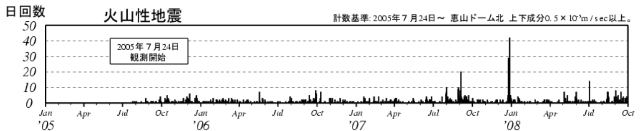
図 1 恵山 日別地震回数（2005 年 7 月～2008 年 9 月）
