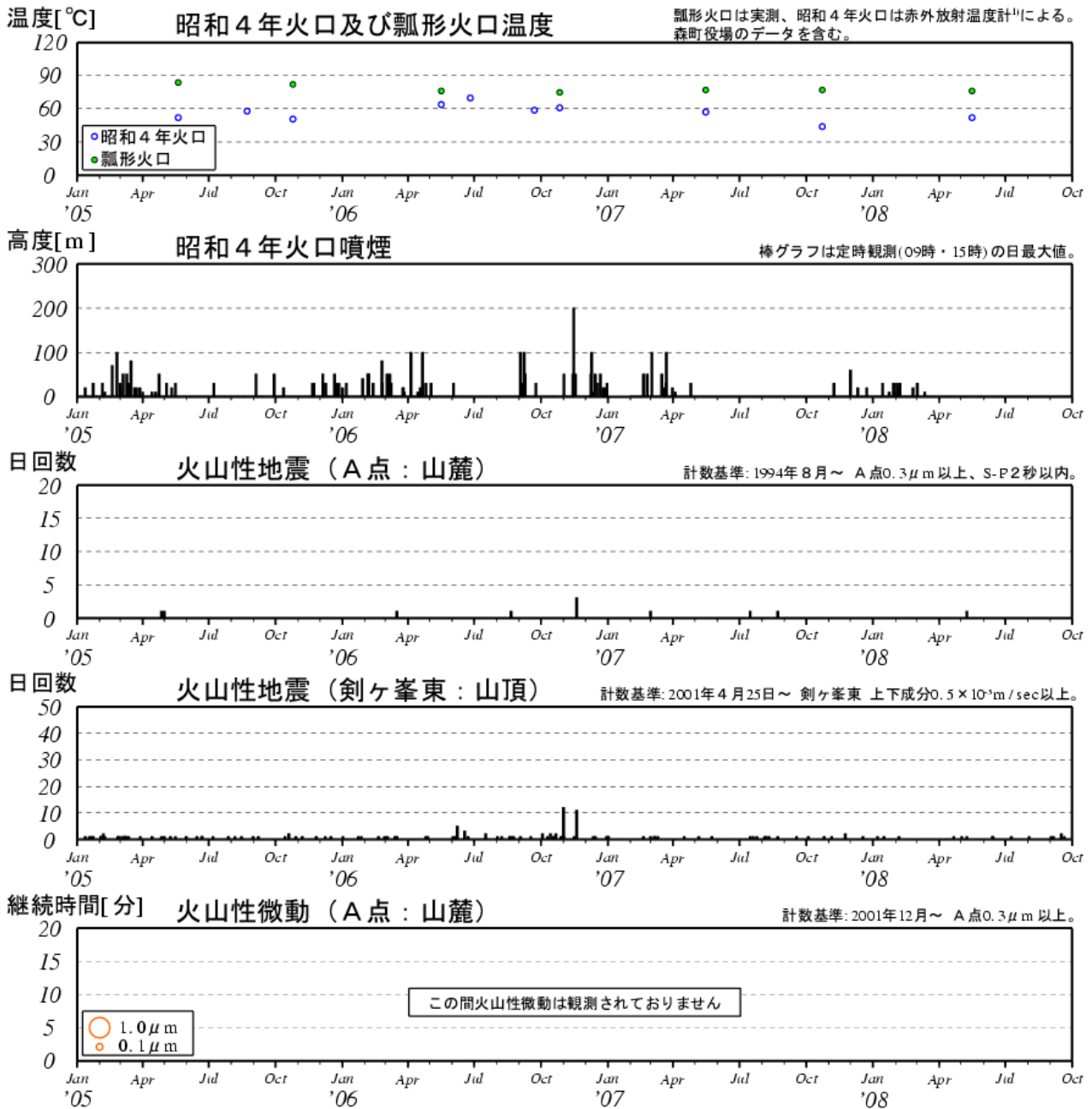
図3※ 北海道駒ヶ岳 最近の火山活動経過図（2005年1月～2008年9月）
