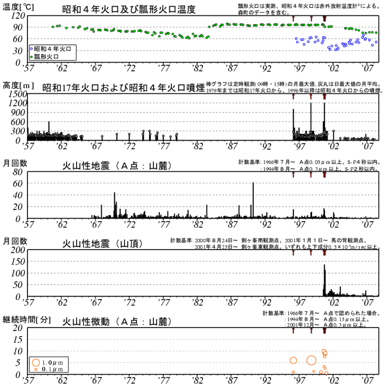
図 2※ 北海道駒ヶ岳 長期の火山活動経過図（1957 年 1 月～2008 年 9 月）↑印は噴火
