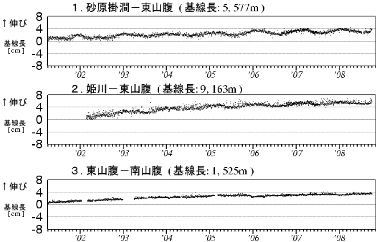
図5 北海道駒ヶ岳 GPS 連続観測による基線長変化（2001年4月～2008年9月） グラフの空白部分は欠測 ・図5の1～3は、図6のGPS基線①～③に対応しています。
